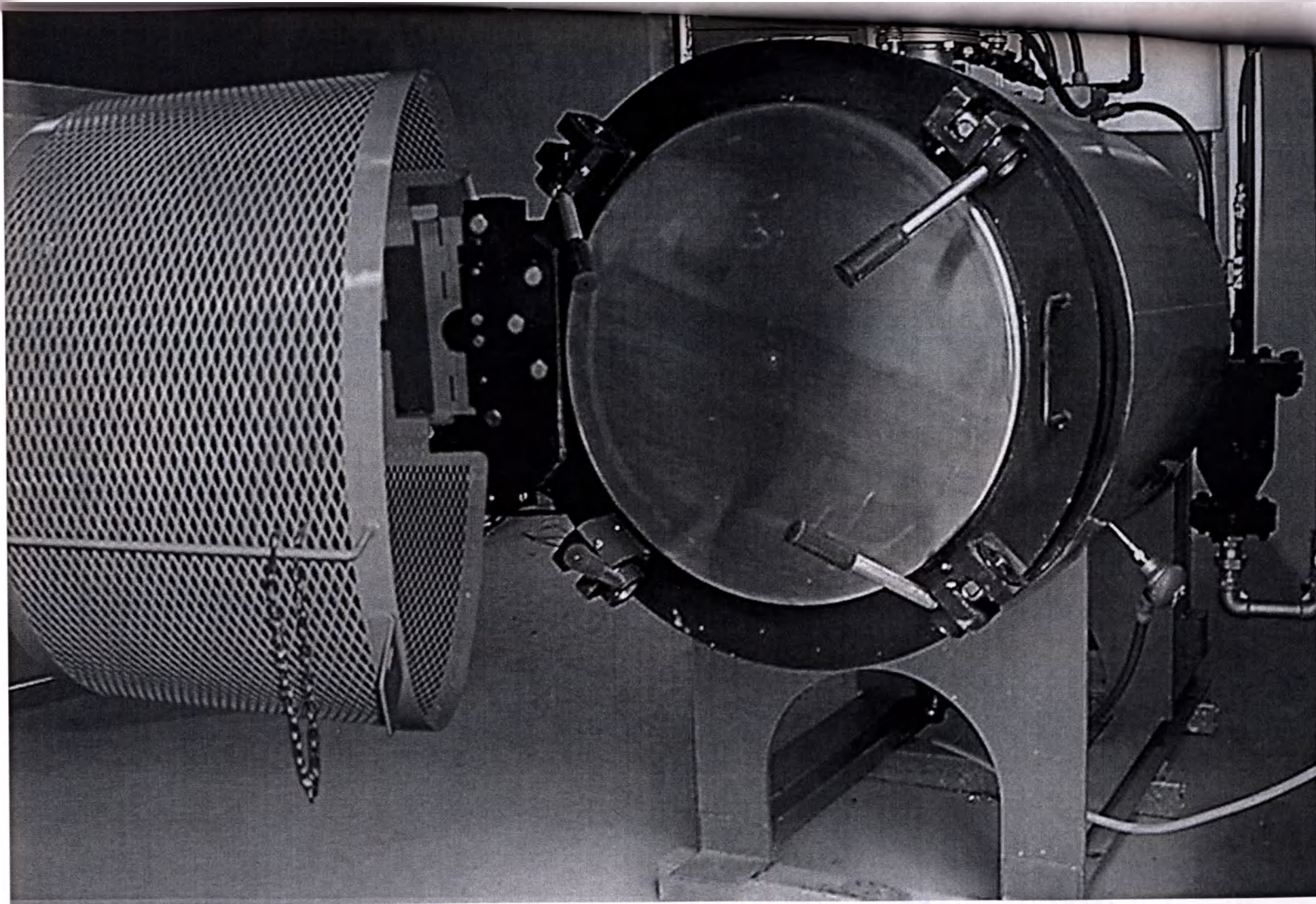
Рис. 4 Установка для обезвреживания и утилизации медицинских отходов «Гидроклав Р-440Б»
