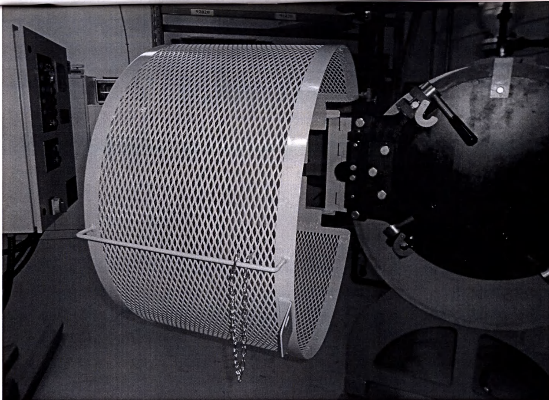
Рис. 2 Установка для обезвреживания и утилизации медицинских отходов «Гидроклав Р-230»
