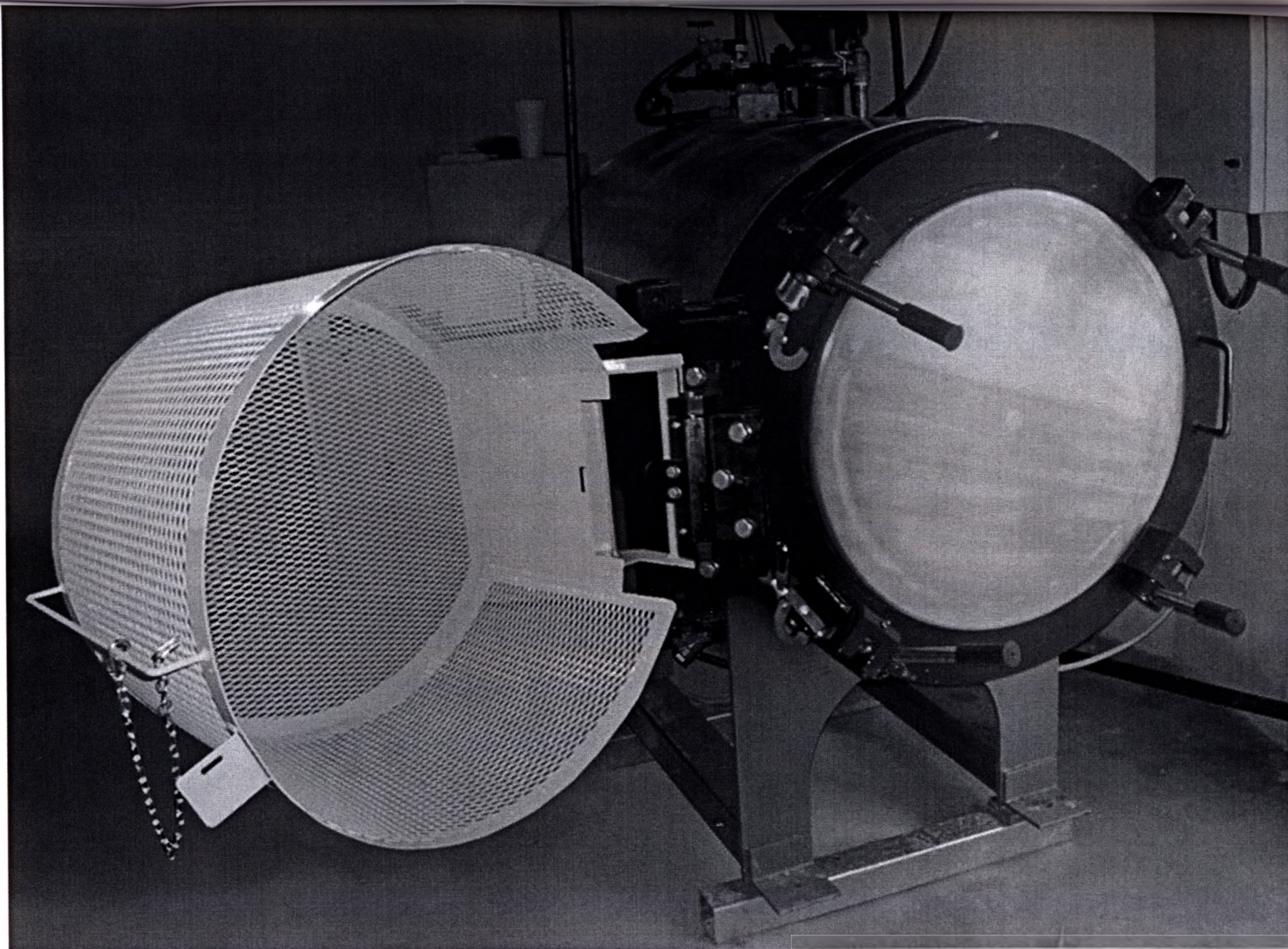
Рис. 3 Установка для обезвреживания и утилизации медицинских отходов «Гидроклав Р-440»
