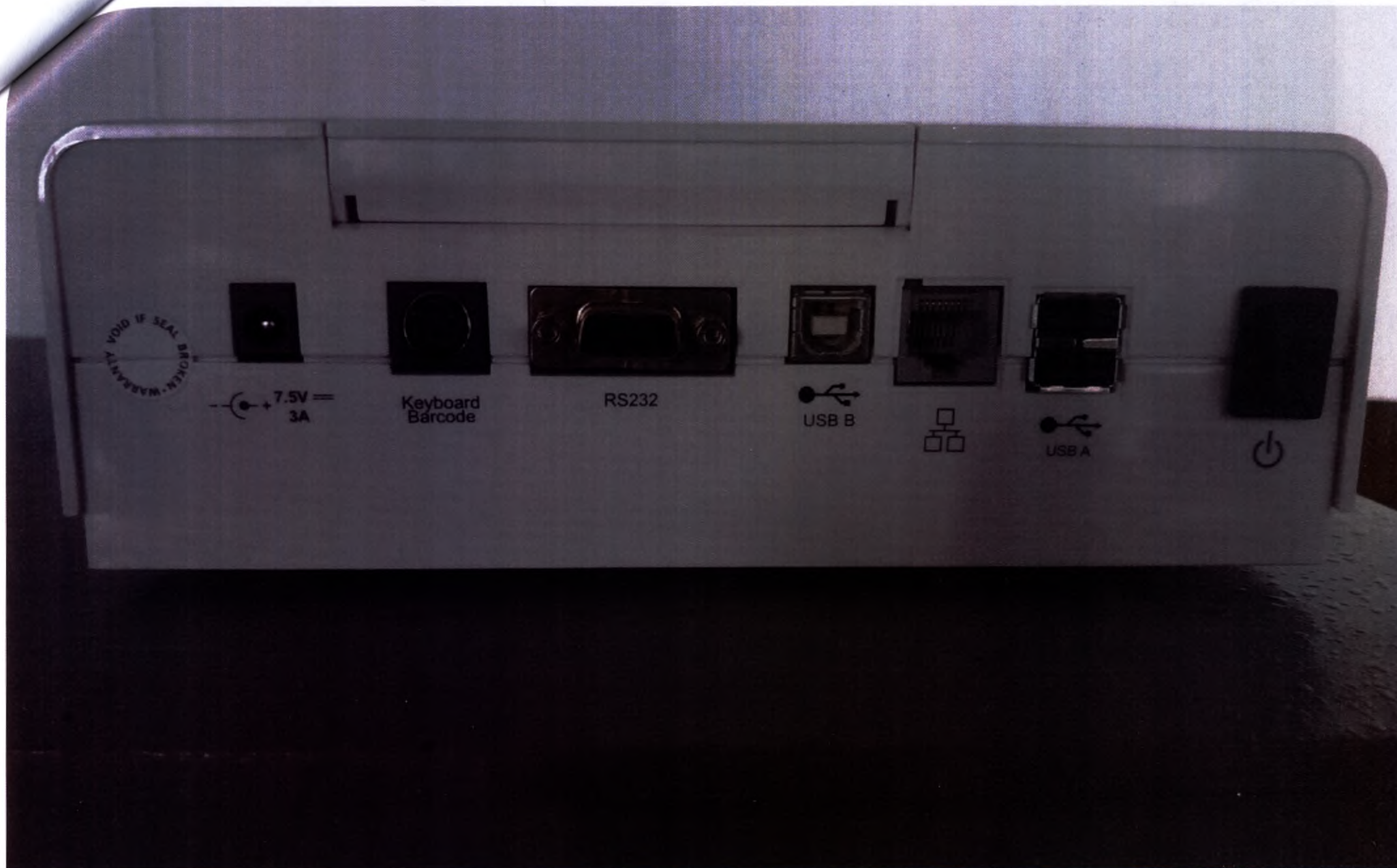
Анализатор мочи лабораторный Urilyzer 100 pro
