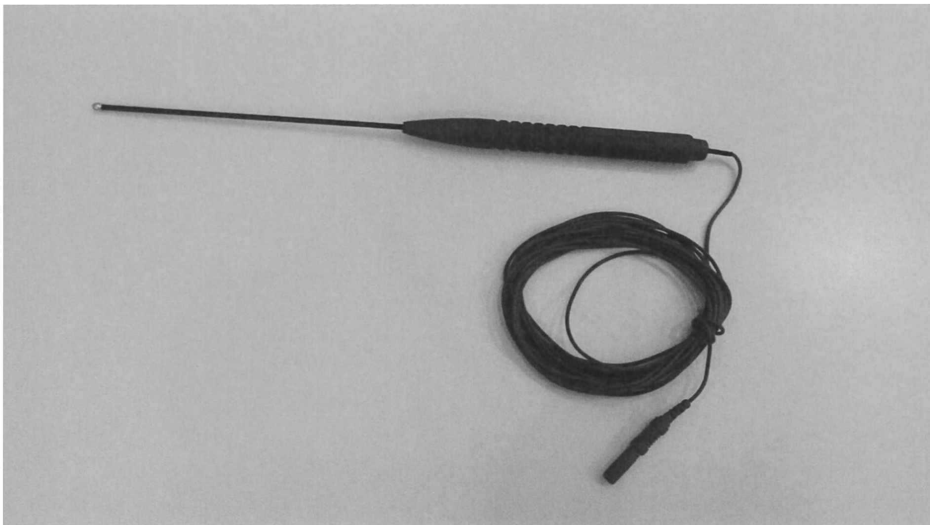
Электрод-зонд стимулирующий монополярный сферический с длиной стержня 100мм, артикул SI1B0100S2526DRU
