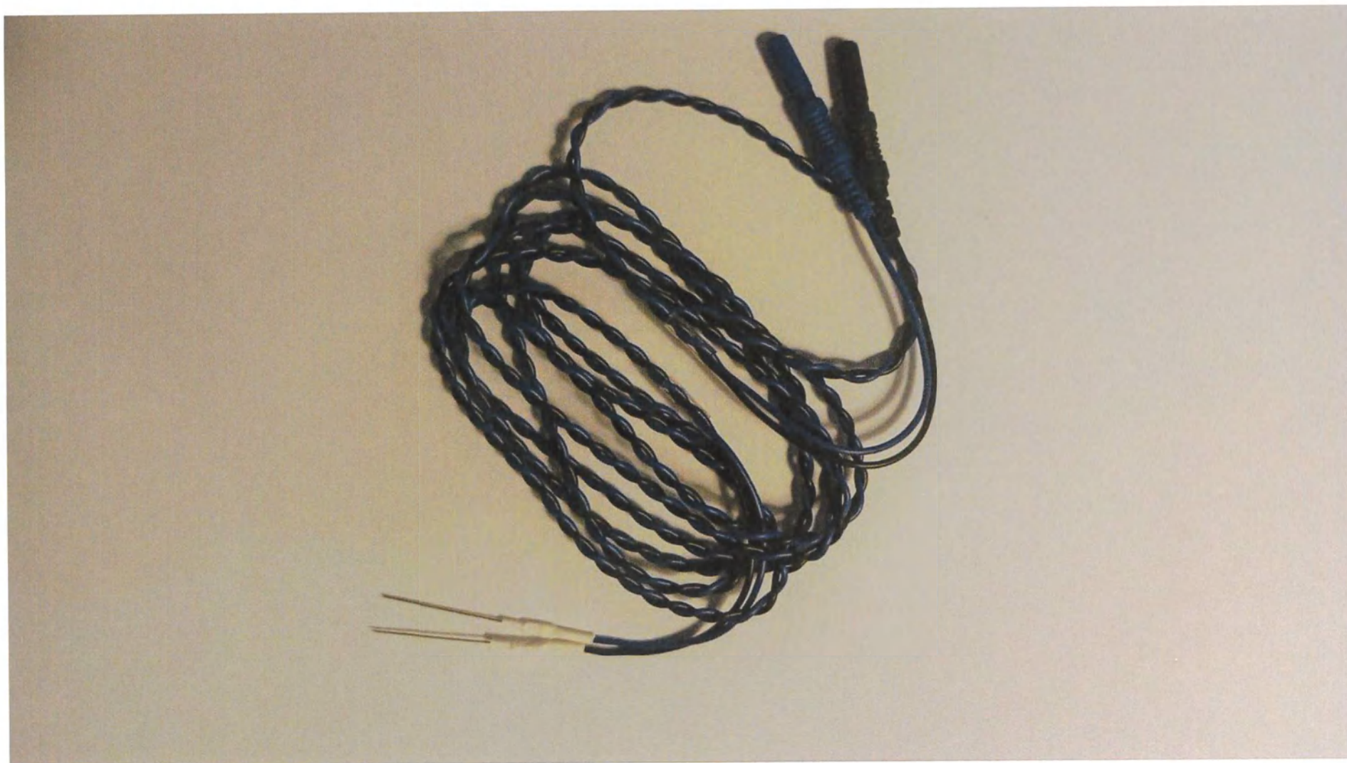
Электрод игольчатый подкожный скрученный с длиной иглы 22 мм, диаметром иглы 0.40 мм, с кабелем длиной 150 см, артикул MN4022D15A/SRU
