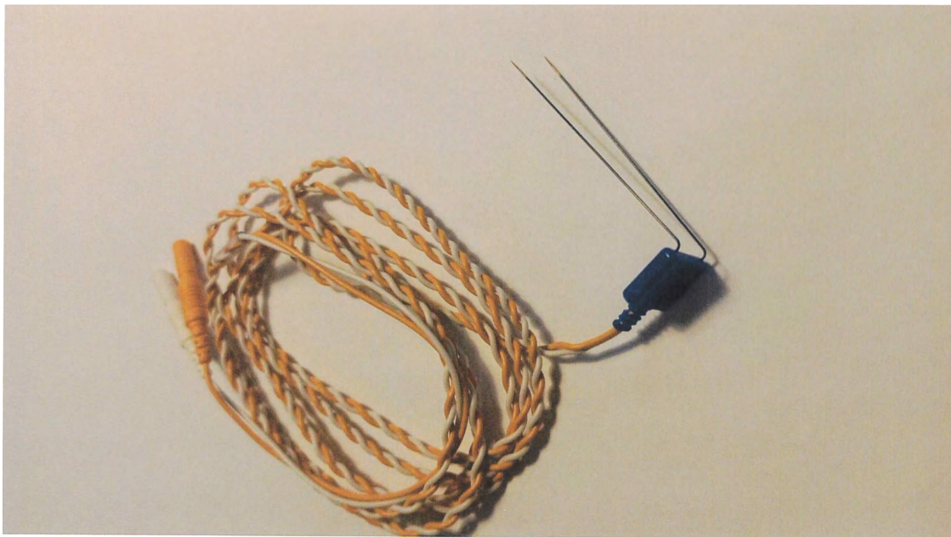
Электрод игольчатый парный скрученный с длиной иглы 50 мм, диаметром иглы 0.45 мм с углом наклона иглы 90° и расстоянием между иглами 10 мм, с кабелем длиной 150 см, артикул TFDN455041RU
