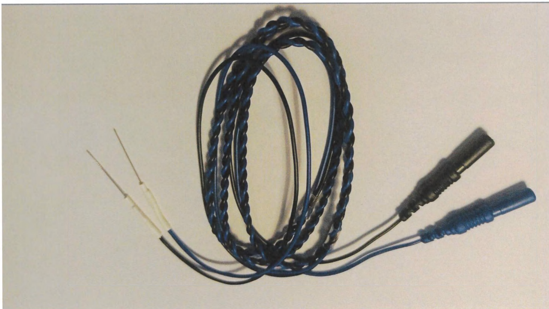
Электрод игольчатый подкожный скрученный с длиной иглы 18 мм, диаметром иглы 0.40 мм, с кабелем длиной 100 см, артикул MN4018D10A/SRU
