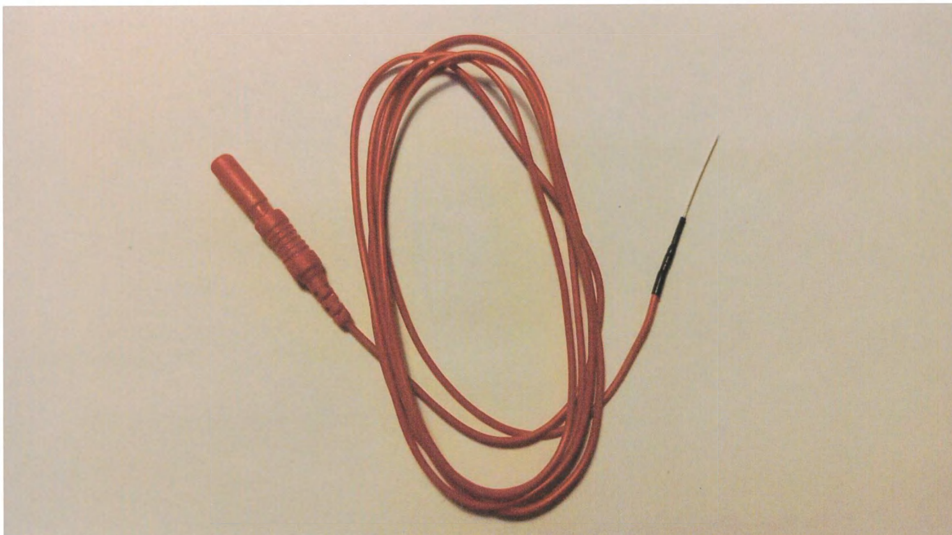
Электрод игольчатый подкожный с длиной иглы 18 мм, диаметром иглы 0.40 мм, с кабелем длиной 100 см, артикул MN4018D10SRU
