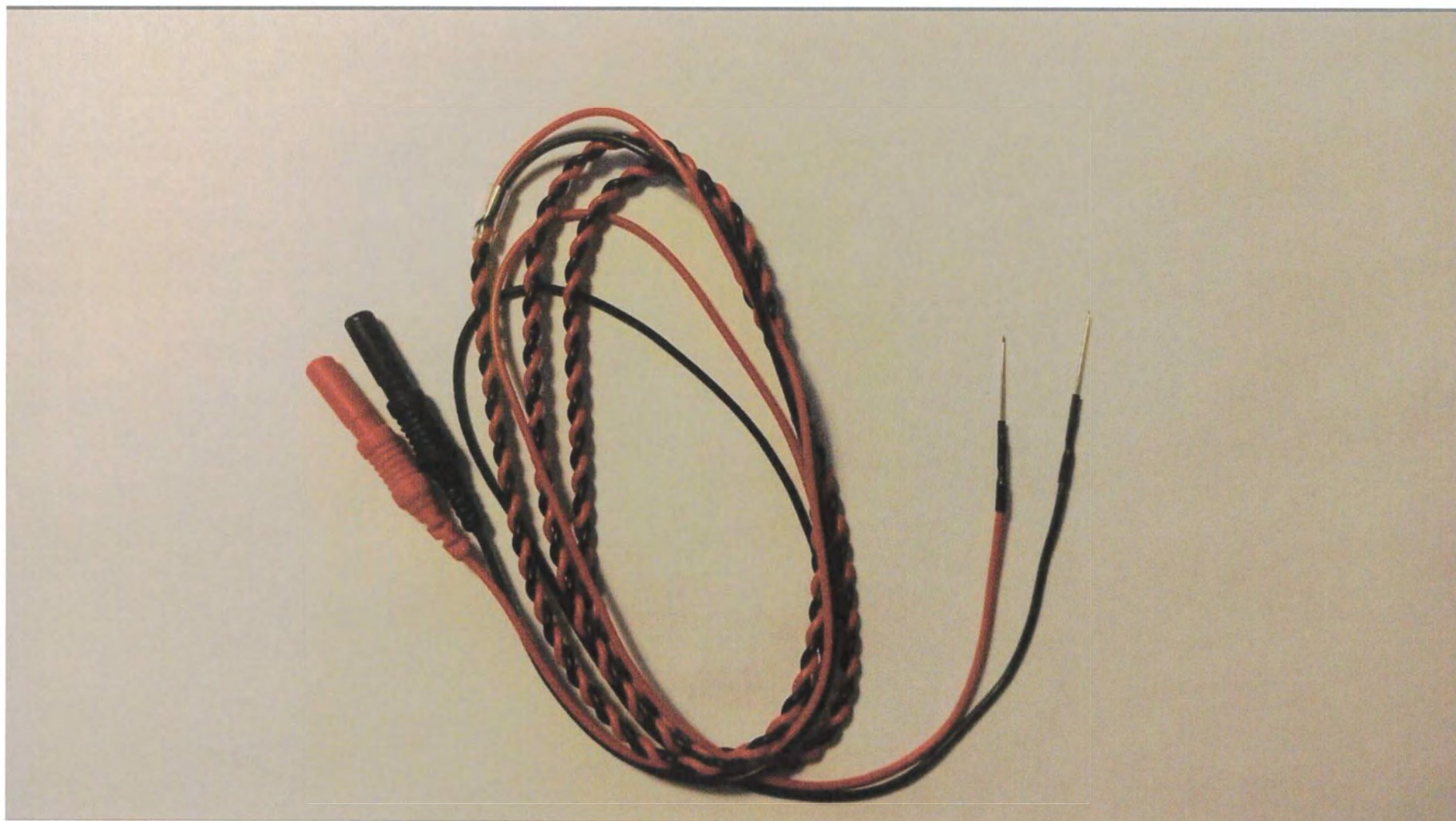
Электрод игольчатый подкожный скрученный с длиной иглы 13 мм, диаметром иглы 0.40 мм, с кабелем длиной 100 см, артикул MN4013D10A/SRU
