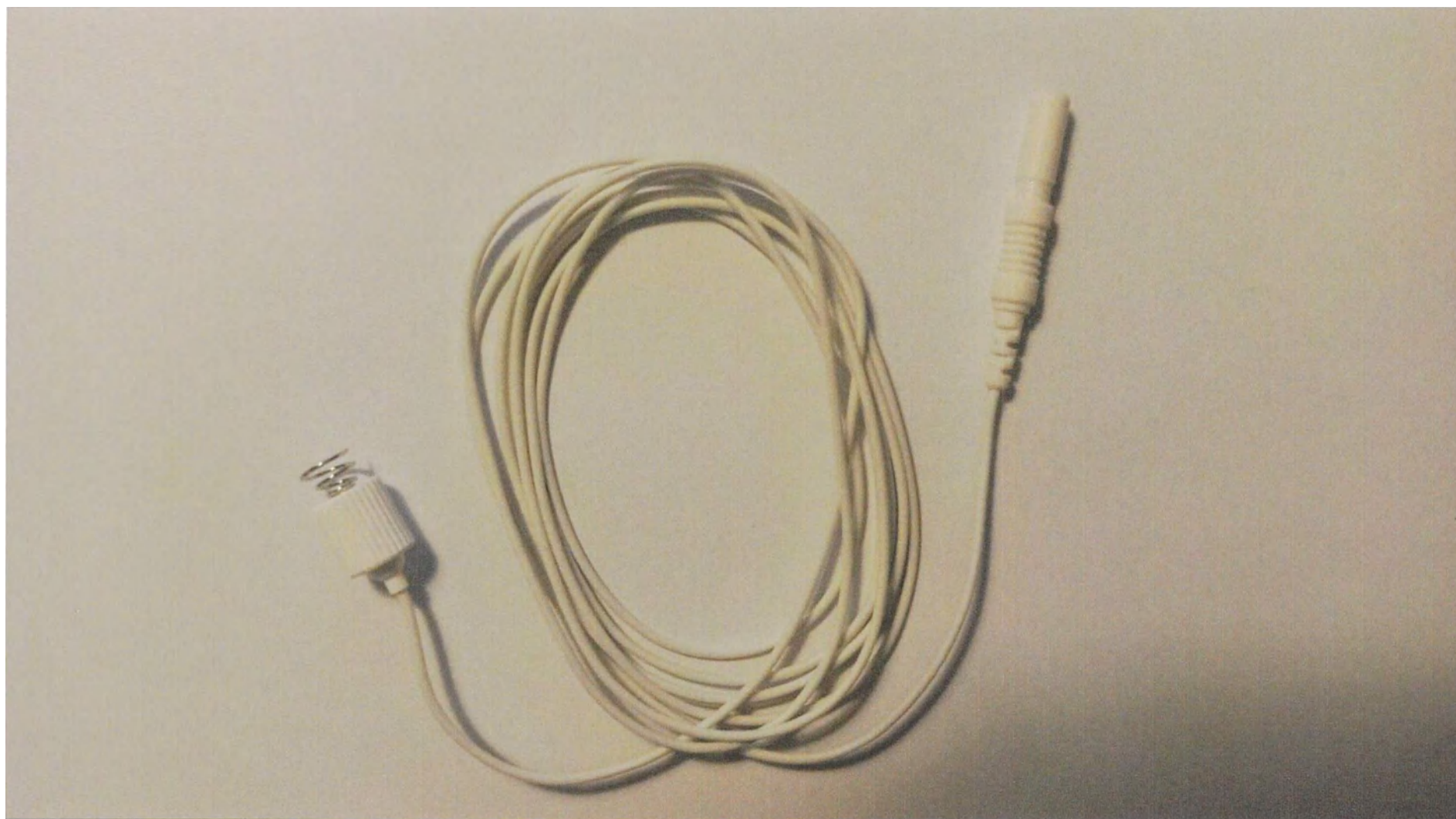
Электрод игольчатый штупорный, без экрана, с длиной иглы 5 мм, диаметром иглы 0.60 мм, с кабелем длиной 150 см, артикул MNCS0615DSRU
