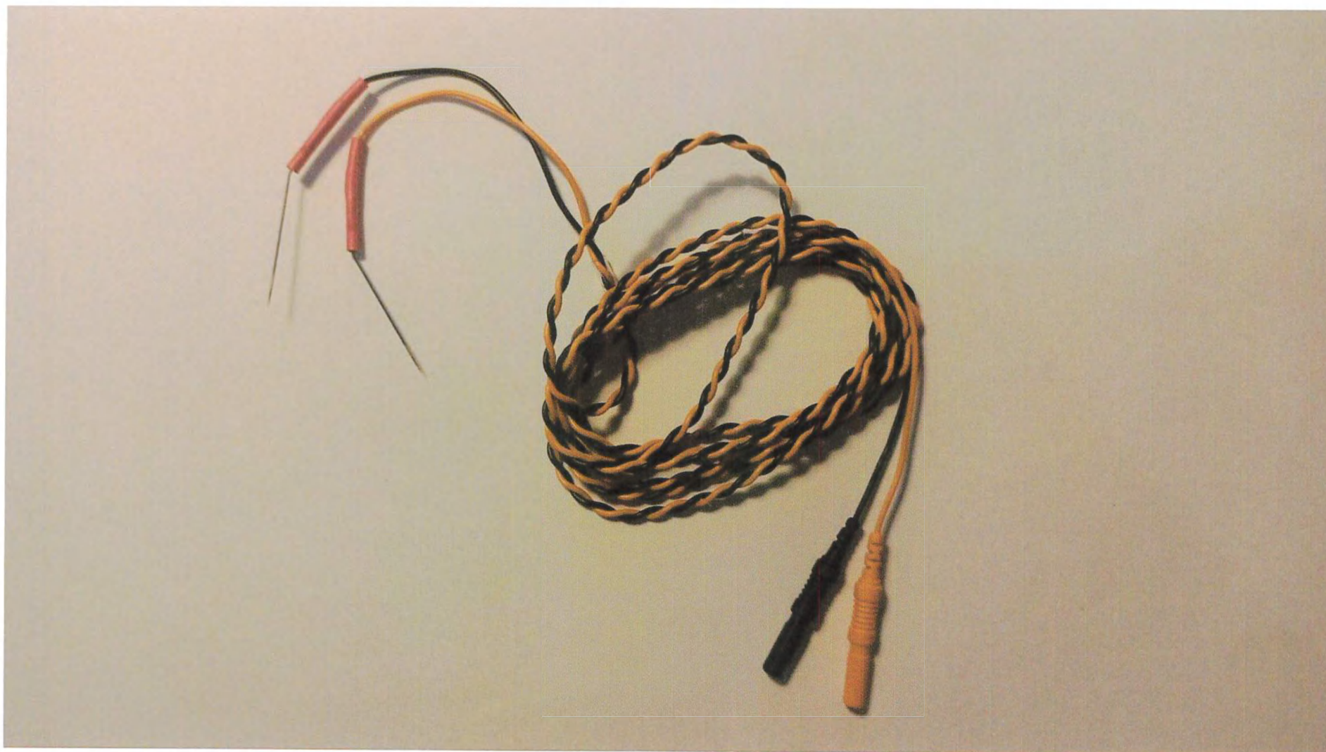
Электрод игольчатый парный скрученный с длиной иглы 25 мм, диаметром иглы 0.45 мм с углом наклона иглы 30° с кабелем длиной 150 см, артикул TFDN452531SBRU
