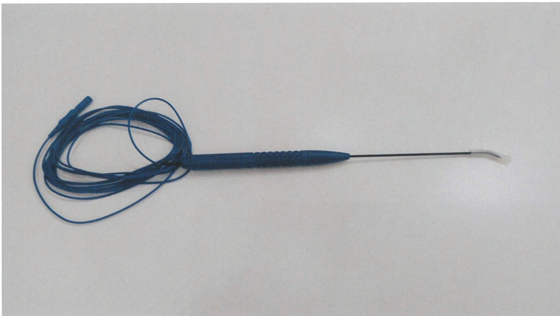
Электрод-зонд стимулирующий монополярный изогнутый с длиной стержня 130/8 мм, артикул SI1IC130S2526DRU
