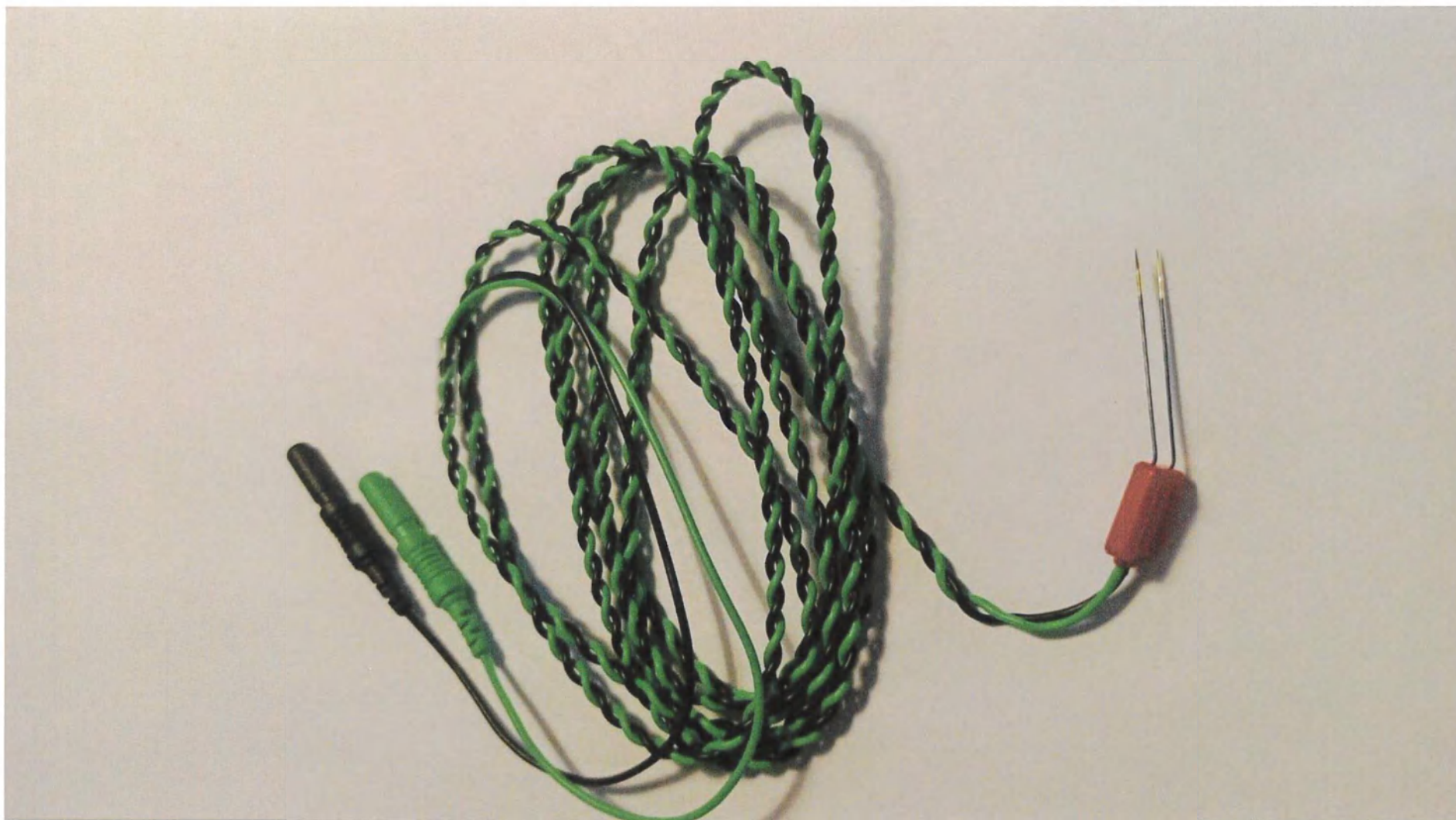
Электрод игольчатый парный скрученный с длиной иглы 25 мм, диаметром иглы 0.45 мм с углом наклона иглы 30° (150°) и расстоянием между иглами 5 мм, с кабелем длиной 150 см, артикул TFDN452531RU
