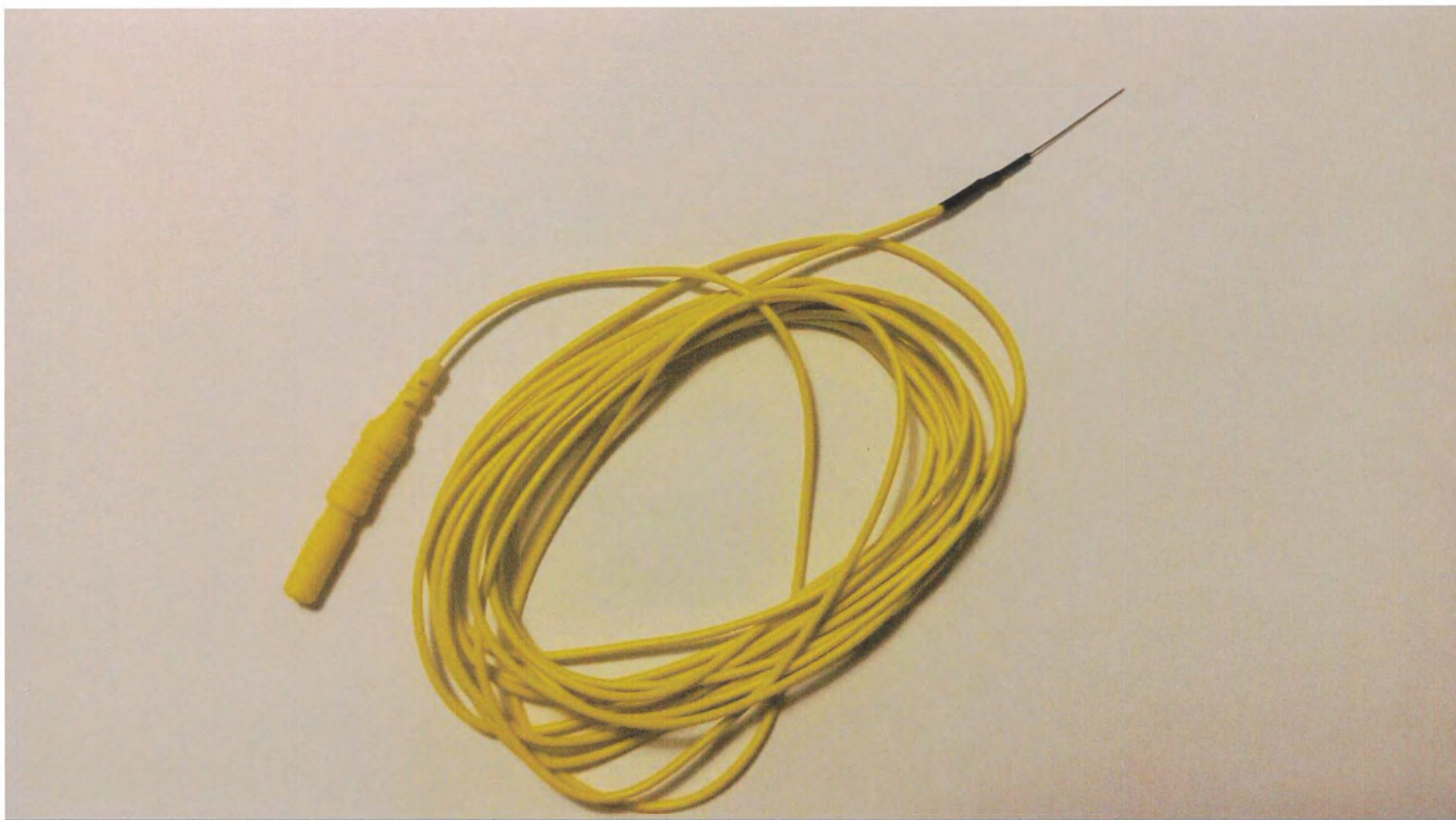
Электрод игольчатый подкожный с длиной иглы 18 мм, диаметром иглы 0.40 мм, с кабелем длиной 250 см, артикул MN4018D25SRU
