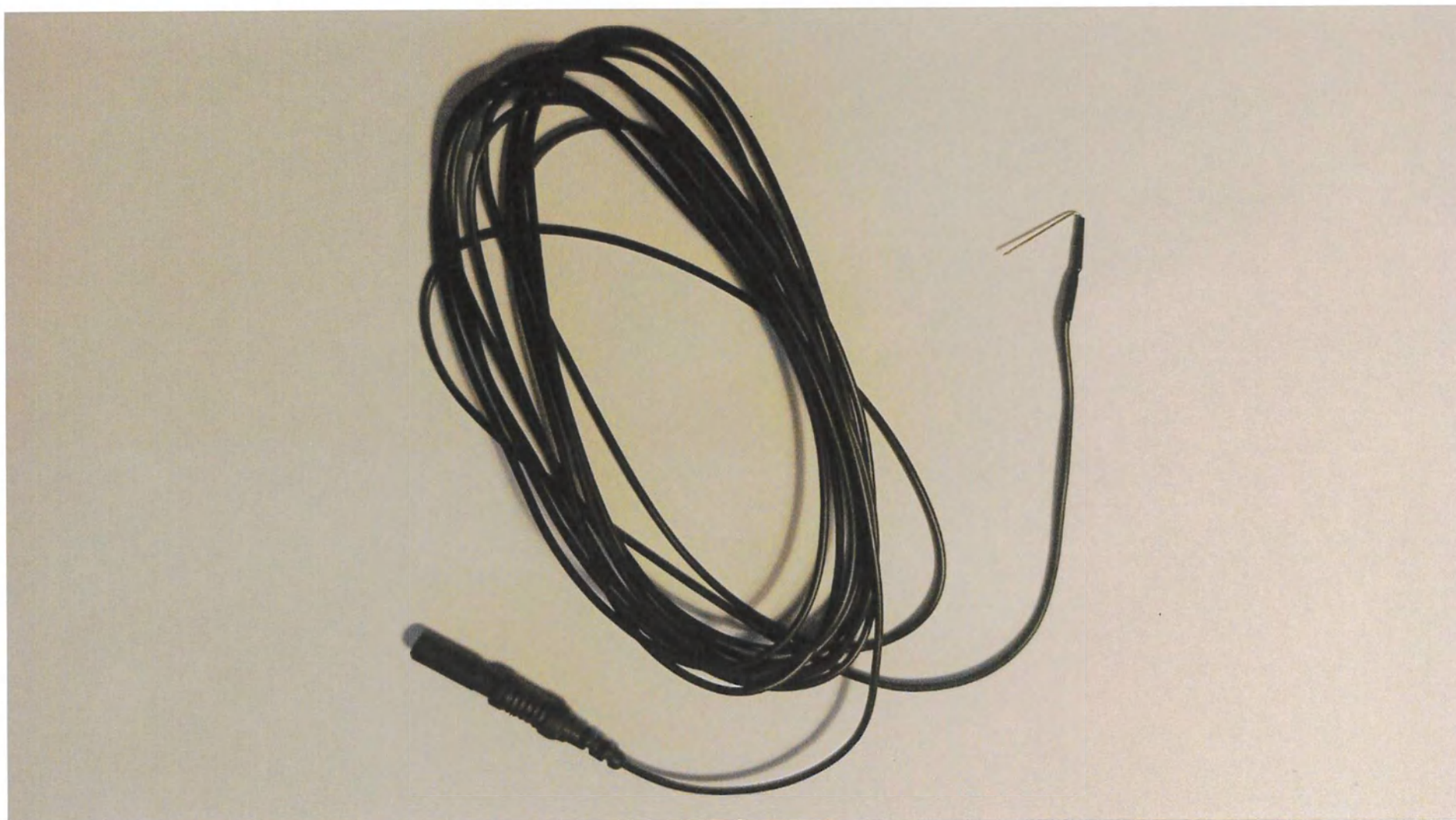
Электрод игольчатый подкожный монополярный с длиной иглы 13 мм, диаметром иглы 0.40 мм, углом наклона иглы 30° (150°), с кабелем длиной 250 см, артикул MN4013HD25SRU
