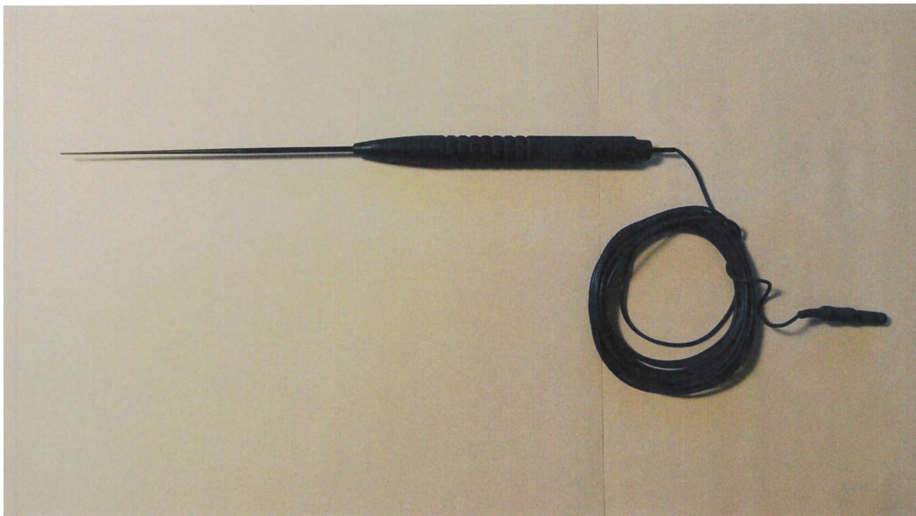
Электрод-зонд стимулирующий монополярный с гибким наконечником с длиной стержня 95мм, артикул SI1IF095S2526DRU
