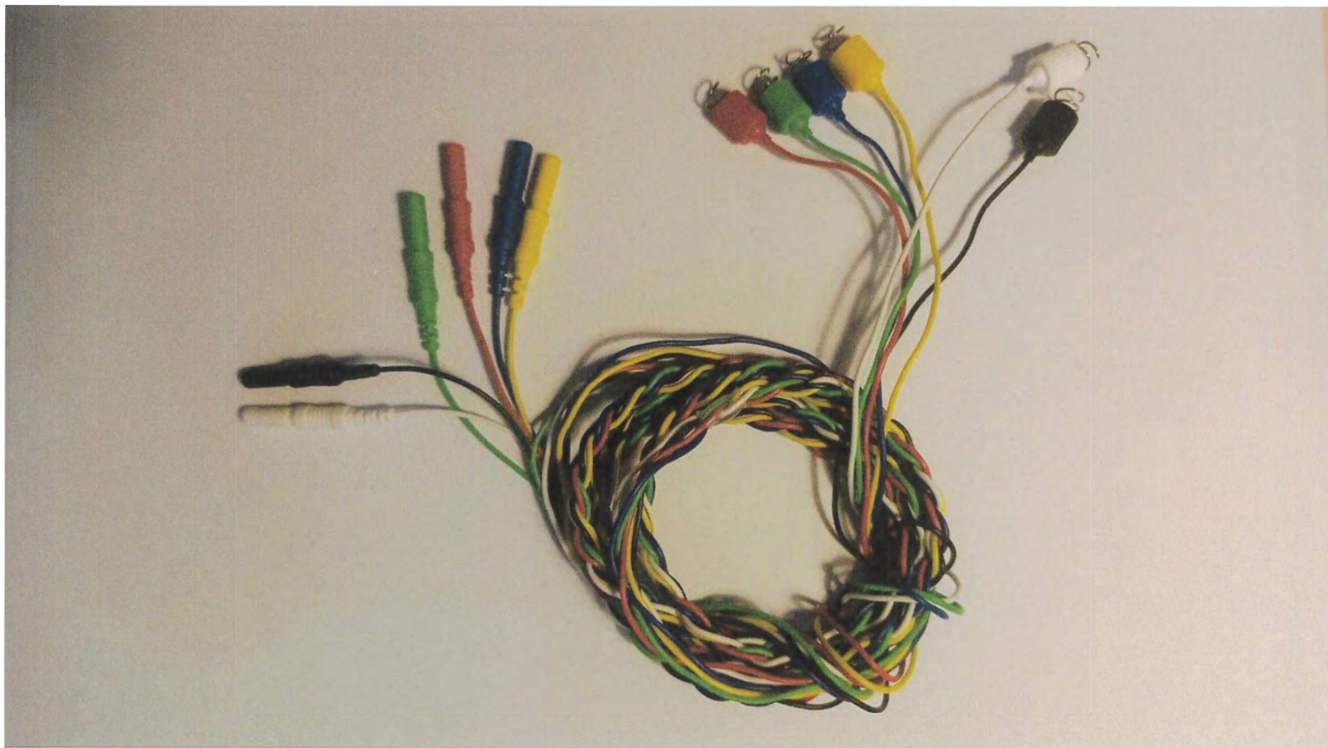
Электрод игольчатый штопорный 6-жильный, без экрана, с длиной иглы 5 мм, диаметром иглы 0.60 мм, с кабелем длиной 150 см, артикул MNCS0615DT6RU
