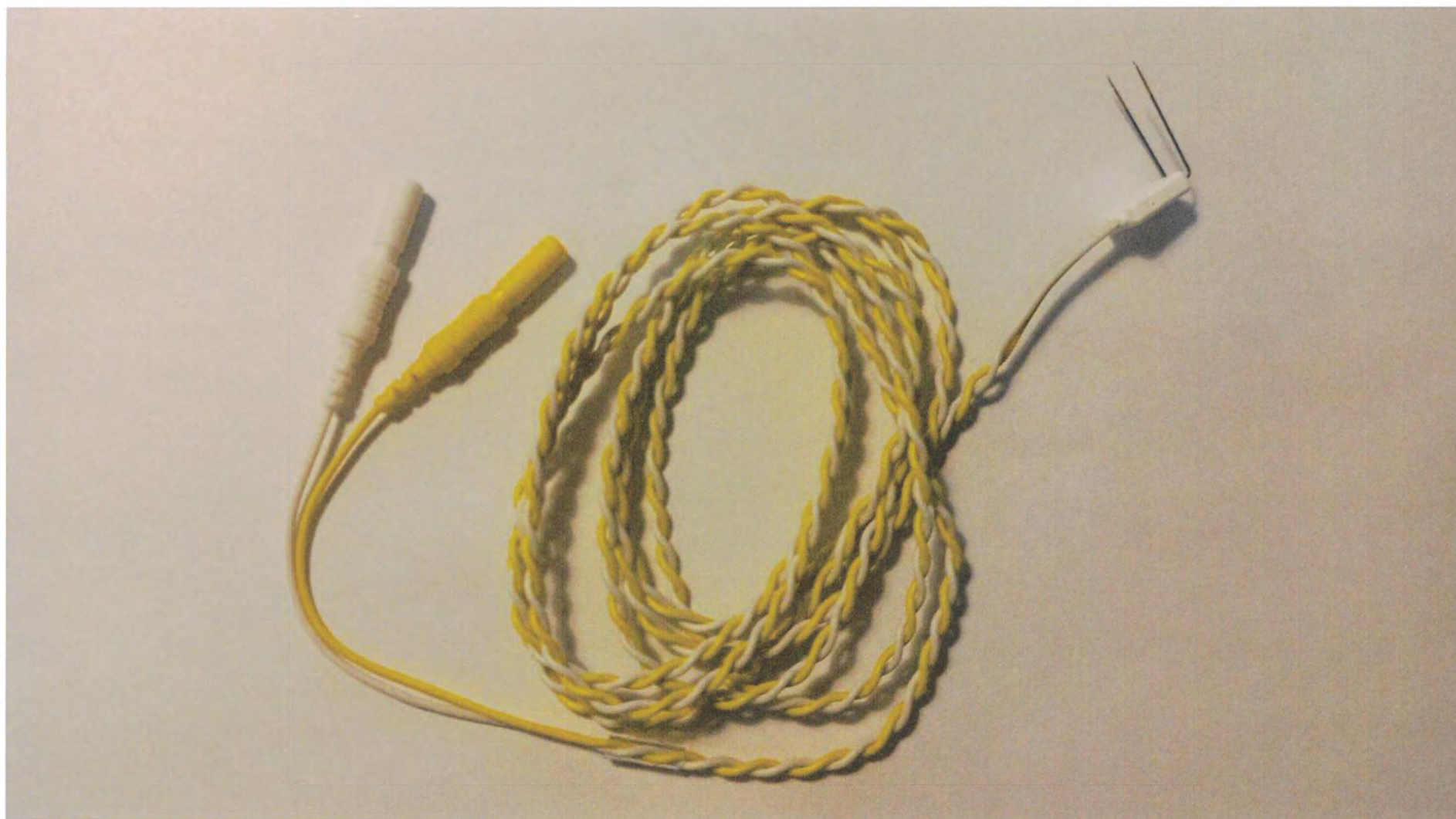
Электрод игольчатый парный скрученный с длиной иглы 18 мм, диаметром иглы 0.45 мм, с углом наклона иглы 30° (150°), расстоянием между иглами 5 мм, с кабелем длиной 150 см, артикул TFDN451841RU
