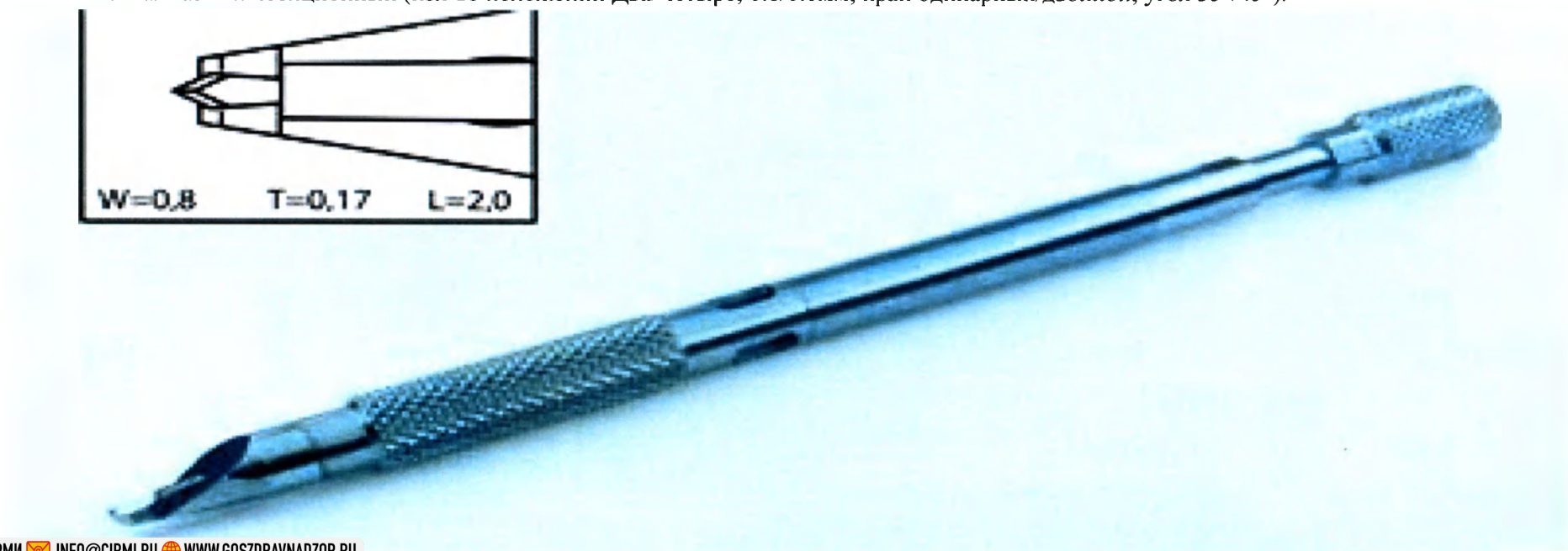
34. Нож алмазный позиционный (кол-во положений Два/Четыре; 0.8/0.1мм; край одинарный/двойной; угол 35°/45°).
