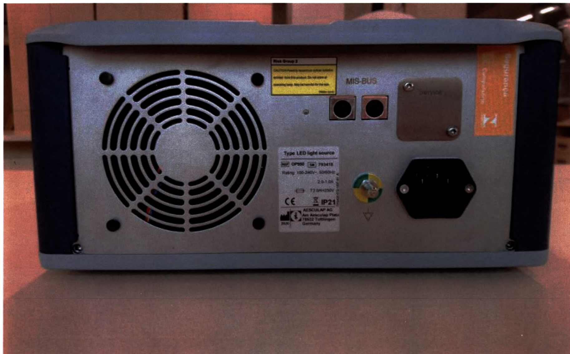
Источник света эндоскопический светодиодный (LED light source), арт OP950 – вид сзади
