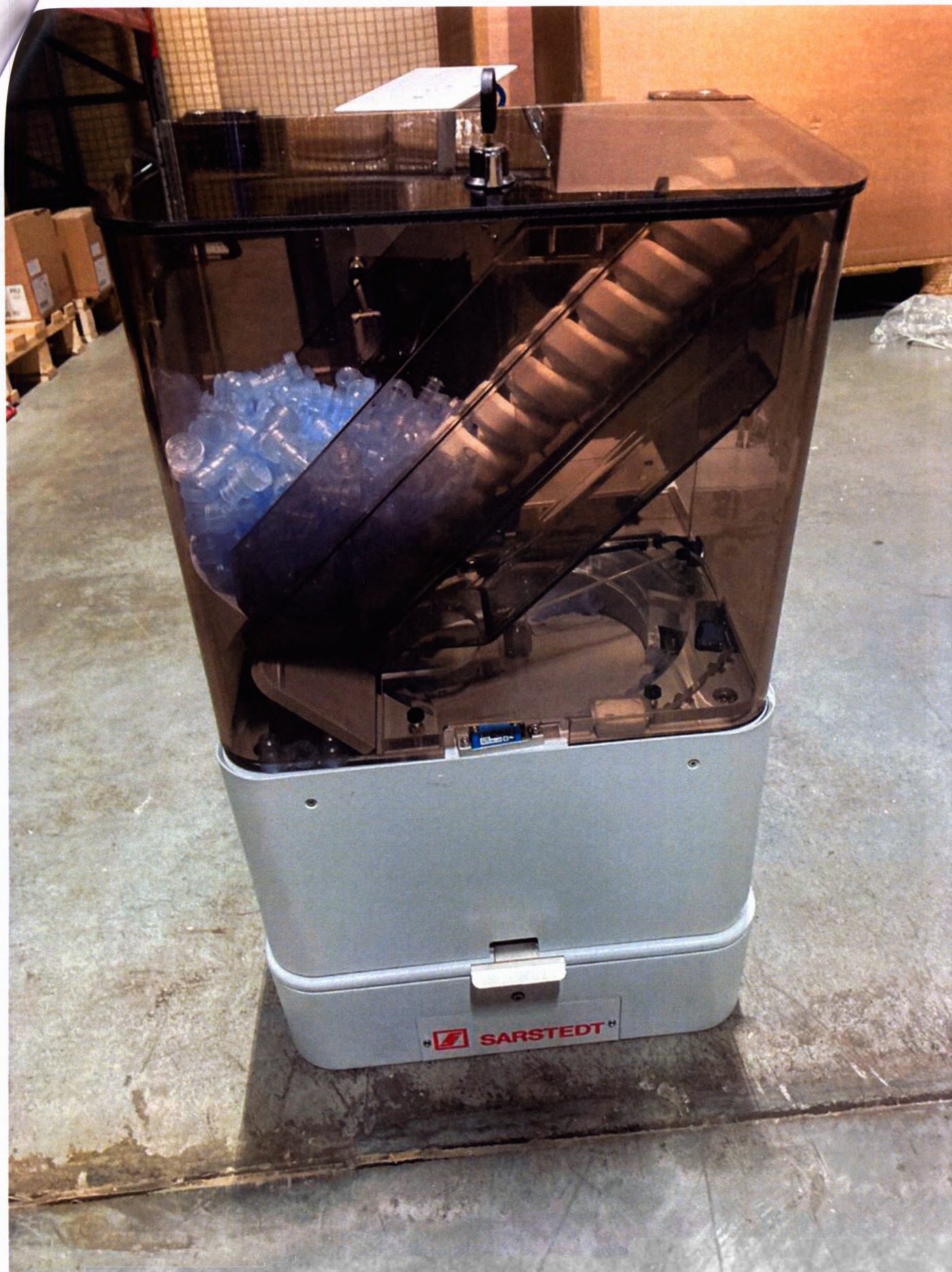
Рисунок 9. Фотографическое изображение Модуля надевания крышек, производства SARSTEDT AG&Co. KG.
