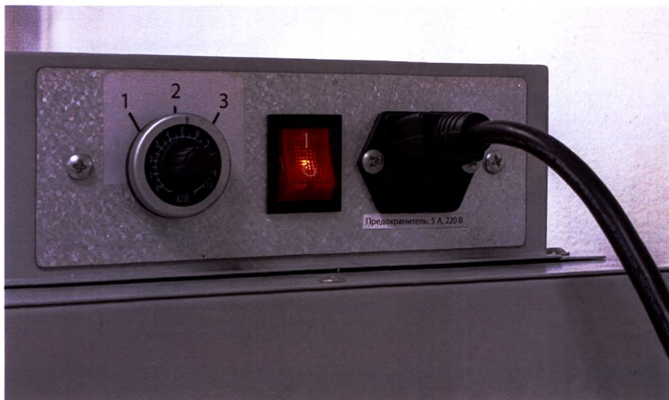
Фото кнопок управления и сетевого шнура фильтромодуля изделия с маркировкой вблизи держателя плавкого предохранителя
