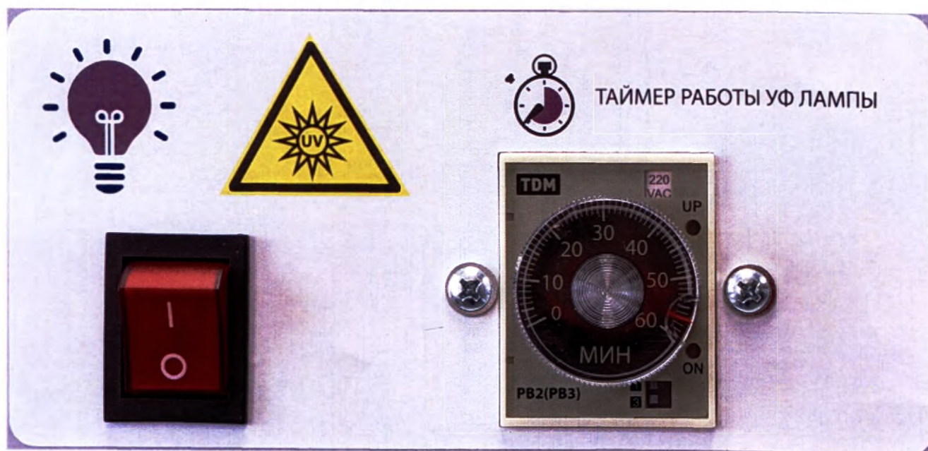
Фото выключателя и таймера УФ лампы изделия
