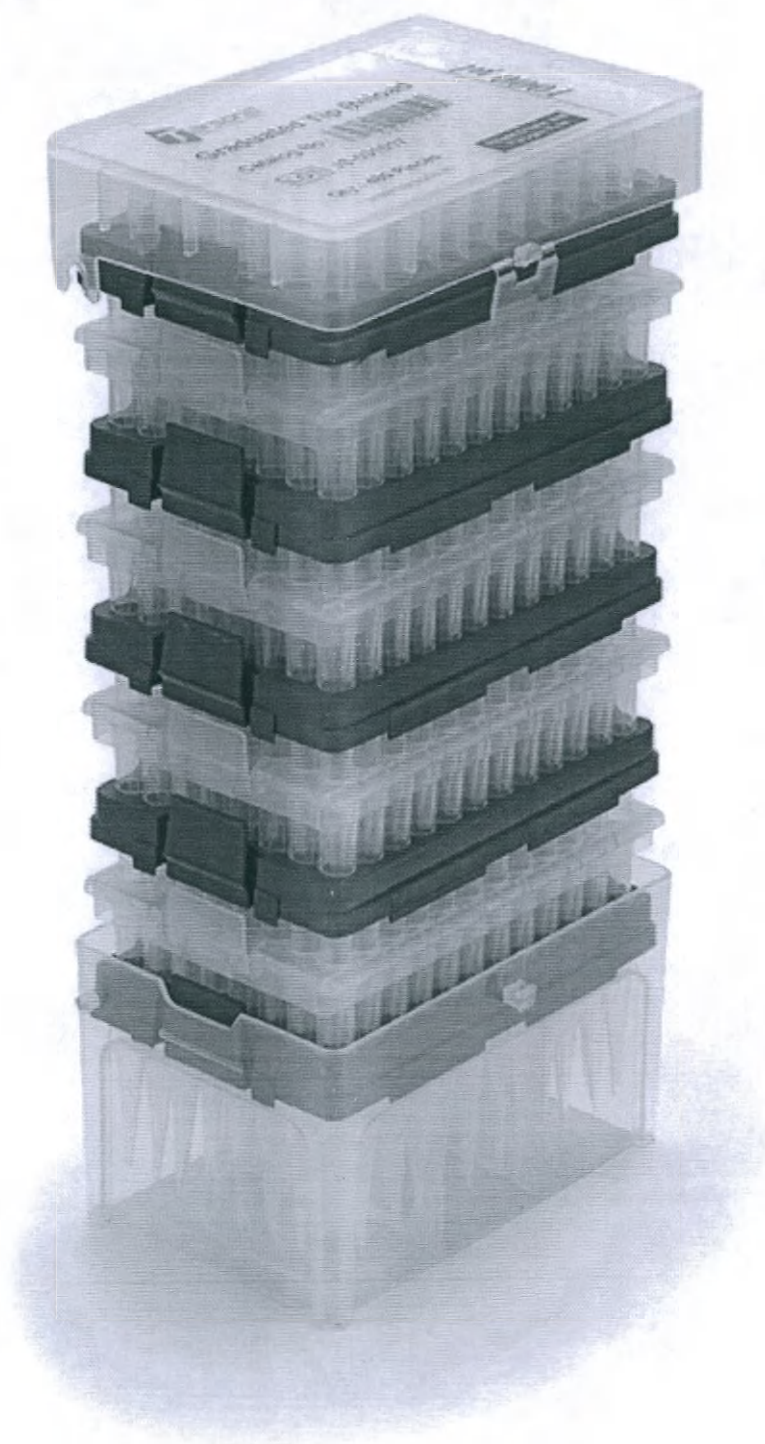
Наконечники одноразовые нестерильные для микропипеточных дозаторов, в сменных блоках, объемом 1000 мкл, градуированные (960 шт./уп.) Общий вид
