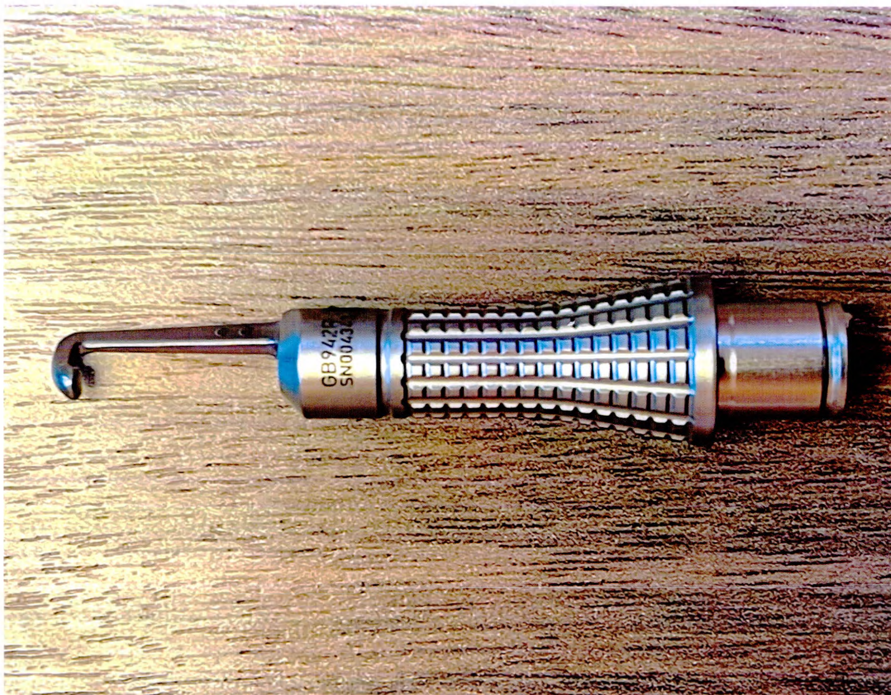
Фото 2.1. Наконечник краниотома с защитой ТМО стандартный фиксированный ELAN 4: GB942R – общий вид медицинского изделия
