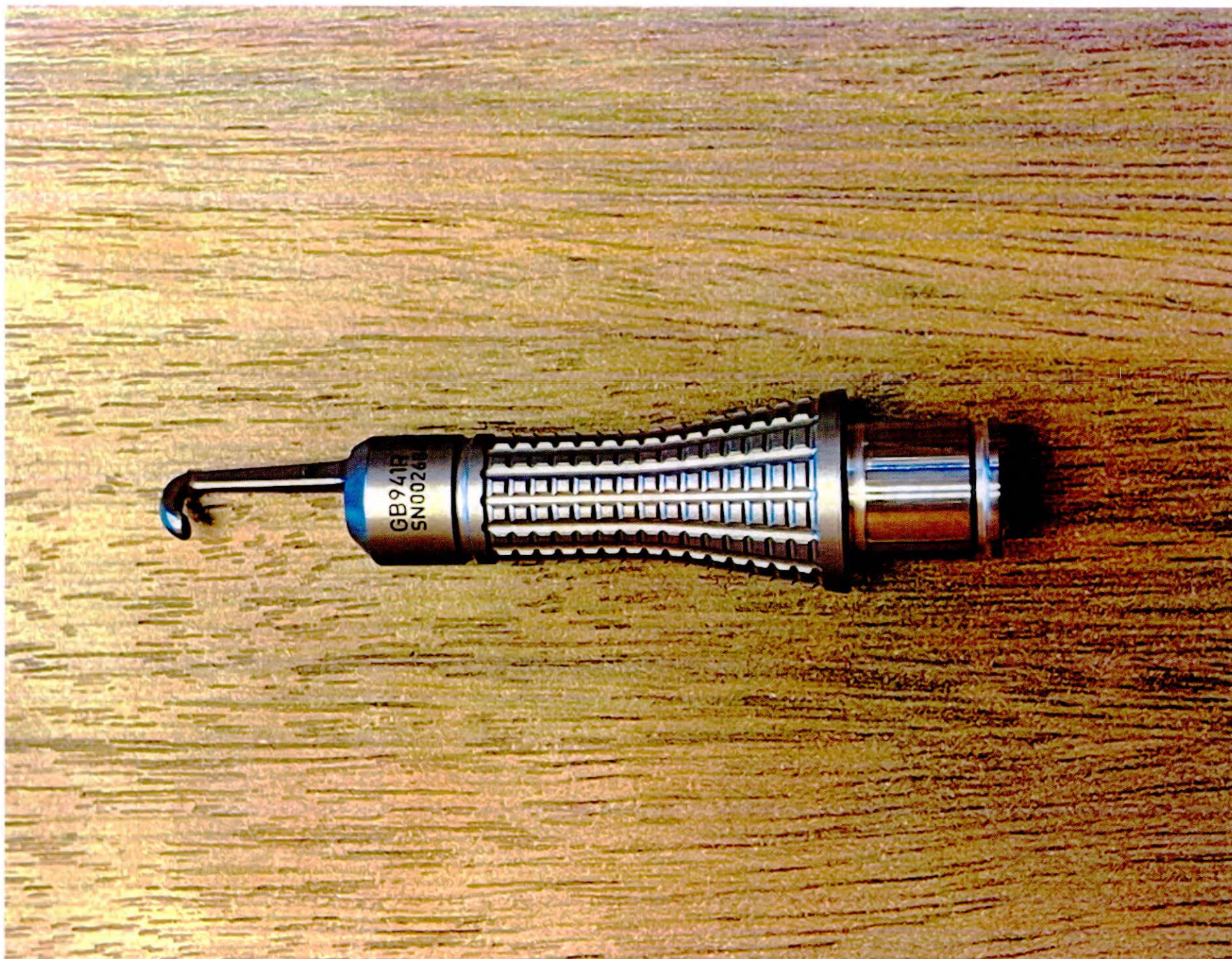
Фото 1.1. Наконечник краниотома с защитой ТМО малый фиксированный ELAN 4; GB941R – общий вид медицинского изделия
