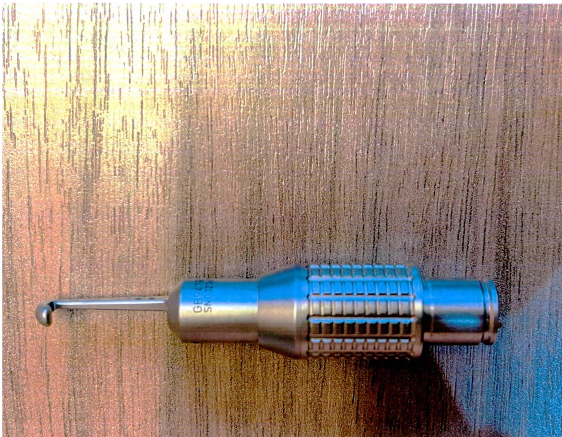
Фото 4.1. Наконечник краниотома с защитой ТМО стандартный ротационный ELAN 4: GB947R – общий вид медицинского изделия
