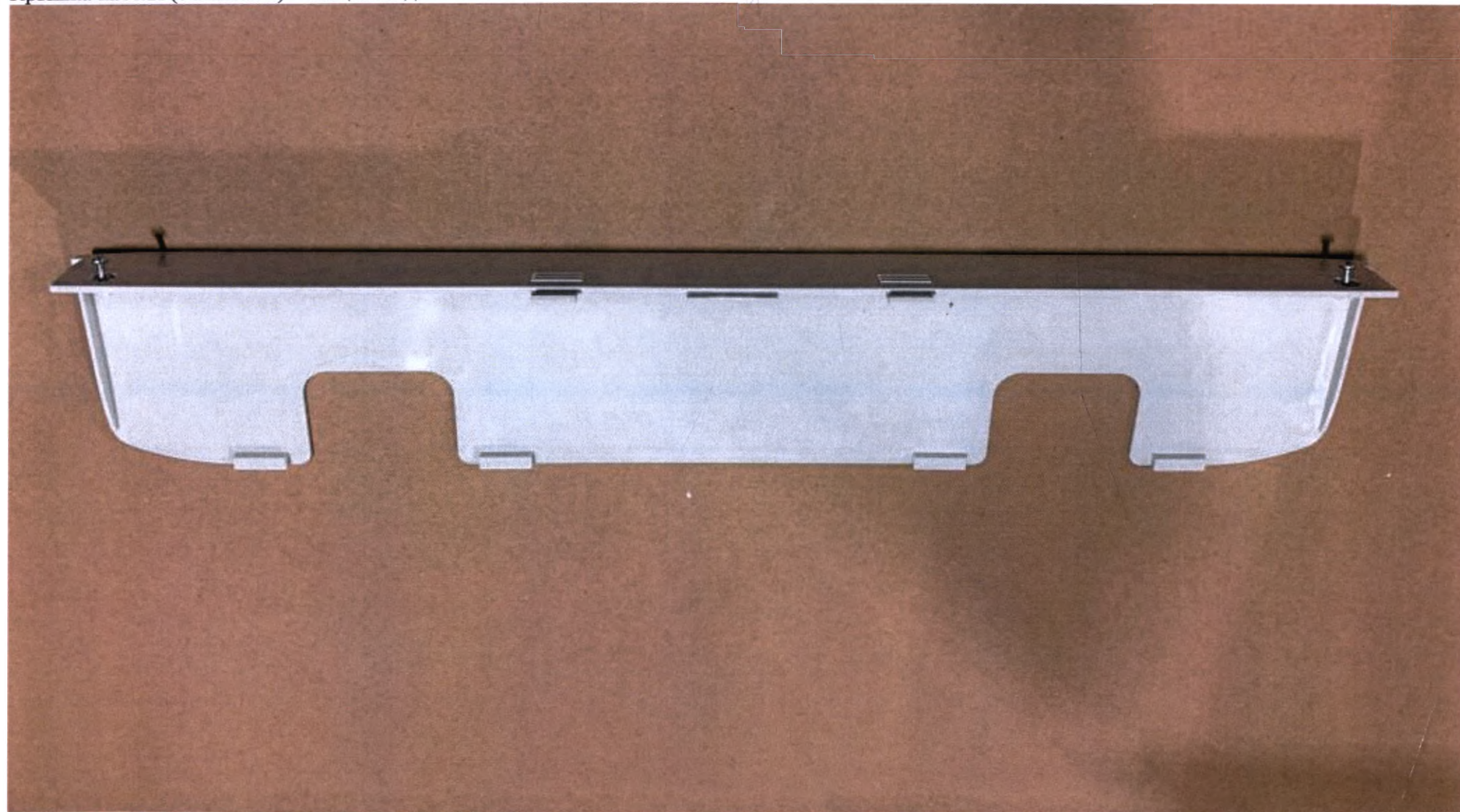
Крышка кабеля (с винтами) – общий вид
