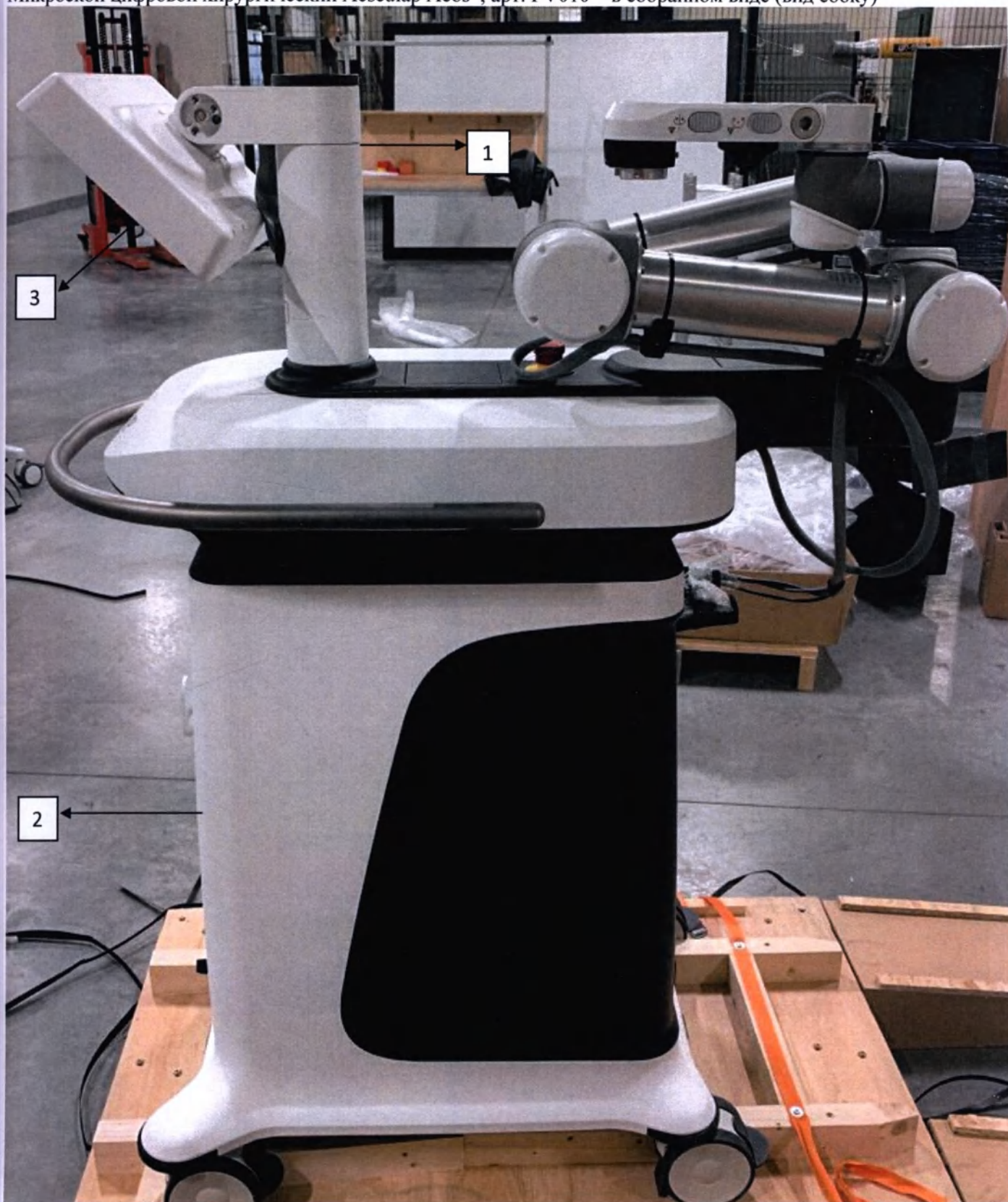
Микроскоп цифровой хирургический Aescular Aeos®, арт. PV010 – в собранном виде (вид сбоку)
