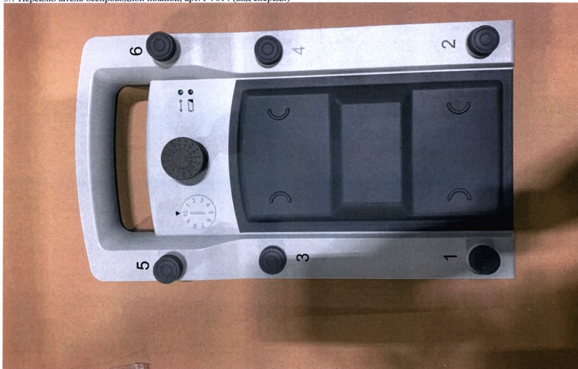
3.7 Переключатель беспроводной ножной, арт. PV014 (вид спереди)
