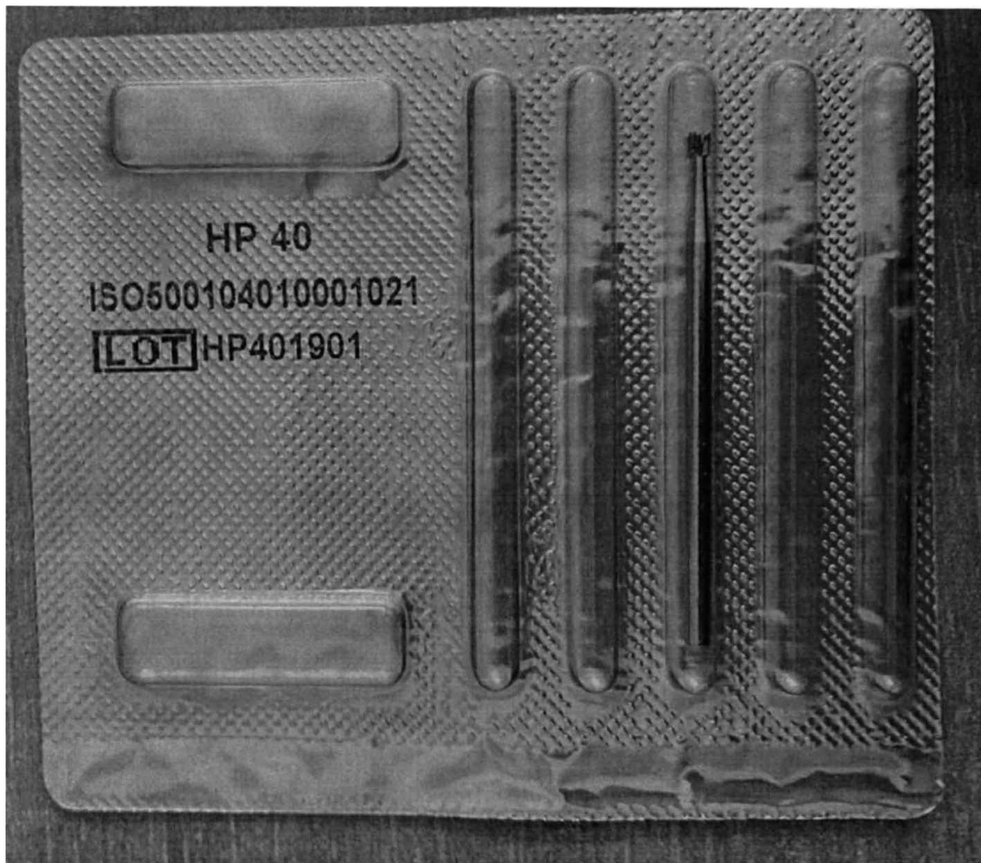
Рисунок 36– Бор стоматологический твердосплавный нестерильный одноразовый, восьмигранный, с хвостовиком типа HP 40, форма рабочей части: обратноконусная головка, код 500-104-010-001-021. LOT HP401901, срок годности 17.03.2029, в упаковке
