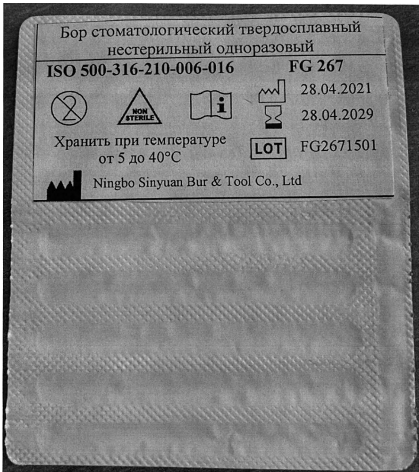
Рисунок 246 – Маркировка упаковки Бор стоматологический твердосплавный нестерильный одноразовый, шестигранный, с хвостовиком типа FG 267, форма рабочей части: конусная фиссурная головка с острым концом, код 500-315-210-006-016. LOT FG2671501, срок годности 28.04.2029
