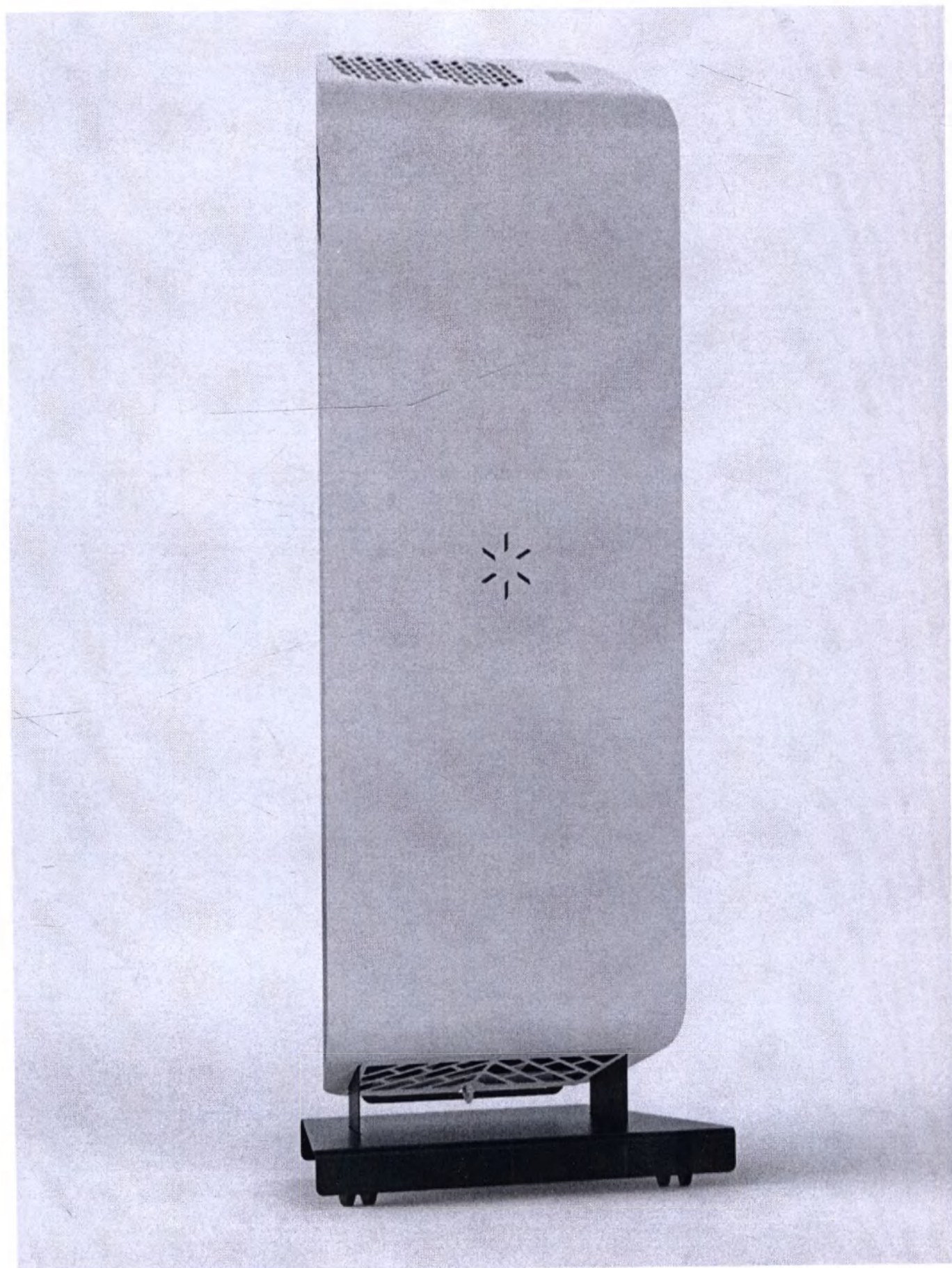
Облучатель-рециркулятор воздуха ультрафиолетовый бактерицидный Milerd® DZR-6 DM
