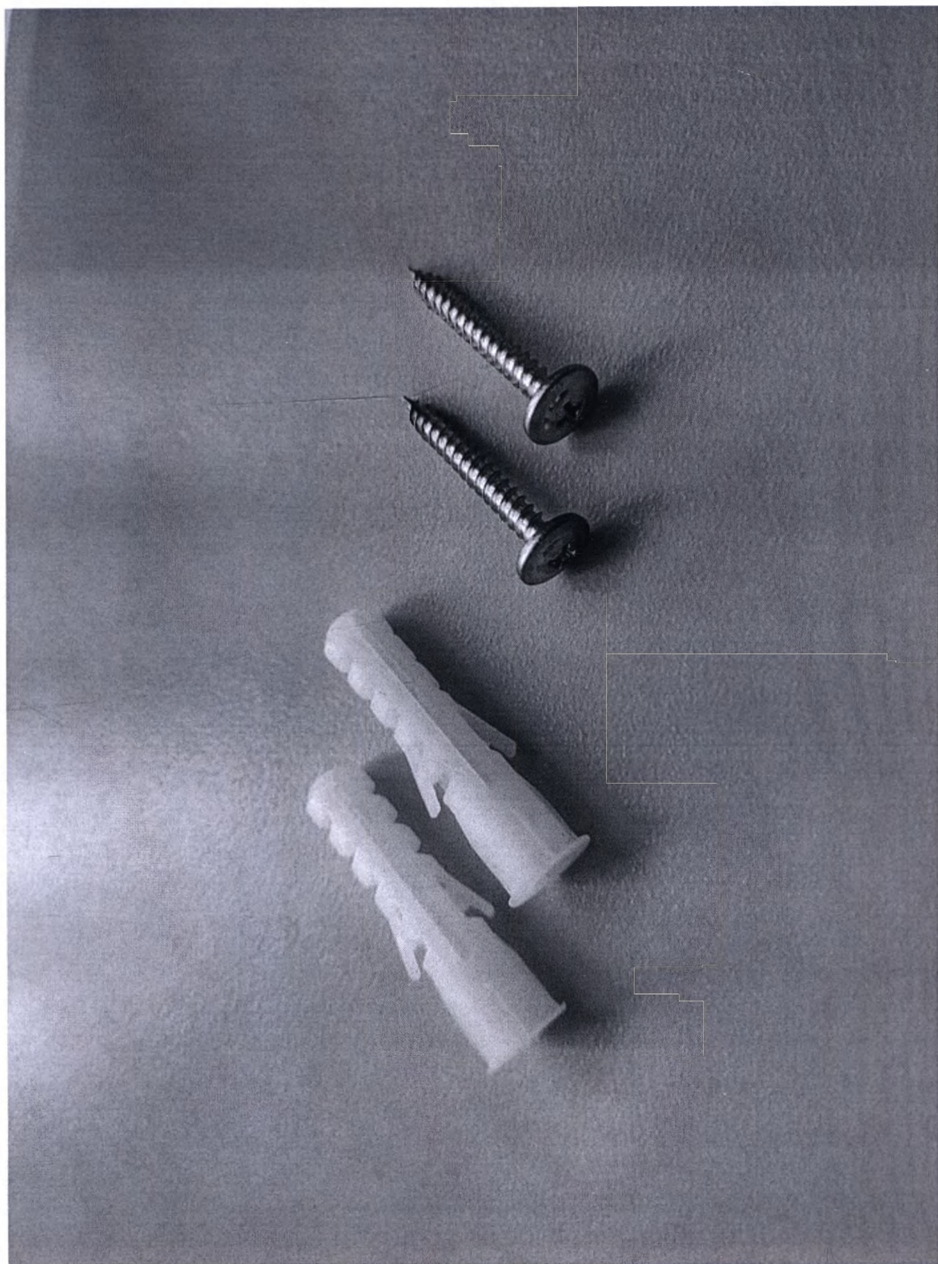
Набор крепежных элементов, в составе: Дюбель универсальный 6 x 42 - 2 шт; Саморез с прессшайбой 4,2 x 40
