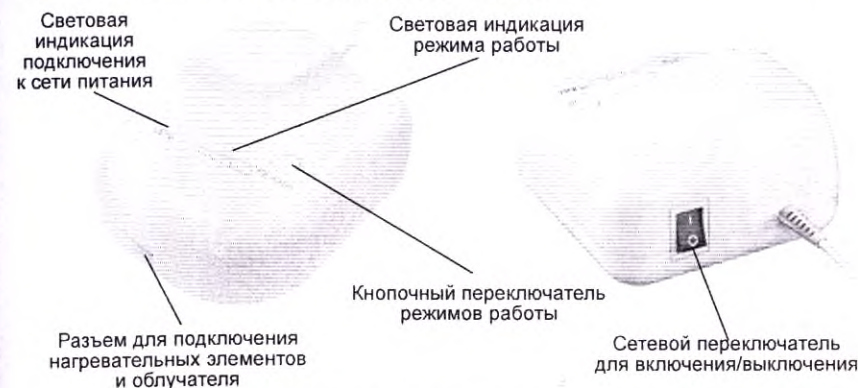
Рис. 2. Общий вид источника питания
