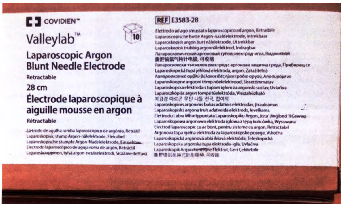
Рис. 22 Маркировка на транспортной упаковке Электрод-игла лапароскопический аргоновый тупой Valleylab, выдвижной, длиной 28 см
