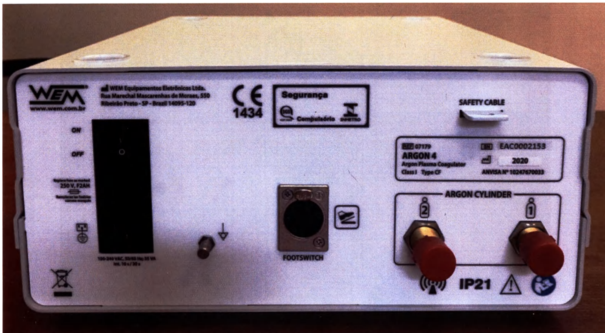
Рис. 2 Коагулятор плазменный Argon 4 (маркировка на задней панели).
