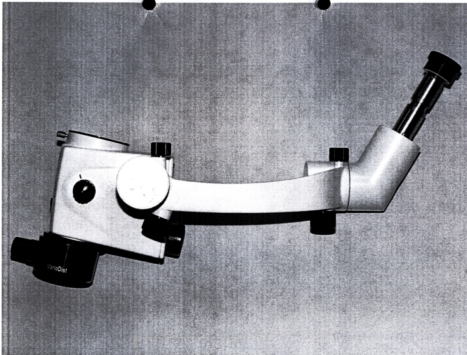
Рис. 12 Оптическая головка с соединительным плечом, с 6-ступенчатым переключателем увеличения, встроенным оранжевым и зеленым светофильтром и объективом
