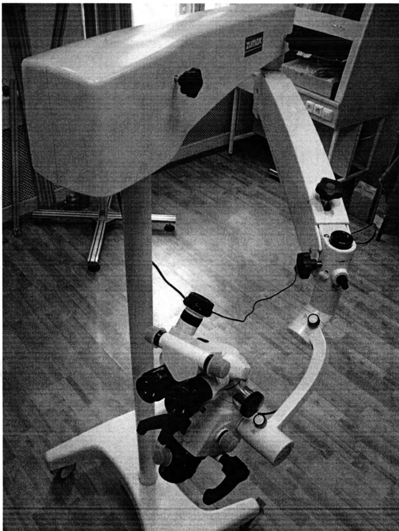
Рис. 1 Микроскоп стереоскопический операционный OMS 2350 в сборе
