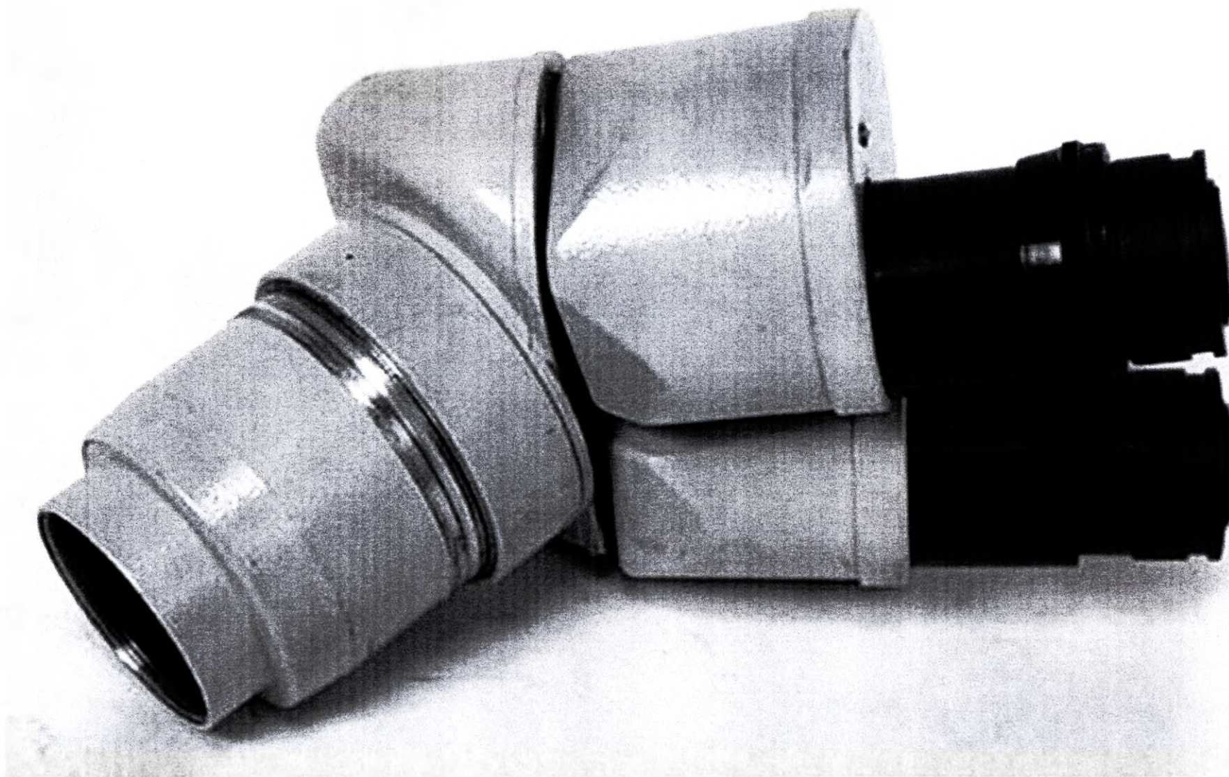
Рис. 31 Тубус бинокулярный с углом наклона 45^\circ
