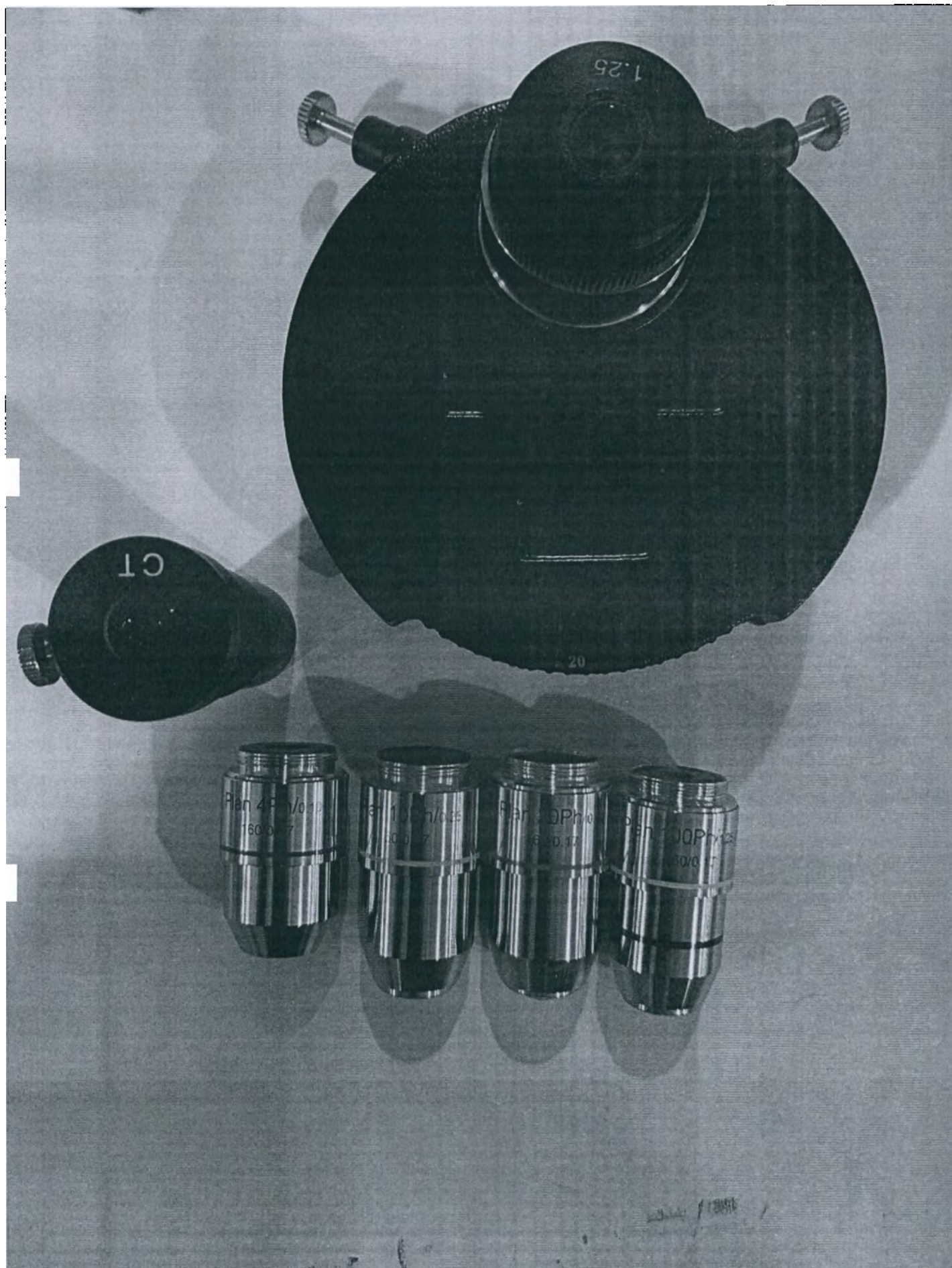
Микроскоп биологический Биолаб 6Т для лабораторной диагностики in vitro .. Устройство фазово-контрастное (опционально)
