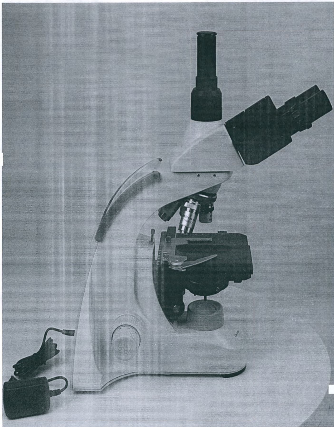
Микроскоп биологический Биолаб 5Т для лабораторной диагностики in vitro. Общий вид
