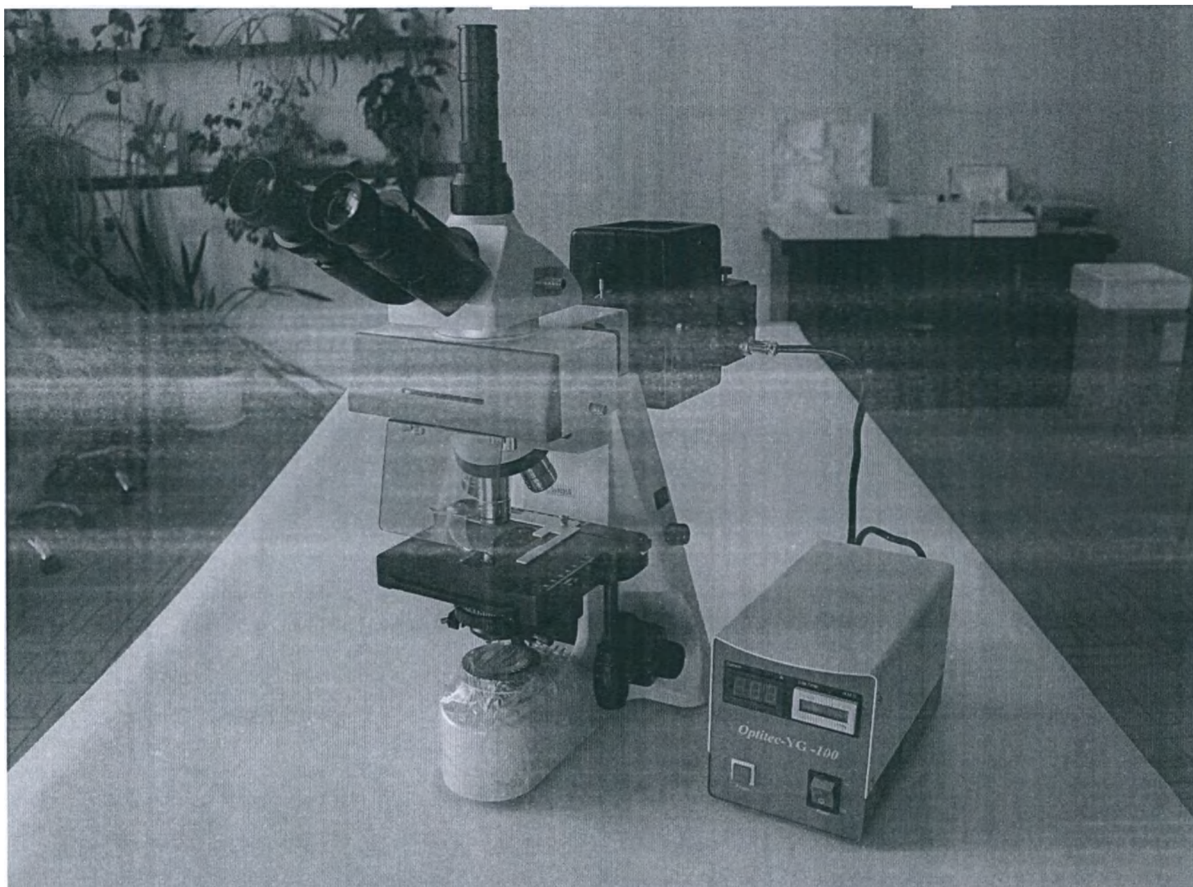
Микроскоп биологический Биолаб 11ЛЮМ для лабораторной диагностики in vitro . Общий вид
