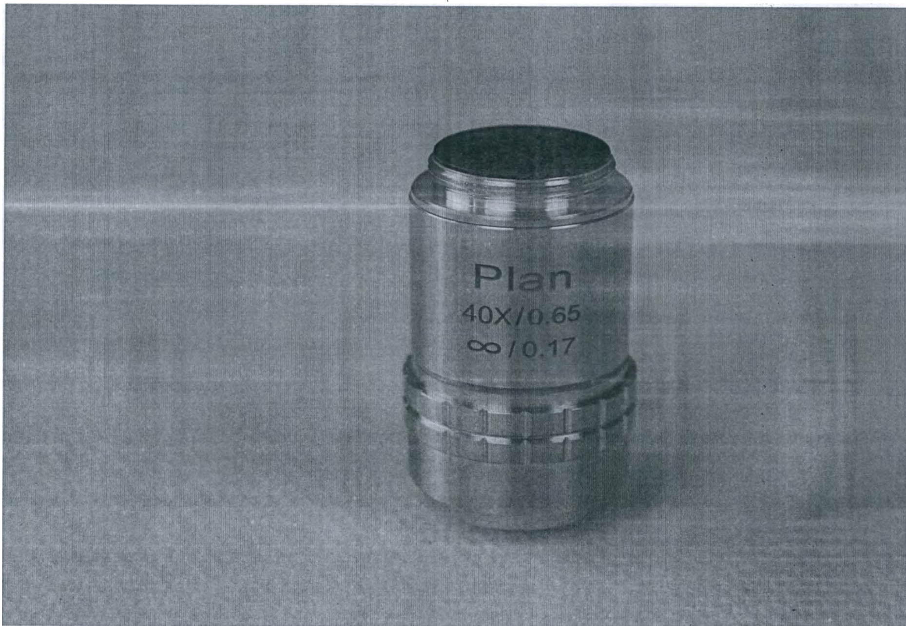
Микроскоп биологический Биолаб 6 ПРО для лабораторной диагностики in vitro .. Объектив Планахромат Plan 40x/0,65.
