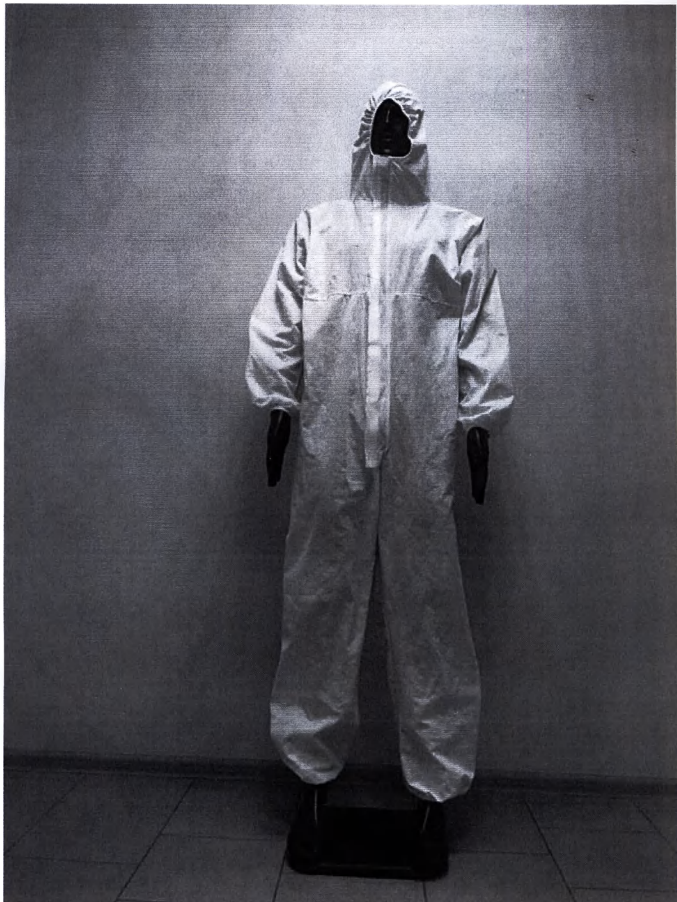
Рис.16 Костюм медицинский изолирующий К-2 (Вид спереди на манекене)
