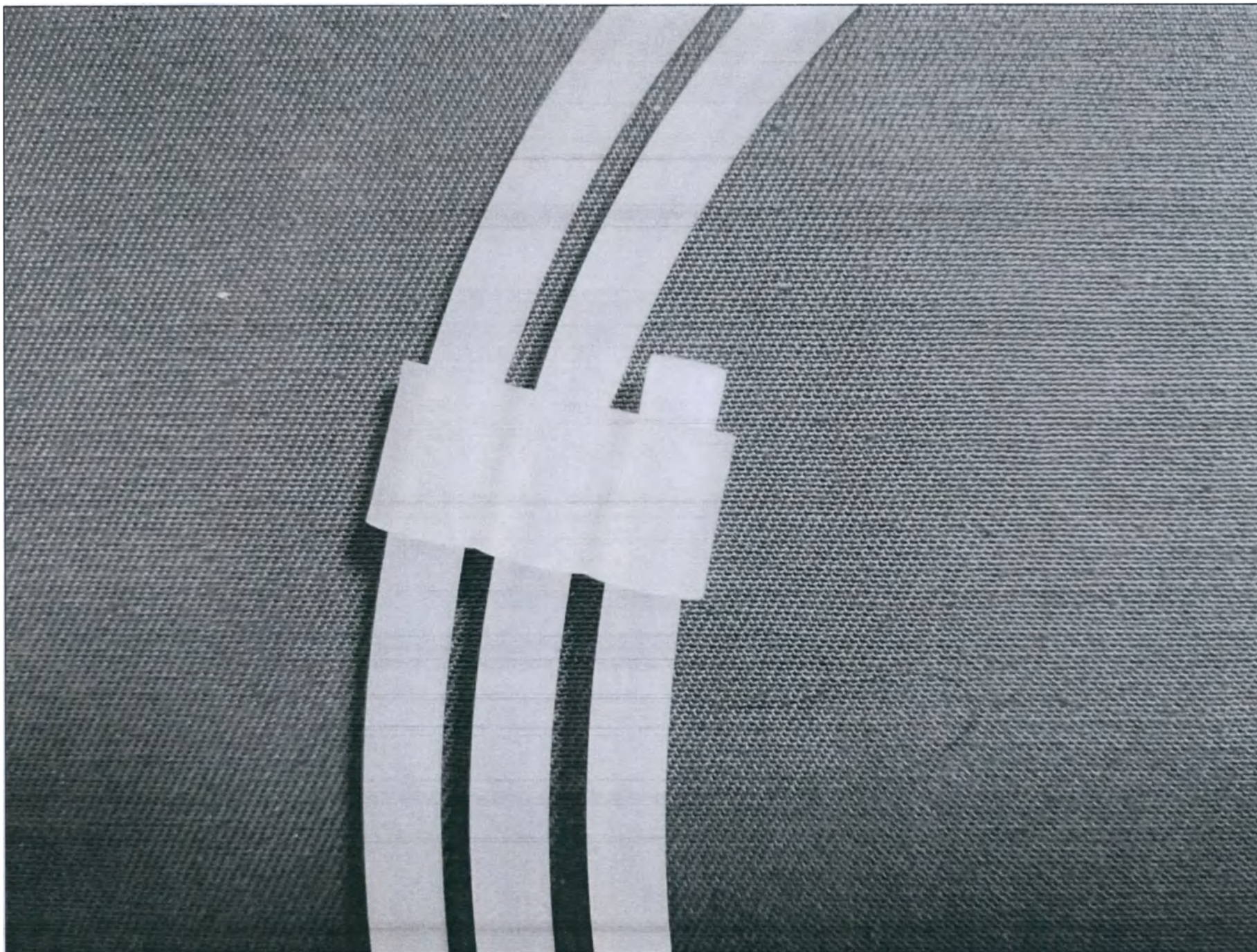
Рис. 11. Катетер баллонный дилатационный для коронарной ангиопластики ПИТОН RX, размер баллона: 4,0 мм x 30 мм по ТУ 32.50.13-001-15624048-2021
