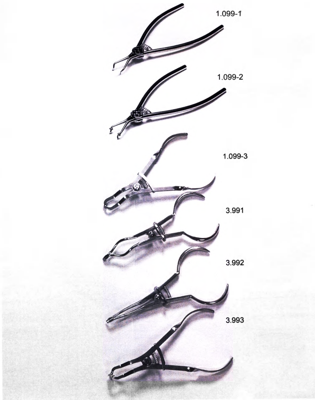
Рис. 29. Щипцы установочные № 1.099-1, № 1.099-2, № 1.099-3, № 3.991, № 3.992, № 3.993
