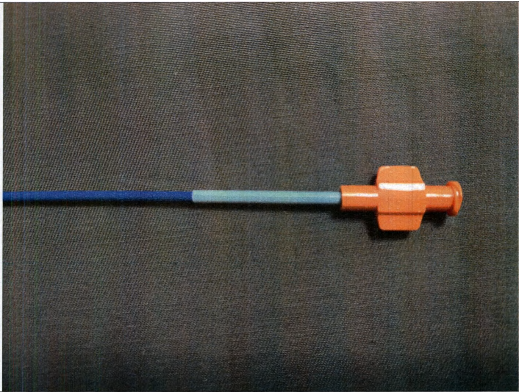
Рис. 29. Катетер внутрисосудистый проводниковый WINDOW, JR4.5, диаметр 7F, длина 100см.
