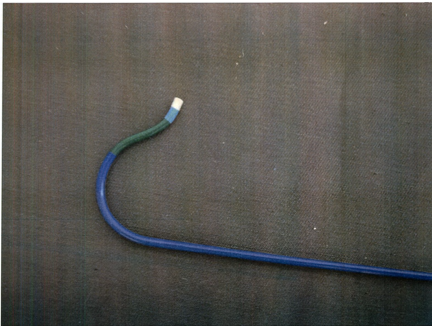
Рис. 9. Катетер внутрисосудистый проводниковый WINDOW, AL2.0, диаметр 7F, длина 100см.
