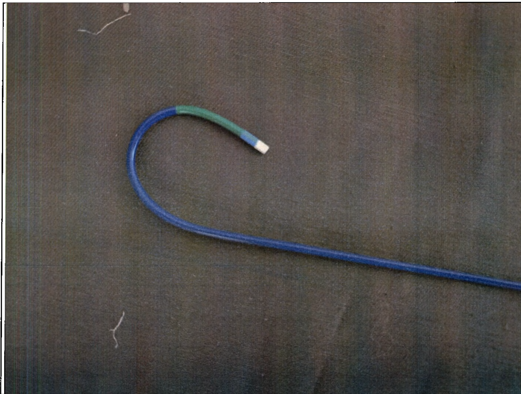
Рис. 37. Катетер внутрисосудистый проводниковый WINDOW, XB3.0, диаметр 6F, длина 100см.
