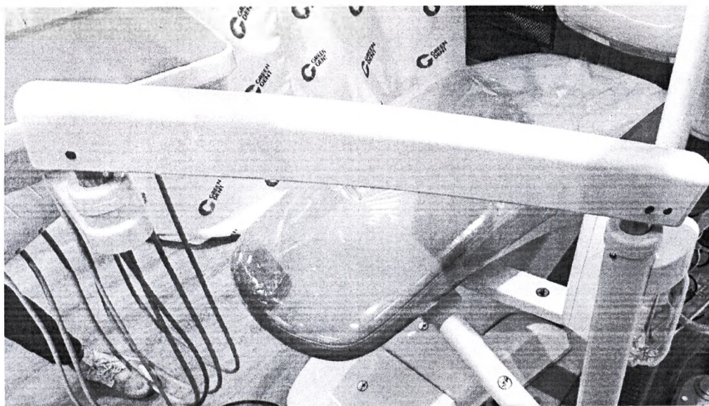
5.5 Рычаг пантографический
