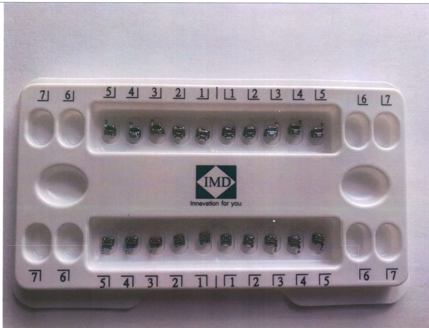
2.2 Фотография общего вида нескольких видов брекетов (на разные типы зубов) на примере типоразмерного ряда комплектующей «Брекеты»: Брекет металлический самолигирующий ProMIM Self-Ligating McBeTr Bracket 0,022 дюйма (0,56 мм)
