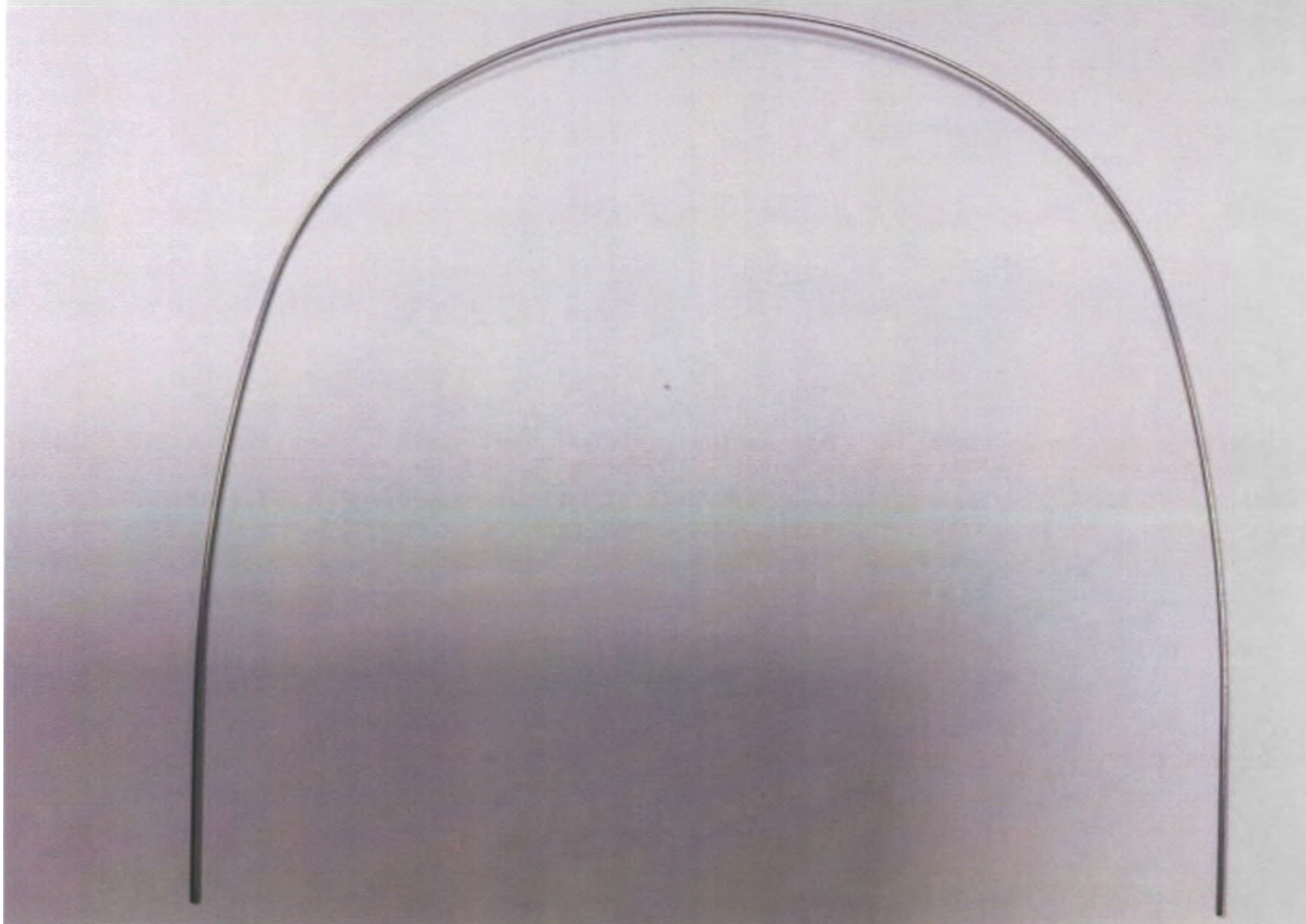
1.3. Дуга ортодонтическая, в варианте исполнения: Дуга ортодонтическая NITI MEMAlloy, сечение круглое, форма Нейчерал, 0,016 дюймов (0,41 мм), верхняя челюсть
