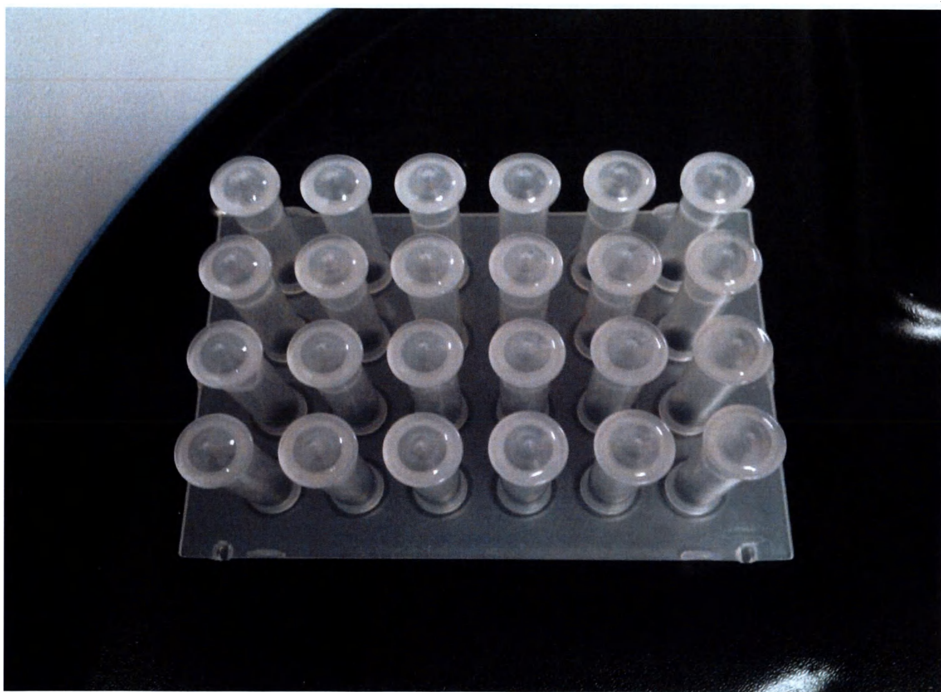
10. Комплект для KingFisher Flex 24 гребенка наконечников и планшет, по 50 штук каждой позиции (KingFisher Flex 24 deep well tip comb), в составе: - Гребенка наконечников для KF 24 Flex (KF24 Flex tip comb);
