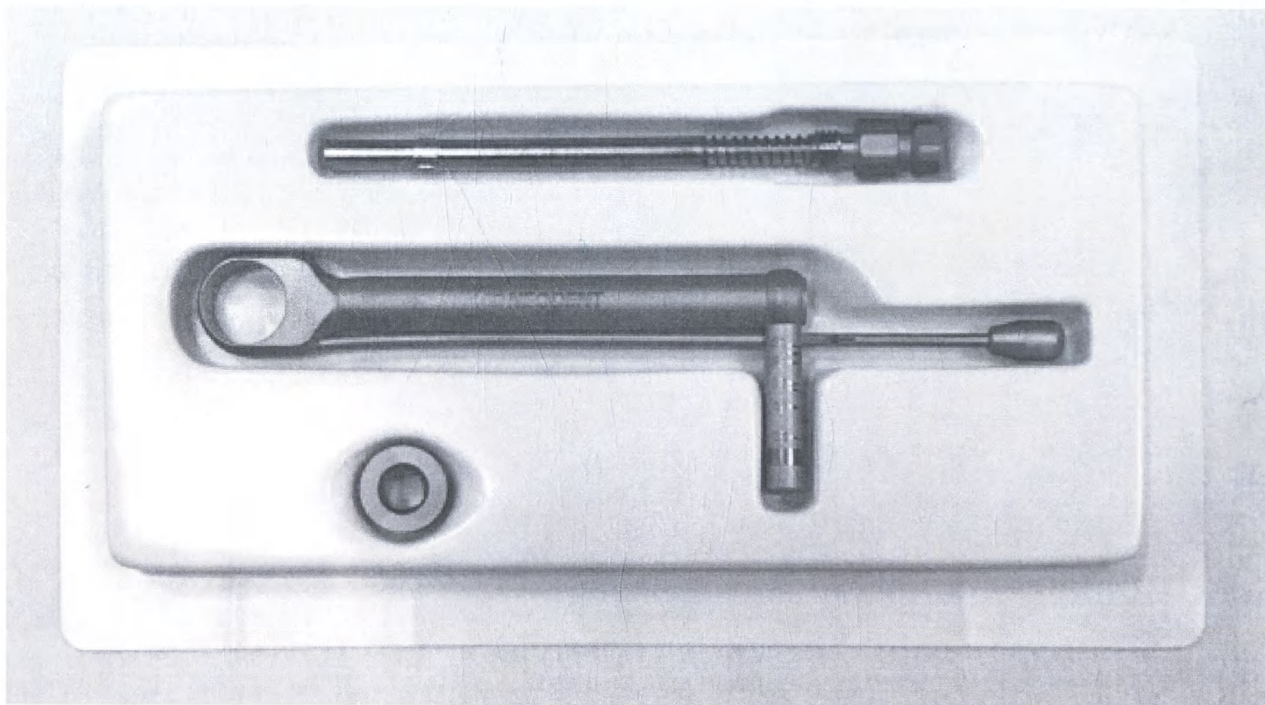
Рис. 3 Ключ динамометрический, в составе: зубчатое колесо, внутренний вал, корпус динамометрического ключа с встроенной трещоткой в пластиковом блистере
