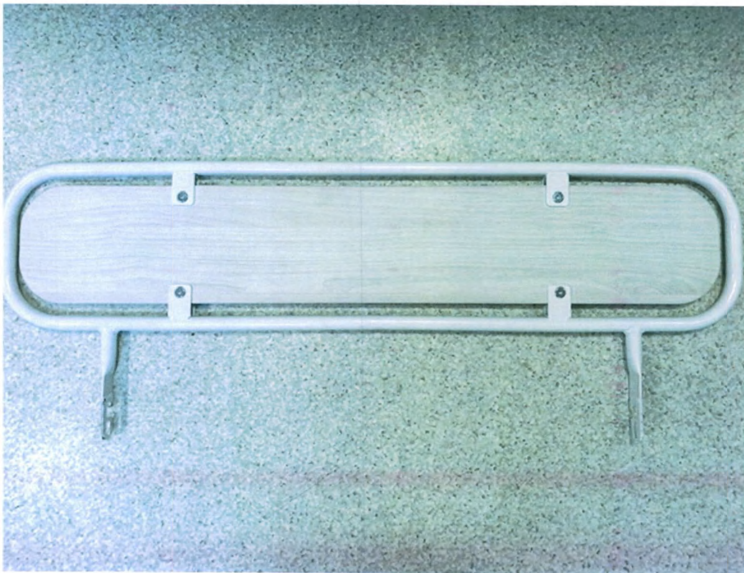
Рис. 1.1.1. Ограждение боковое MBW-01 (внешний вид)- металлическая труба со вставкой ЛДСП.
