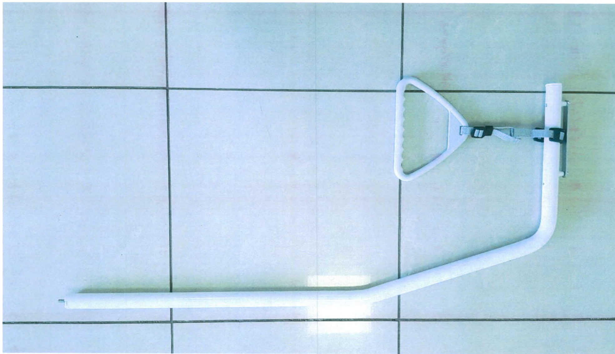
Рис. 2.5.1. Штанга для подвески ручных опор MBR-01.
