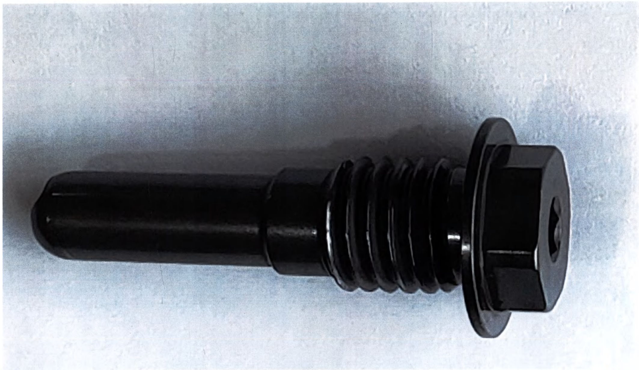
Заглушка проксимального бедренного антитротационного стержня (PFNA) условный номер 0
