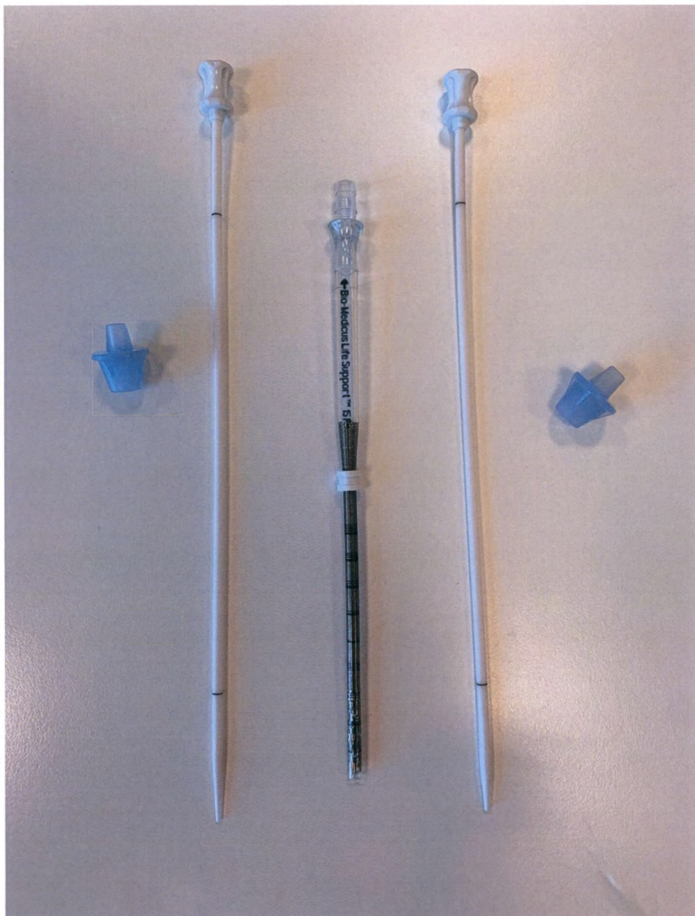
Рисунок 5. Катетер дренажный и интродьюсеры Bio-Medicus Life Support, длина катетера 11,5 см, наружный диаметр катетера 15 Fr (5,05 мм): Катетер, Интродьюсер с цельным коническим кончиком, Интродьюсер для использования с проводником, Колпачок гемостатический, Кольцо шовное рентгеноконтрастное регулируемое
