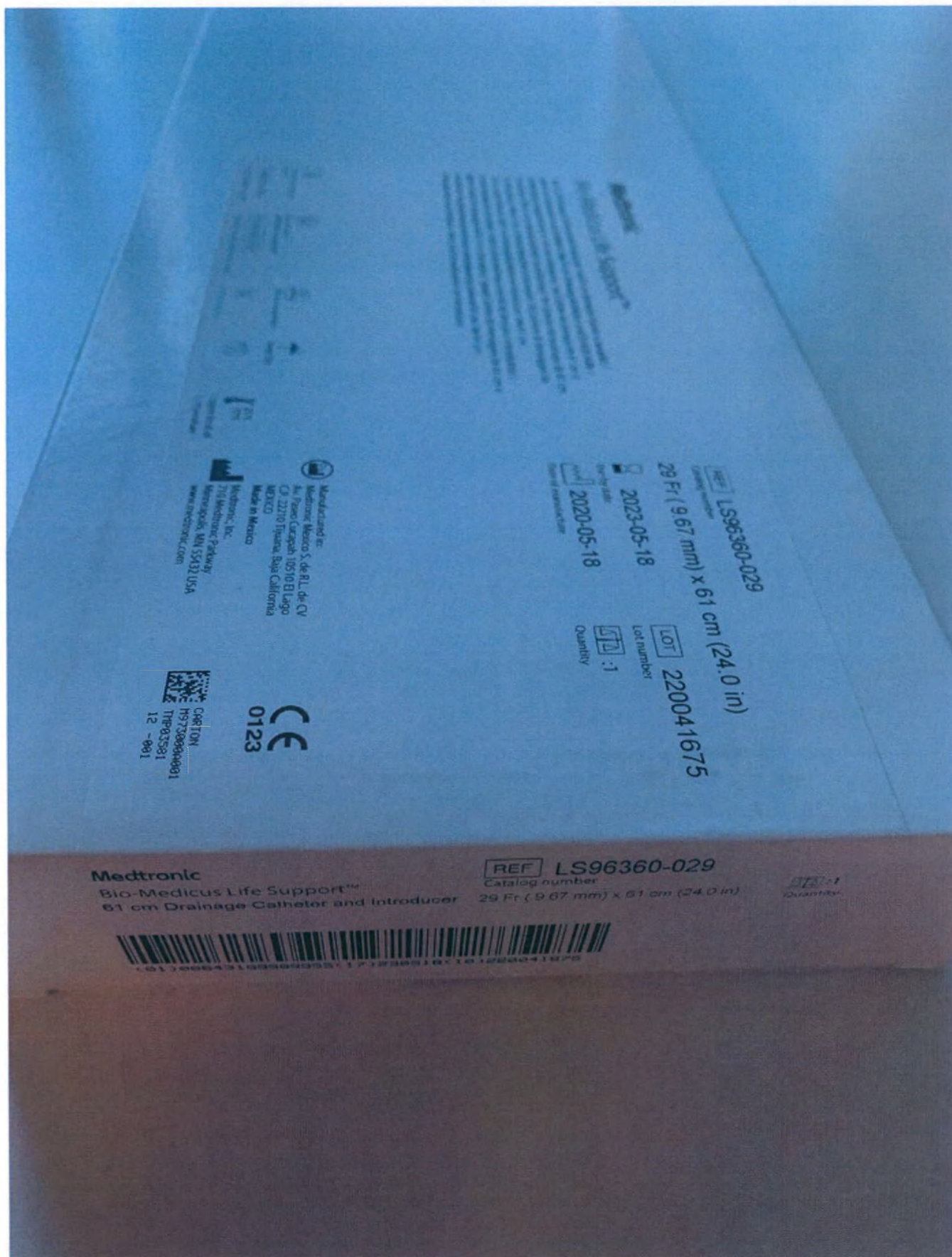
Рисунок 55. Потребительская упаковка Катетера дренажного и интродьюсера Bio-Medicus Life Support, длина катетера 61 см, наружный диаметр катетера 29 Fr (9,67 мм)
