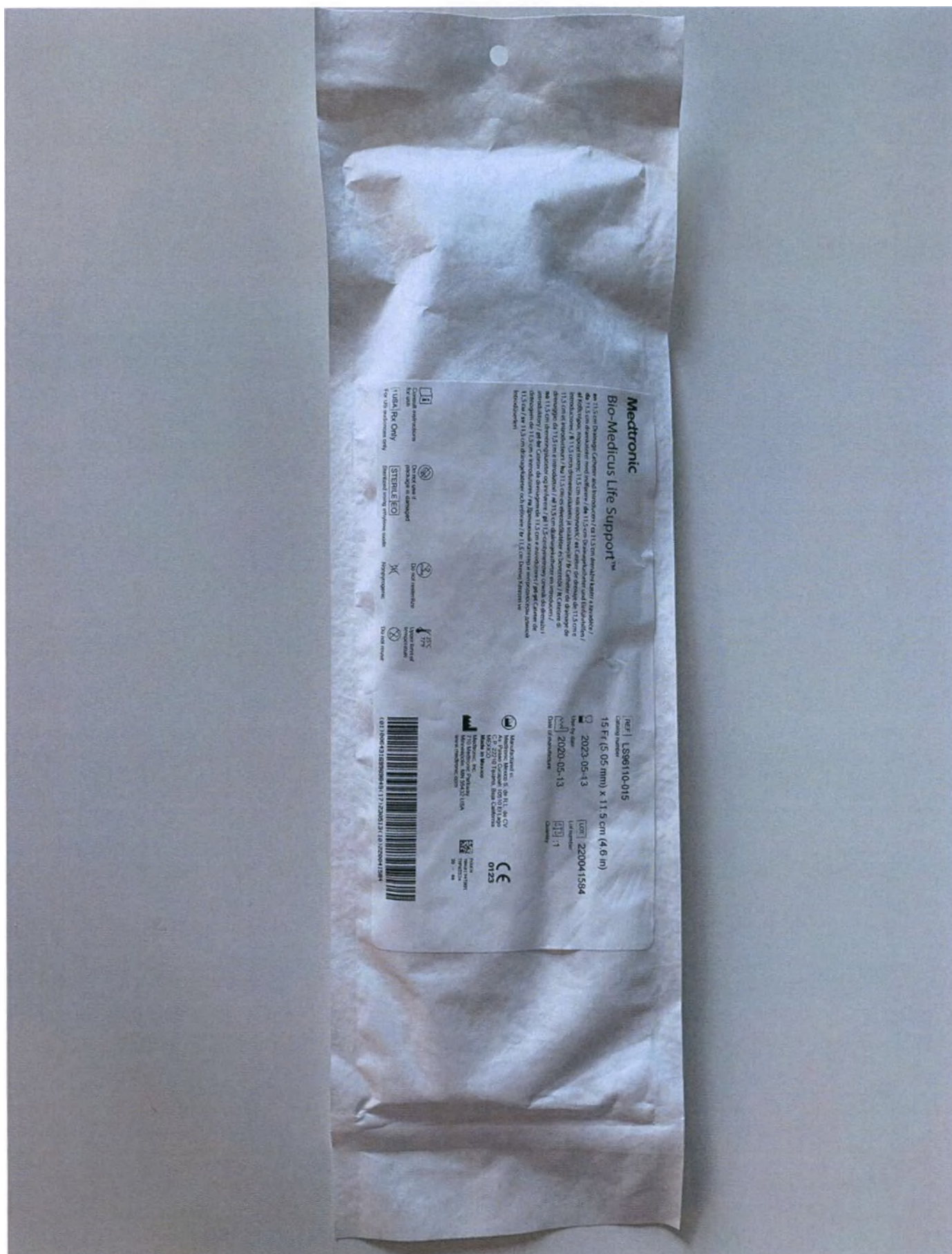
Рисунок 3. Стерильная упаковка Катетера дренажного и интродьюсеров Bio-Medicus Life Support, длина катетера 11,5 см, наружный диаметр катетера 15 Fr (5,05 мм)
