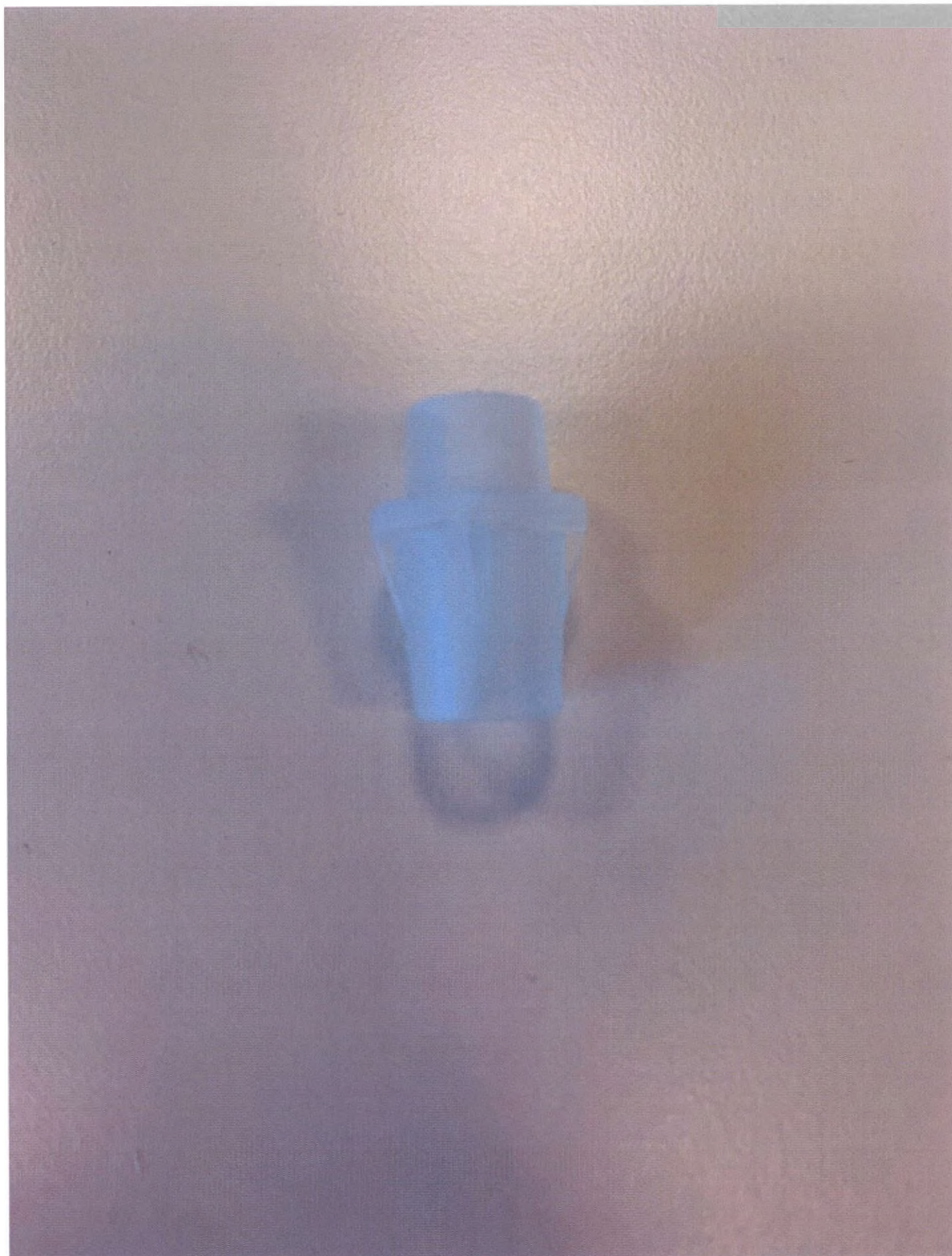
Рисунок 29. Катетер и интродьюсер Bio-Medicus Life Support, длина катетера 18 см, наружный диаметр катетера 25 Fr (8,36 мм): Колпачок гемостатический,
