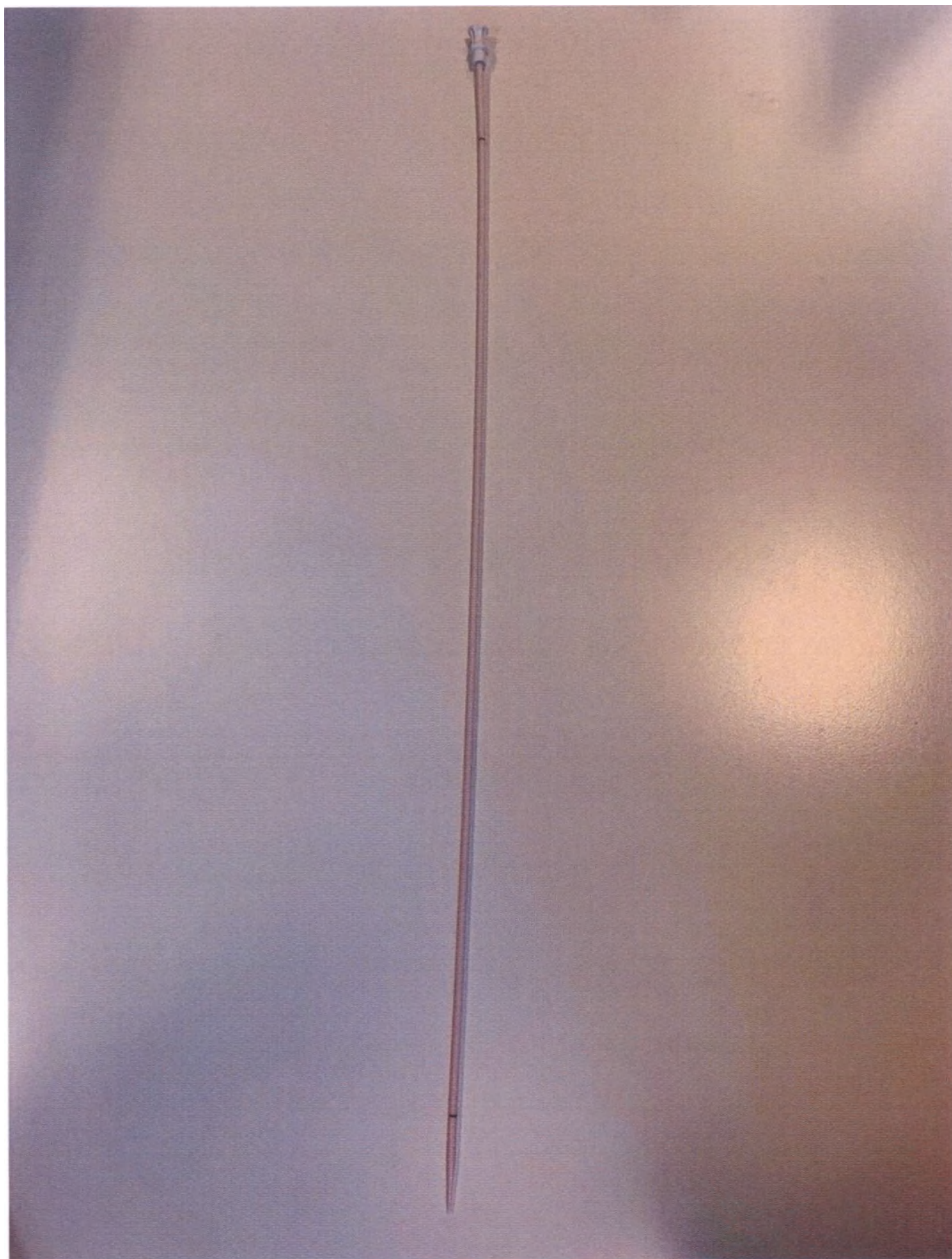
Рисунок 70. Катетер и интродьюсер Bio-Medicus Life Support, длина катетера 50 см, наружный диаметр катетера 17 Fr (5,72 мм): Интродьюсер для использования с проводником
