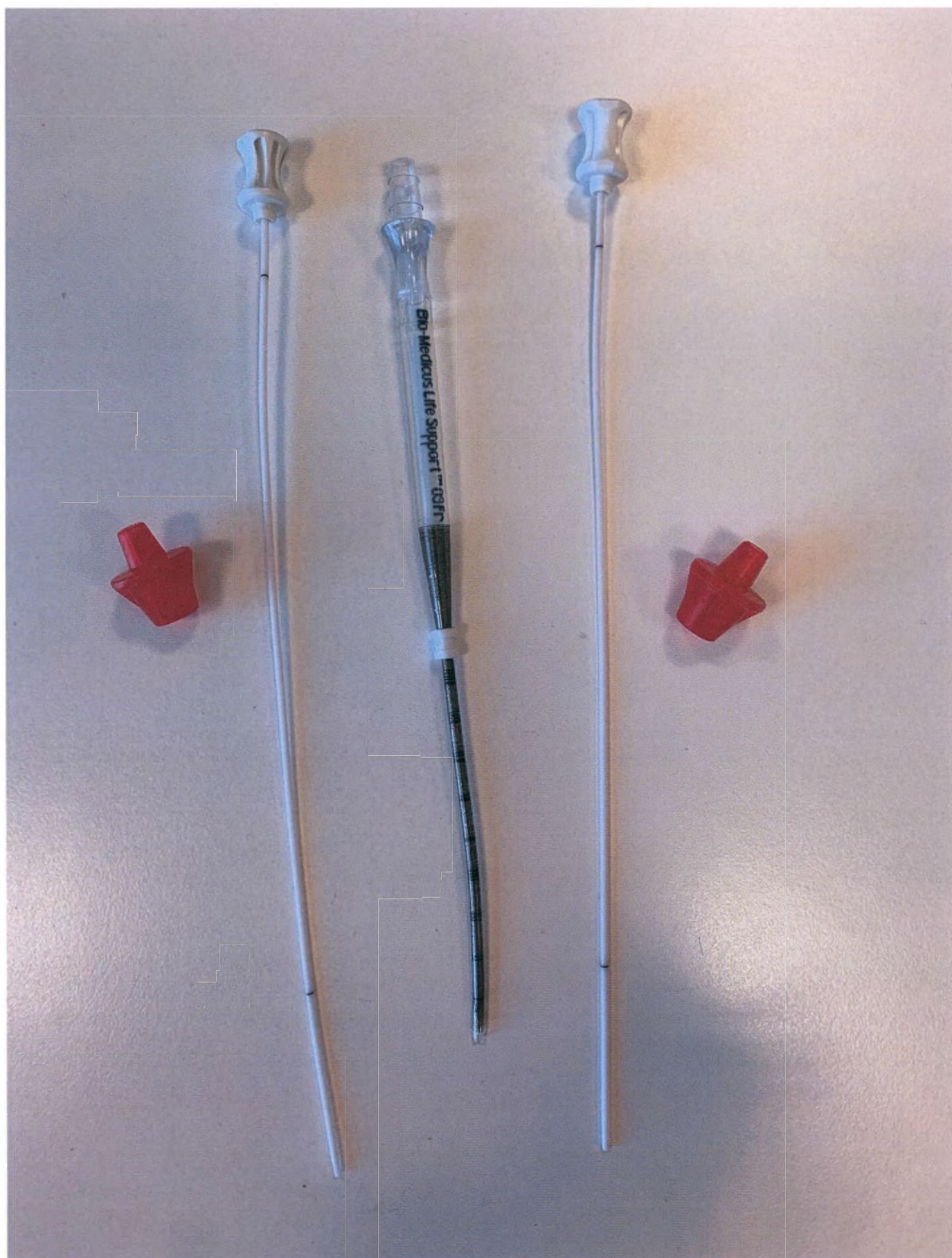
Рисунок 14. Катетер возвратный и интродьюсеры Bio-Medicus Life Support, длина катетера 10 см, наружный диаметр катетера 9 Fr (3,10 мм): Катетер, Интродьюсер с цельным коническим кончиком, Интродьюсер для использования с проводником, Колпачок гемостатический, Кольцо шовное рентгеноконтрастное регулируемое
