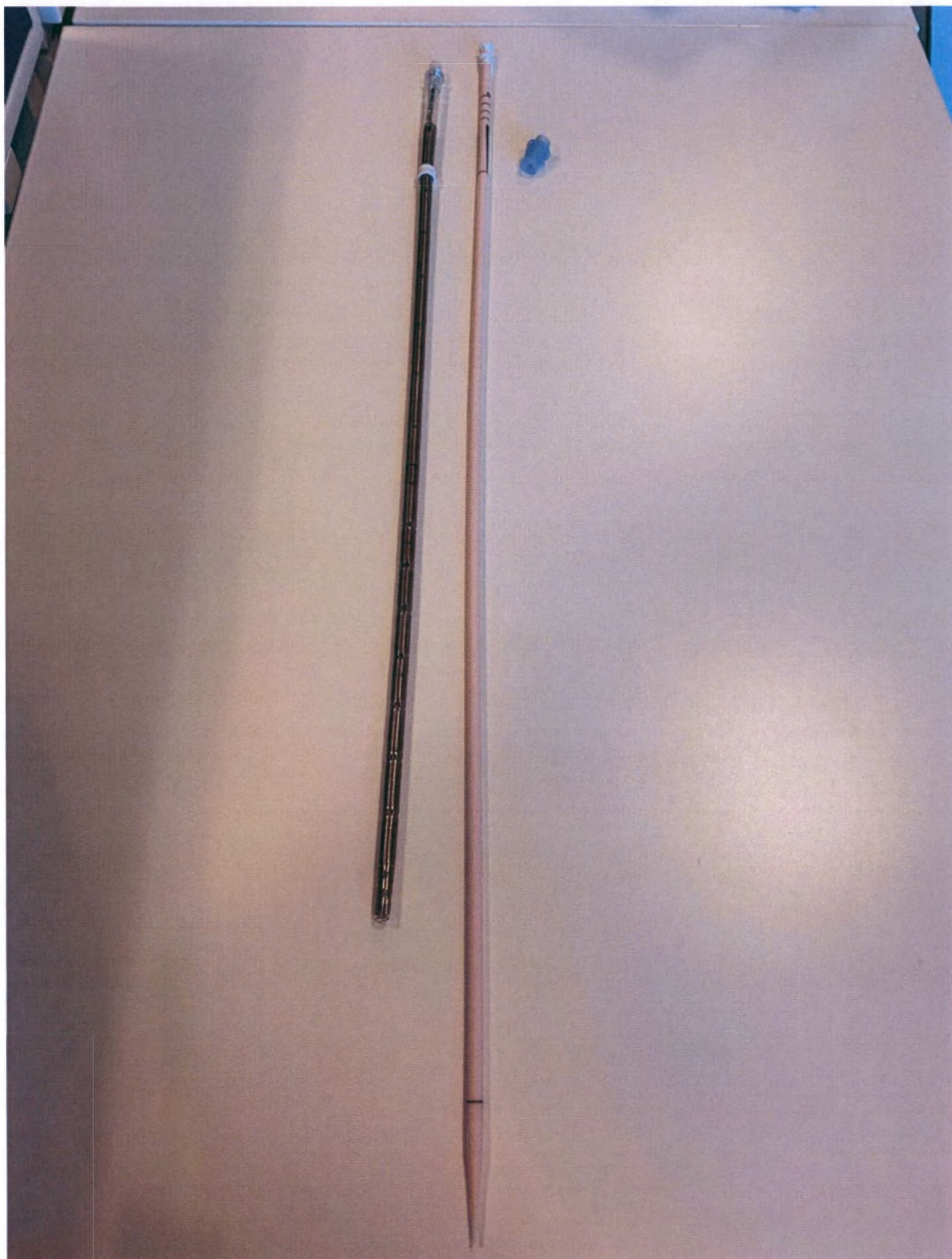
Рисунок 58. Катетер дренажный и интродьюсер Bio-Medicus Life Support, длина катетера 61 см, наружный диаметр катетера 29 Fr (9,67 мм): Катетер, Интродьюсер для использования с проводником, Колпачок гемостатический, Кольцо шовное рентгеноконтрастное регулируемое
