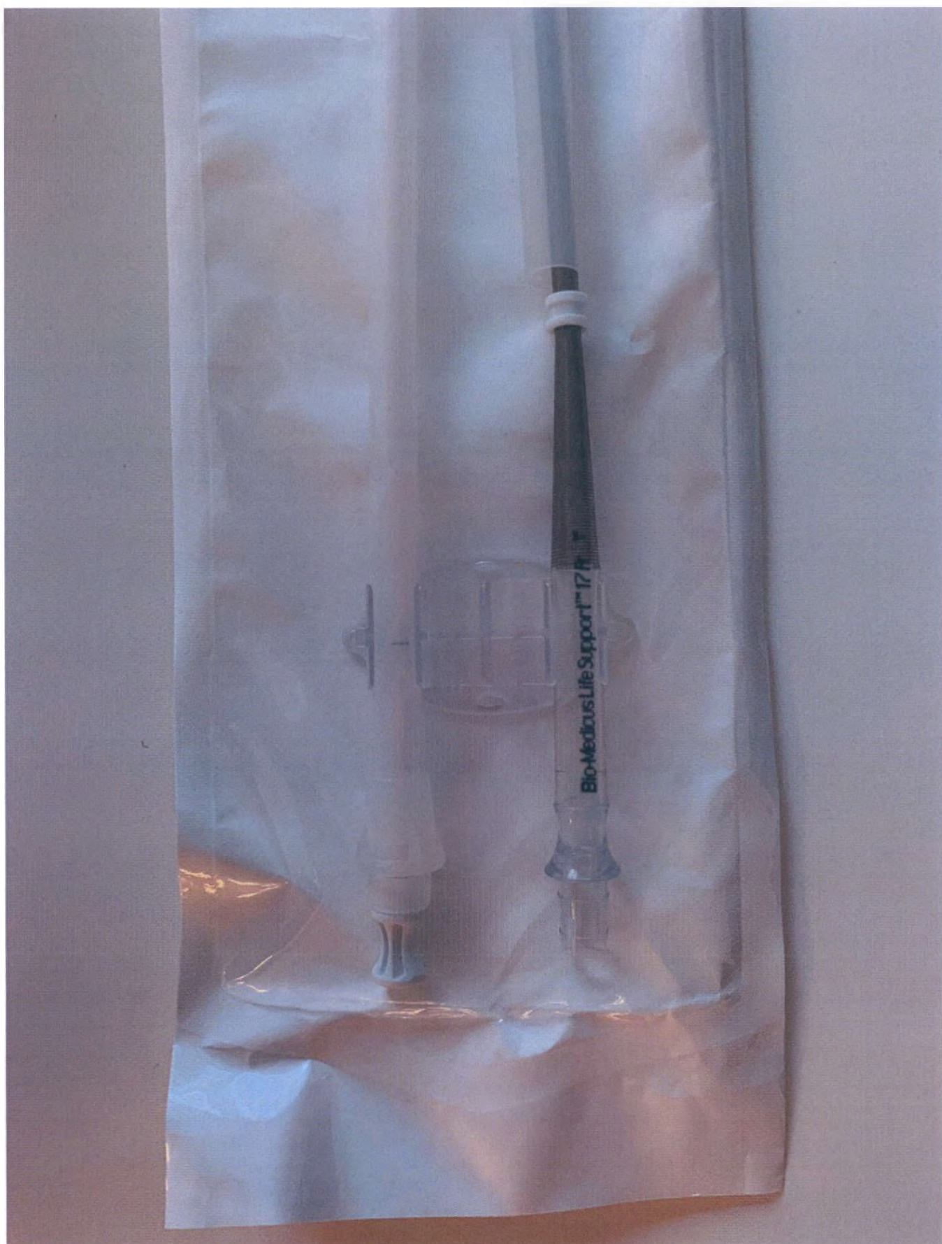
Рисунок 64. Катетер и интродьюсер Bio-Medicus Life Support, длина катетера 50 см, наружный диаметр катетера 17 Fr (5,72 мм), в составе: Катетер, Интродьюсер для использования с проводником, Колпачок гемостатический, Кольцо шовное рентгеноконтрастное регулируемое, Зажим для фиксации катетера
