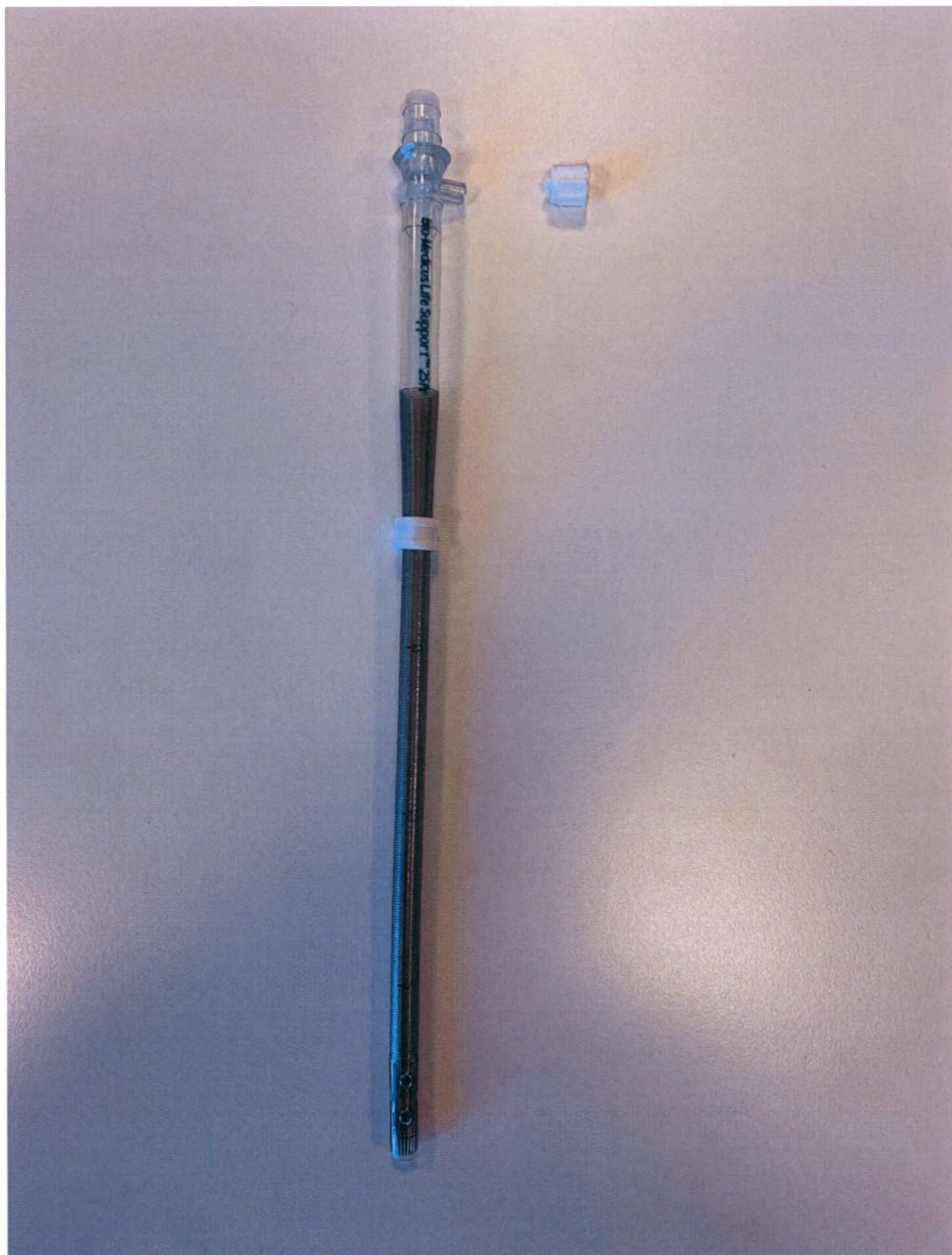
Рисунок 27. Катетер и интродьюсер Bio-Medicus Life Support, длина катетера 18 см, наружный диаметр катетера 25 Fr (8,36 мм): Катетер
