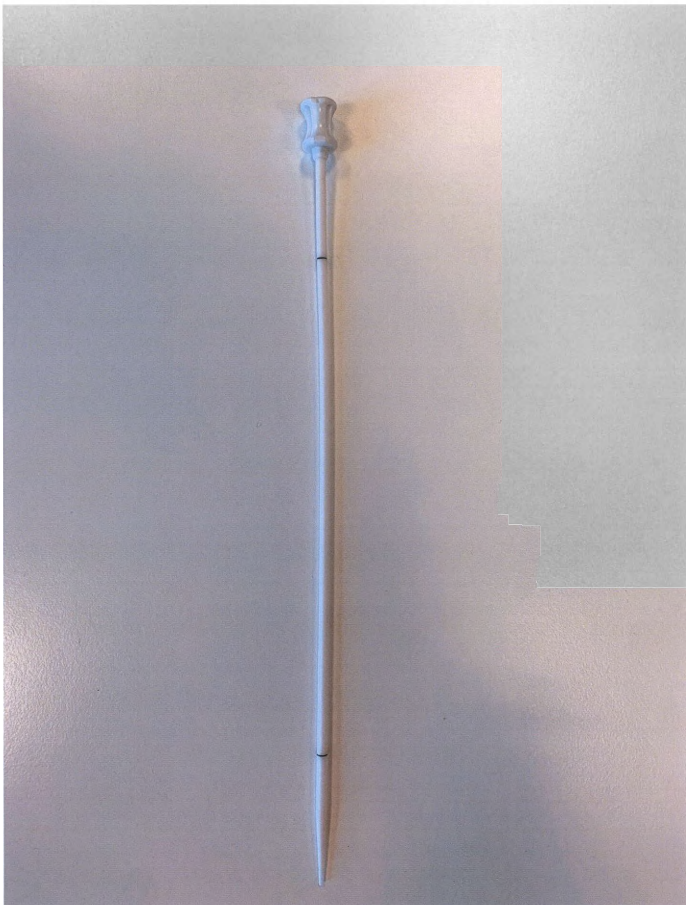
Рисунок 7. Катетер дренажный и интродьюсеры Bio-Medicus Life Support, длина катетера 11,5 см, наружный диаметр катетера 15 Fr (5,05 мм): Интродьюсер с цельным коническим кончиком
