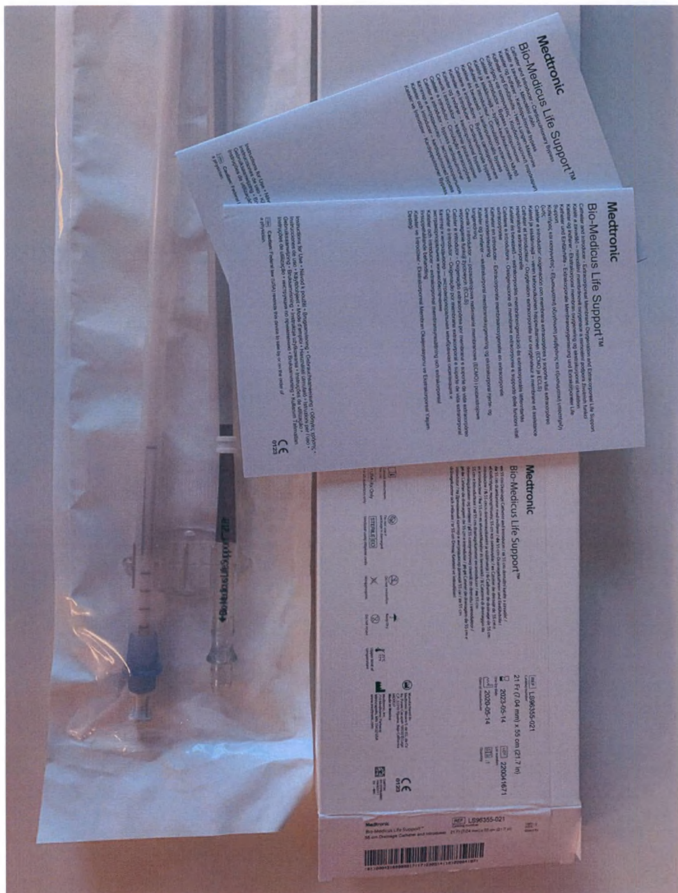
Рисунок 73. Катетер дренажный и интродьюсер Bio-Medicus Life Support, длина катетера 55 см, наружный диаметр катетера 21 Fr (7,04 мм), в составе: Катетер, Интродьюсер для использования с проводником, Колпачок гемостатический, Кольцо шовное рентгеноконтрастное регулируемое, Жажим для фиксации катетера
