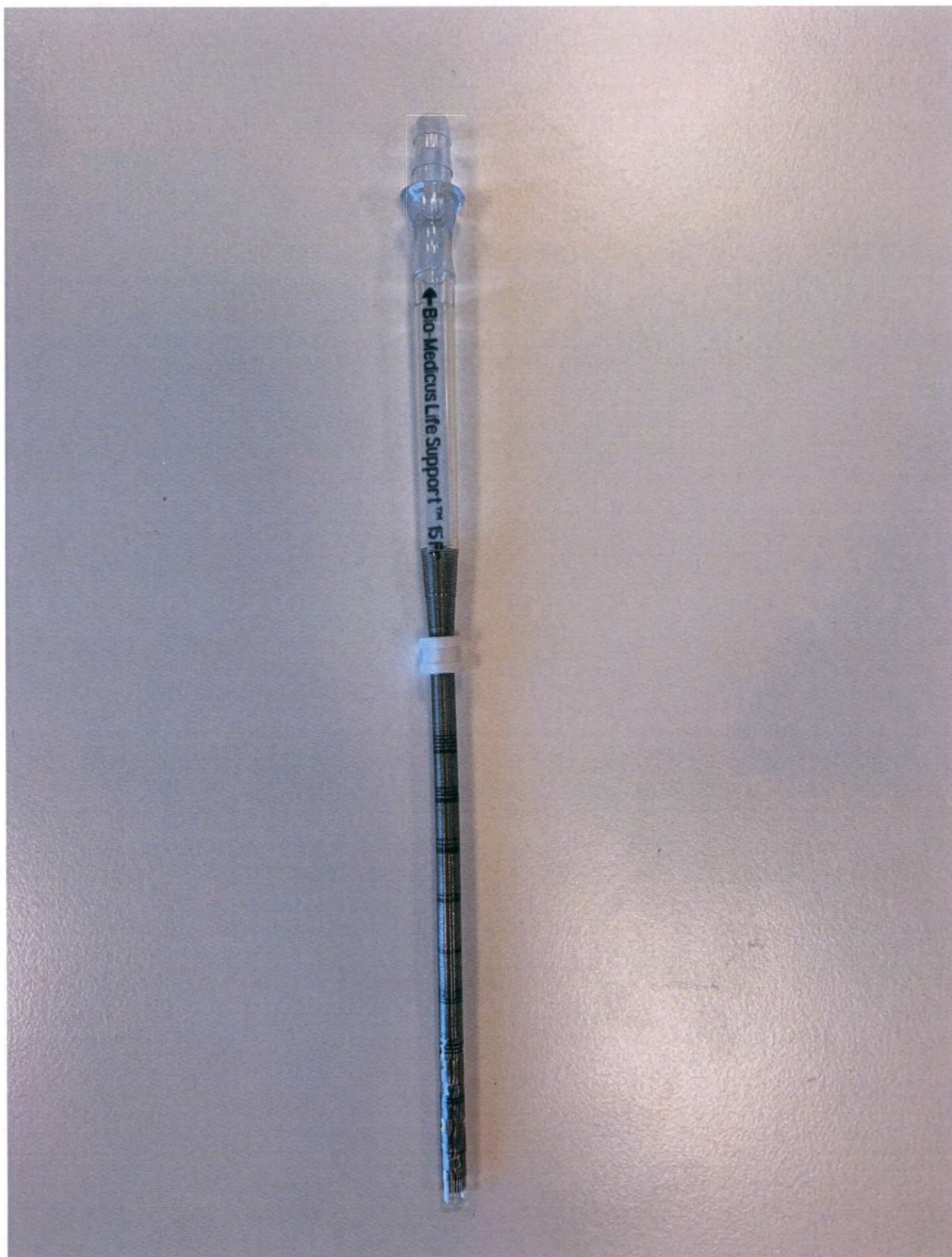
Рисунок 6. Катетер дренажный и интродьюсеры Bio-Medicus Life Support, длина катетера 11,5 см, наружный диаметр катетера 15 Fr (5,05 мм): Катетер
