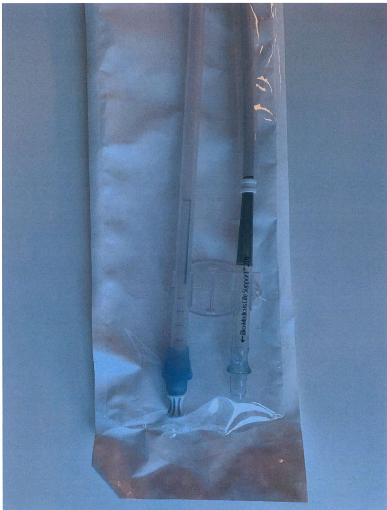
Рисунок 44. Рисунок 43. Катетер дренажный и интродьюсер Bio-Medicus Life Support, длина катетера 38 см, наружный диаметр катетера 21 Fr (7,04 мм), в составе: Катетер, Интродьюсер для использования с проводником, Колпачок гемостатический, Кольцо шовное рентгеноконтрастное регулируемое, Зажим для фиксации катетера
