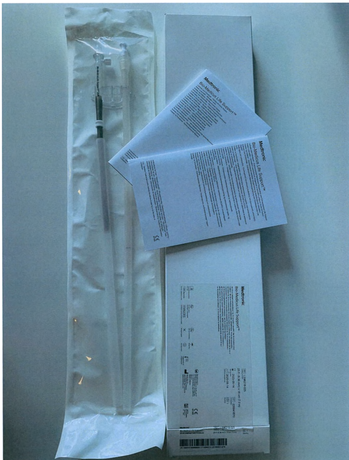
Рисунок 19. Катетер и интродьюсер Bio-Medicus Life Support, длина катетера 18 см, наружный диаметр катетера 25 Fr (8,36 мм), в составе: Катетер, Интродьюсер для использования с проводником, Колпачок гемостатический, Кольцо шовное рентгеноконтрастное регулируемое, Зажим для фиксации катетера, Инструкции по применению
