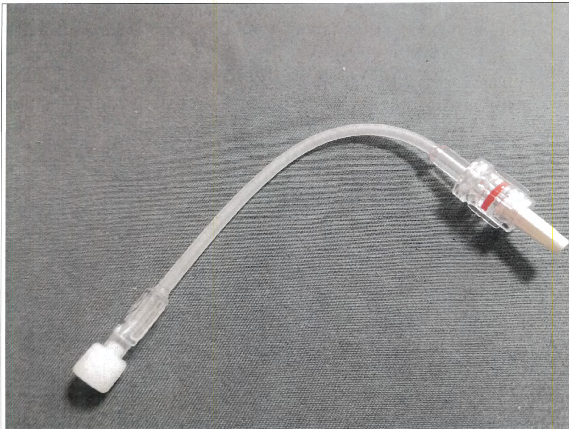
Рис. 21. Линия соединительная высокого давления, длина 10 см, 15 см, 30 см, 35 см, 50 см, 60 см, 70 см, 75 см, 90 см, 100 см, 120 см по ТУ 32.50.13-005-15624048-2021
