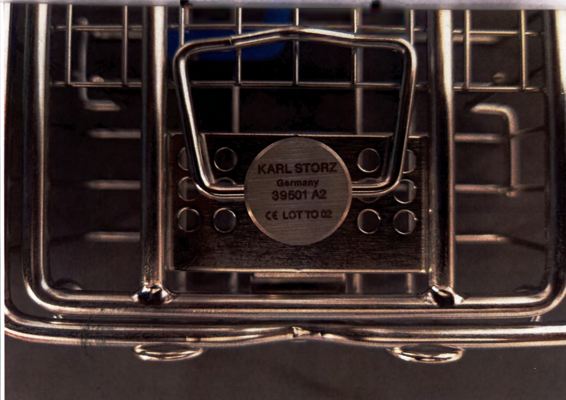
Рис. 29. Контейнер проволочный для дезинфекции/стерилизации/хранения, размеры: 352 x 125 x 54 мм
