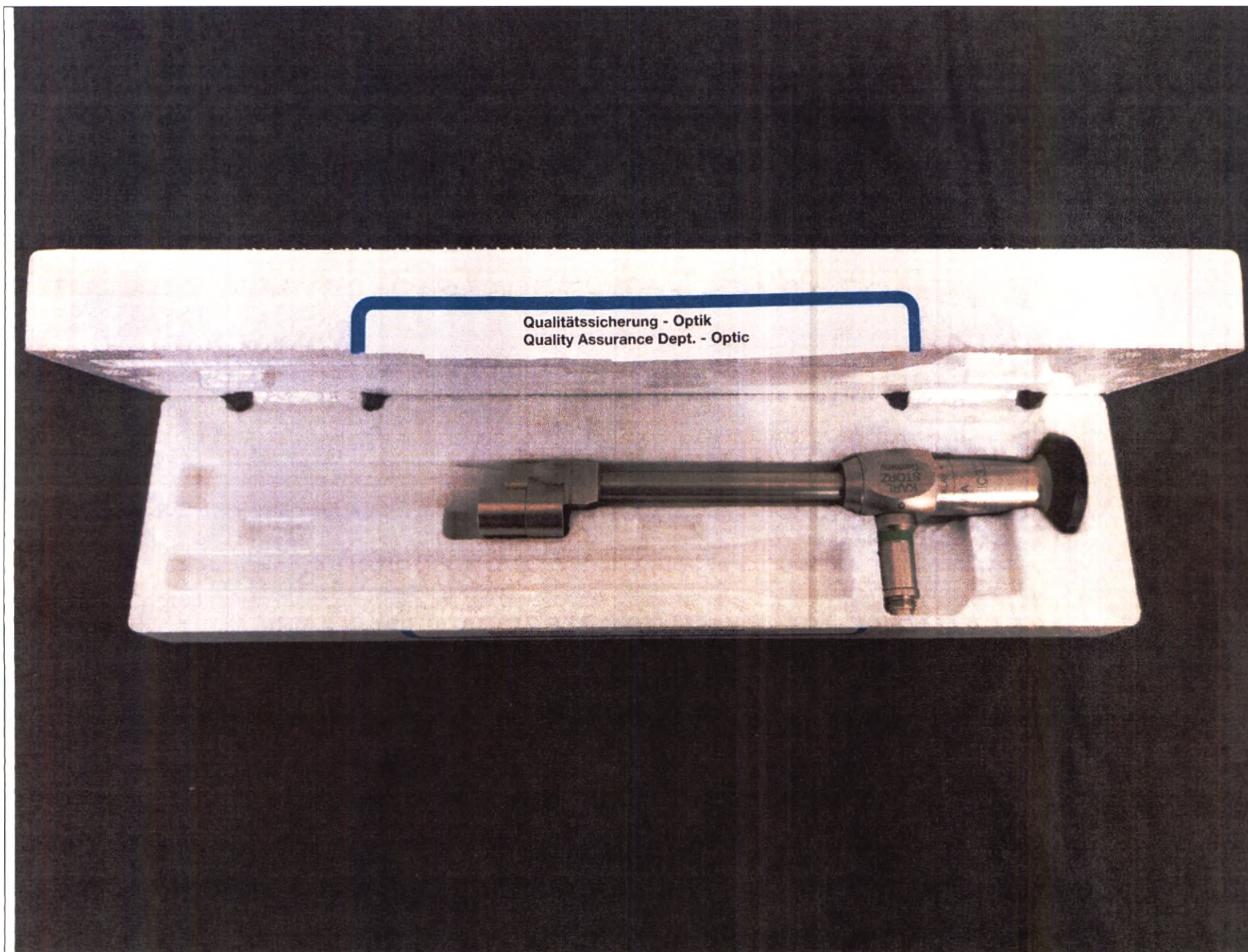
Рис. 19. Экзоскоп VITOM II NIR/ ICG, направление наблюдения 0°, длина 18 см.
