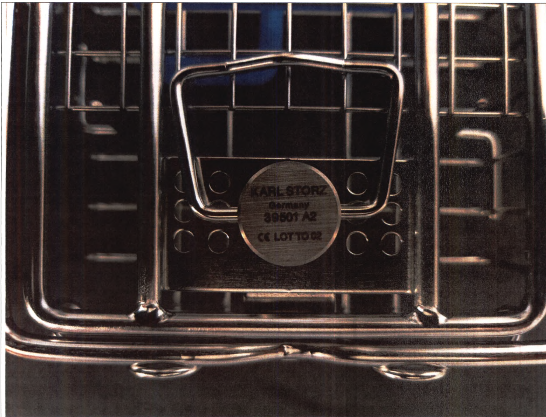
Рис. 33. Контейнер проволочный для дезинфекции/стерилизации/хранения, размеры: 352 x 125 x 54 мм
