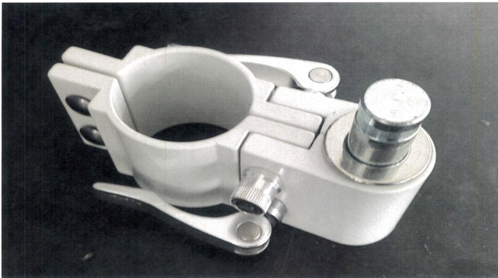
Крепление фиксирующее (Арт. RL10IA-ZR010)
