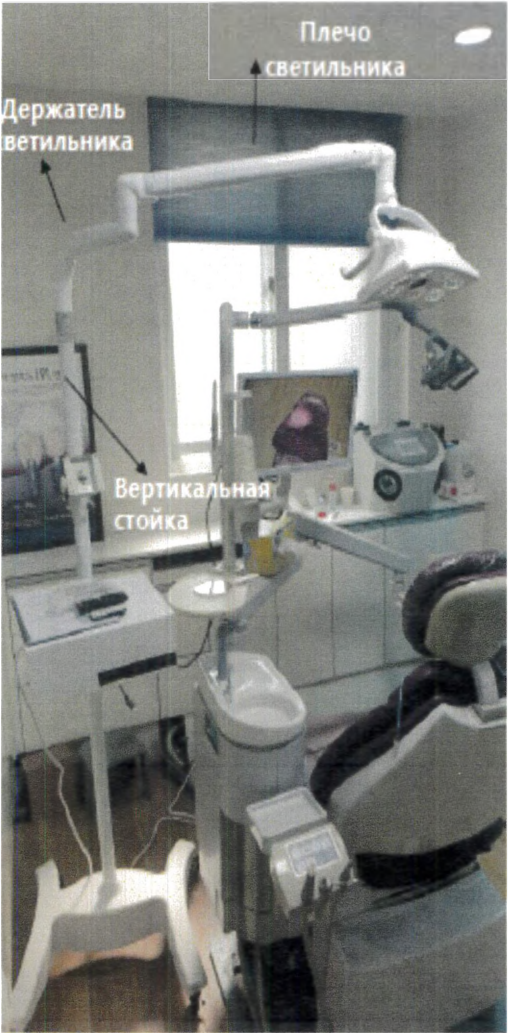
Крепление мобильное (Арт. RL10IA-CC020)
