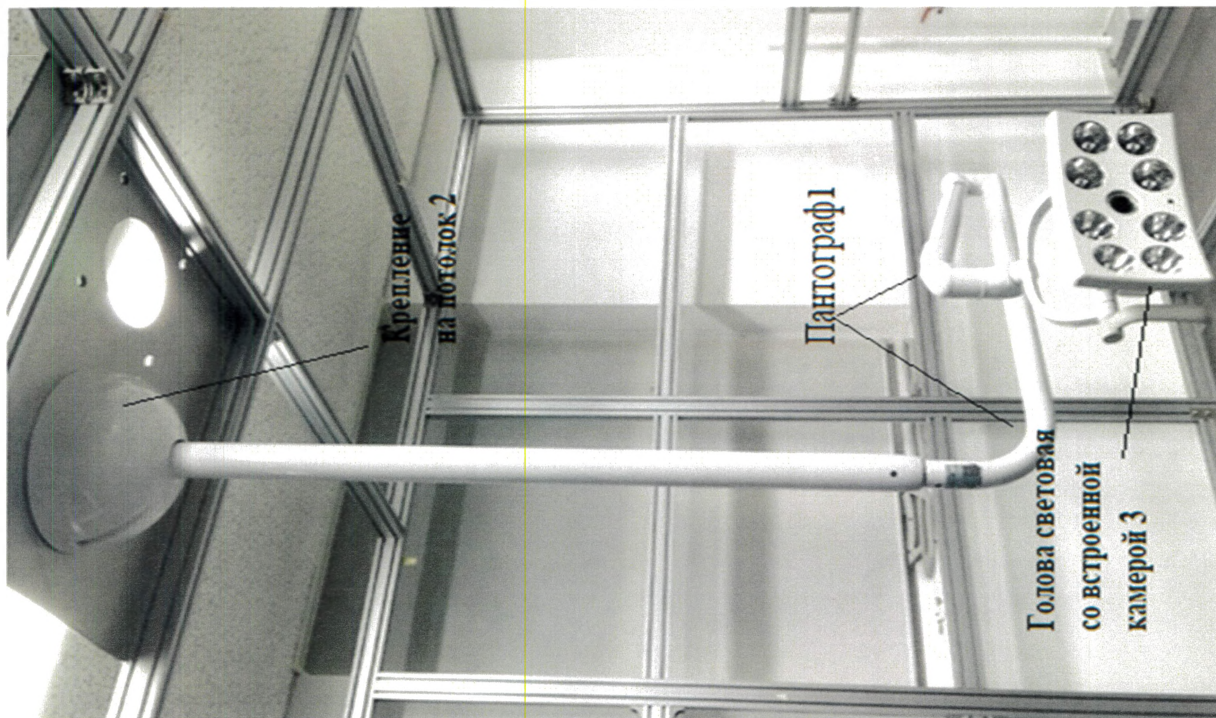
Светильник стоматологический Luvis C500, вариант исполнения C50-E2M1B1, крепление на потолок
