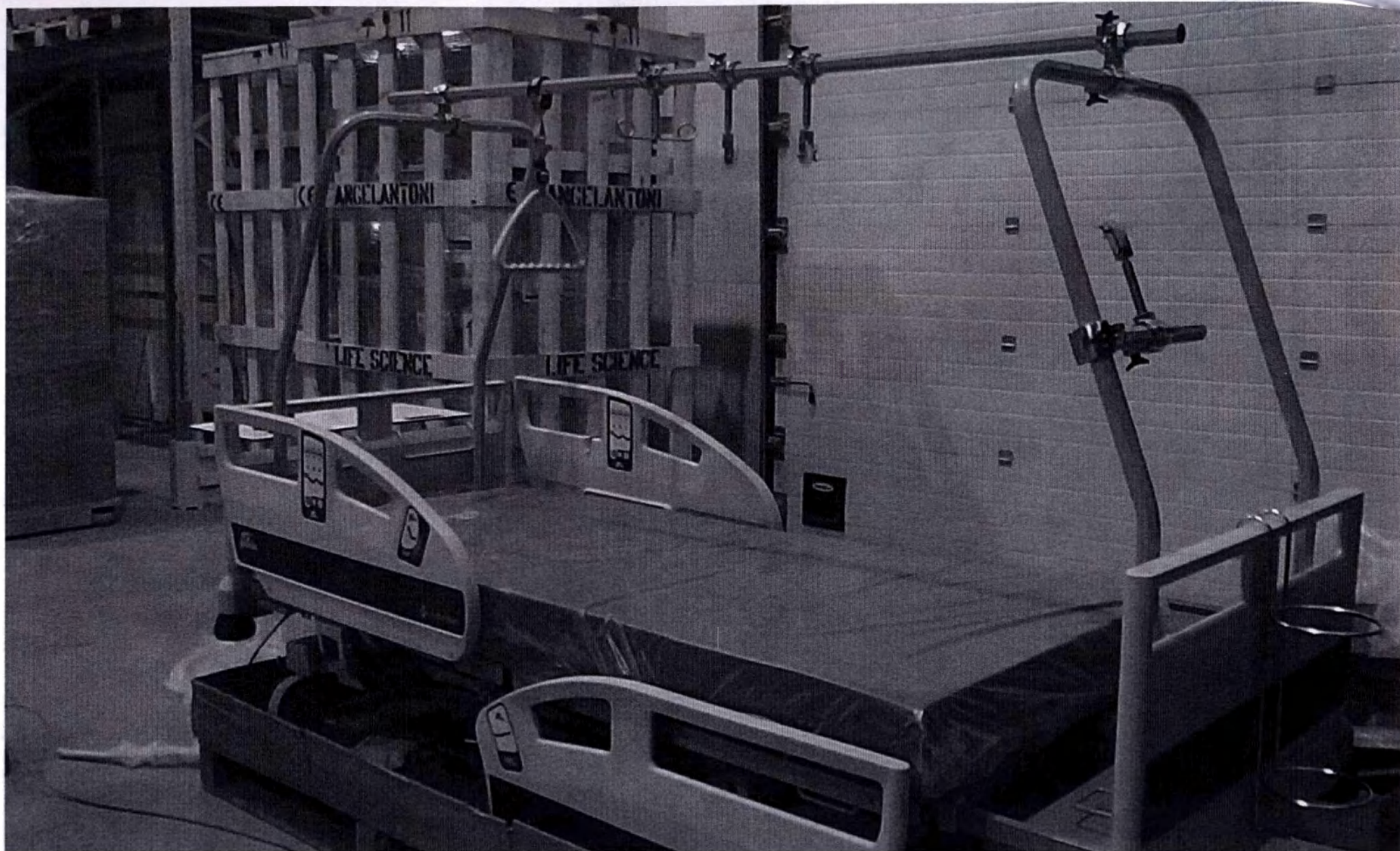
Рис.24 Тракционная рама (Рама Балканского)
