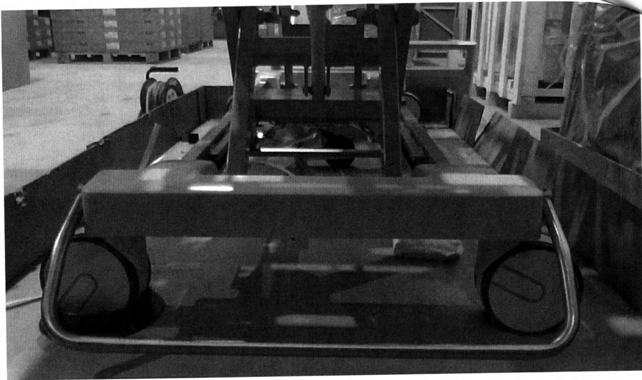
Рис. 9 Центральный тормоз, вариант исполнения многофункциональная педаль.
