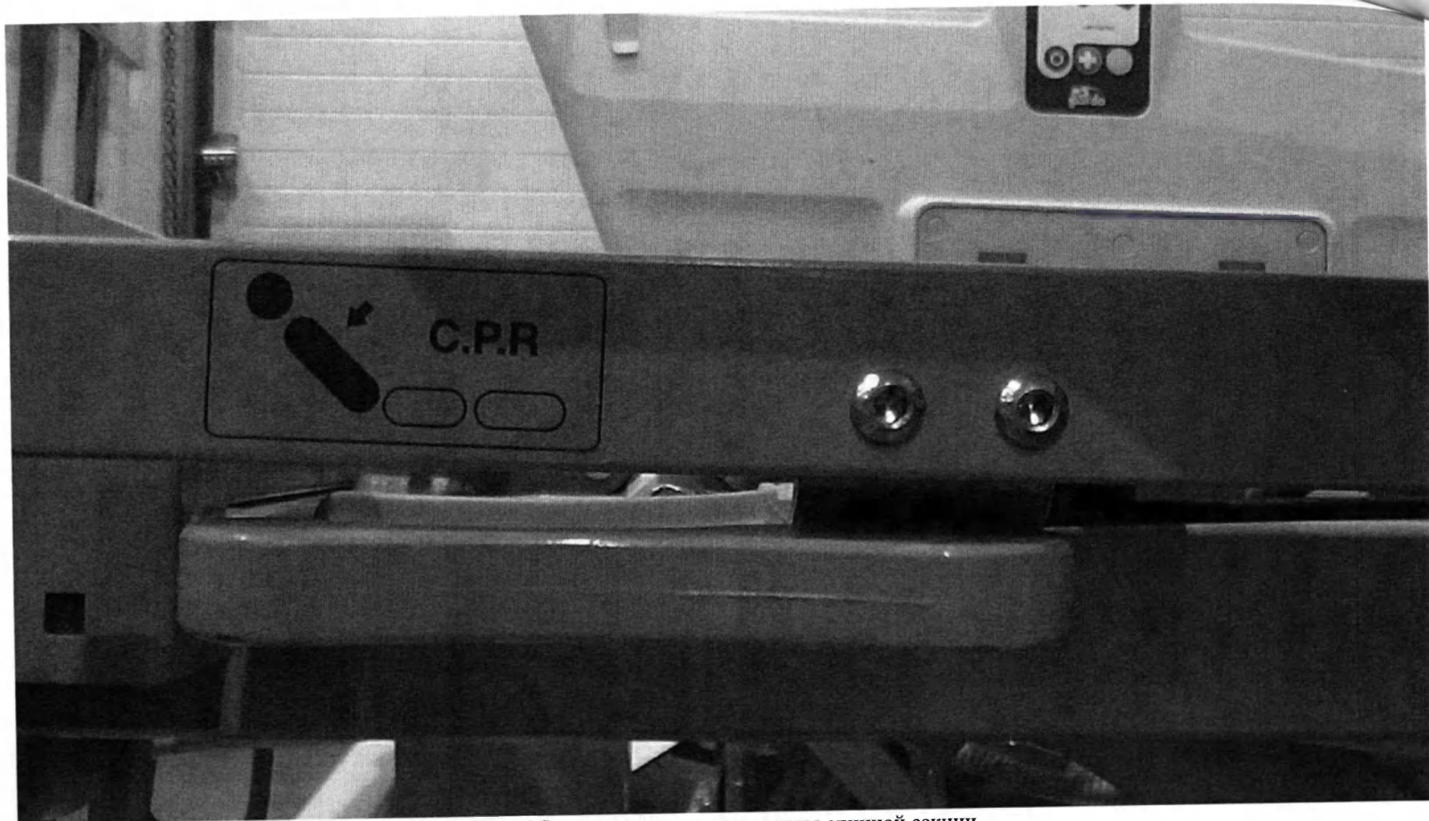
Рис.11 Рычаг экстренного опускания спинной секции
