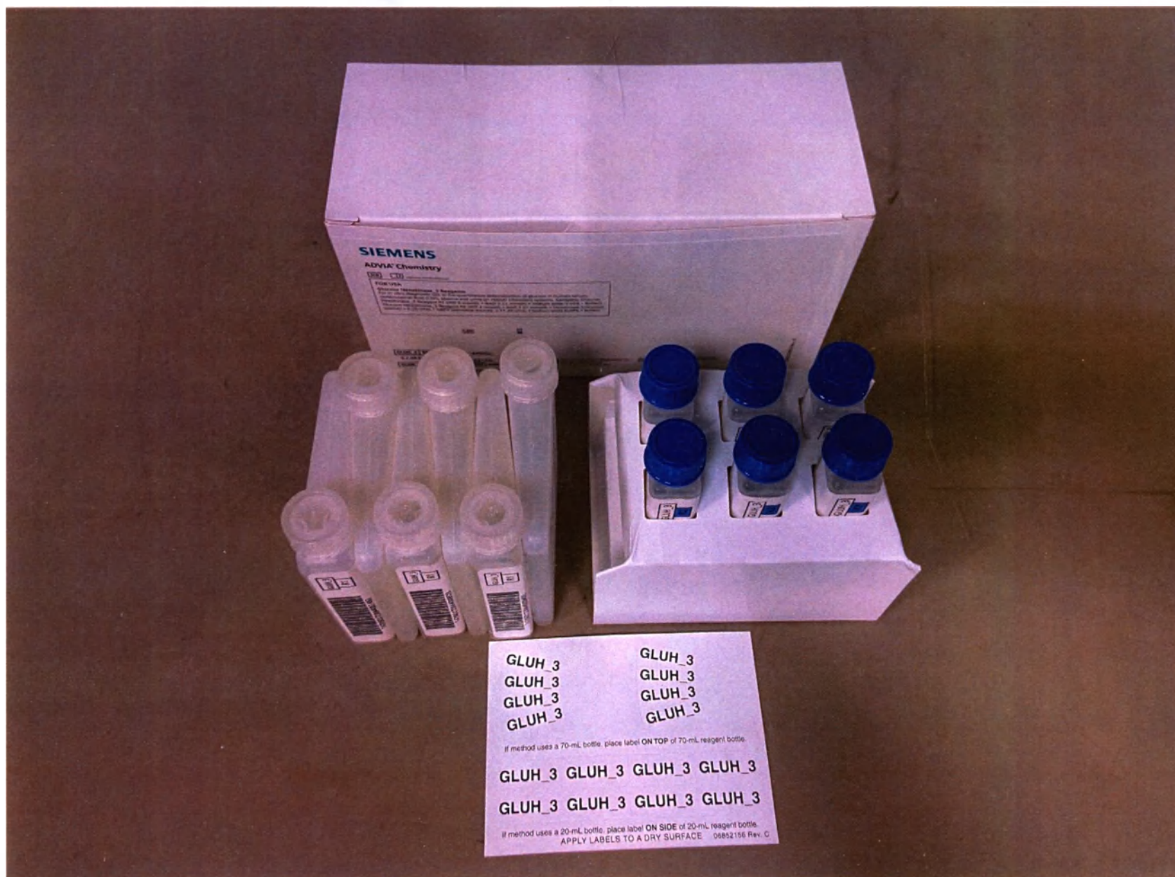
Рисунок 2. Набор реагентов для определения глюкозы гексокиназы_3 для автоматических биохимических анализаторов серии ADVIA (ADVIA Chemistry Glucose Hexokinase_3 (GLUH_3)) – общий вид медицинского изделия
