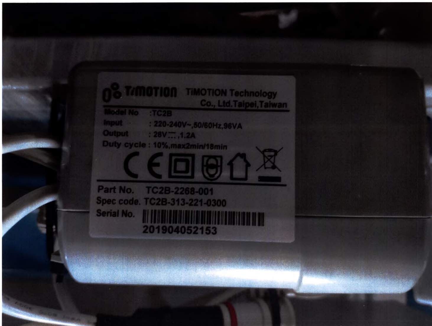
Маркировка мотора блока управления
