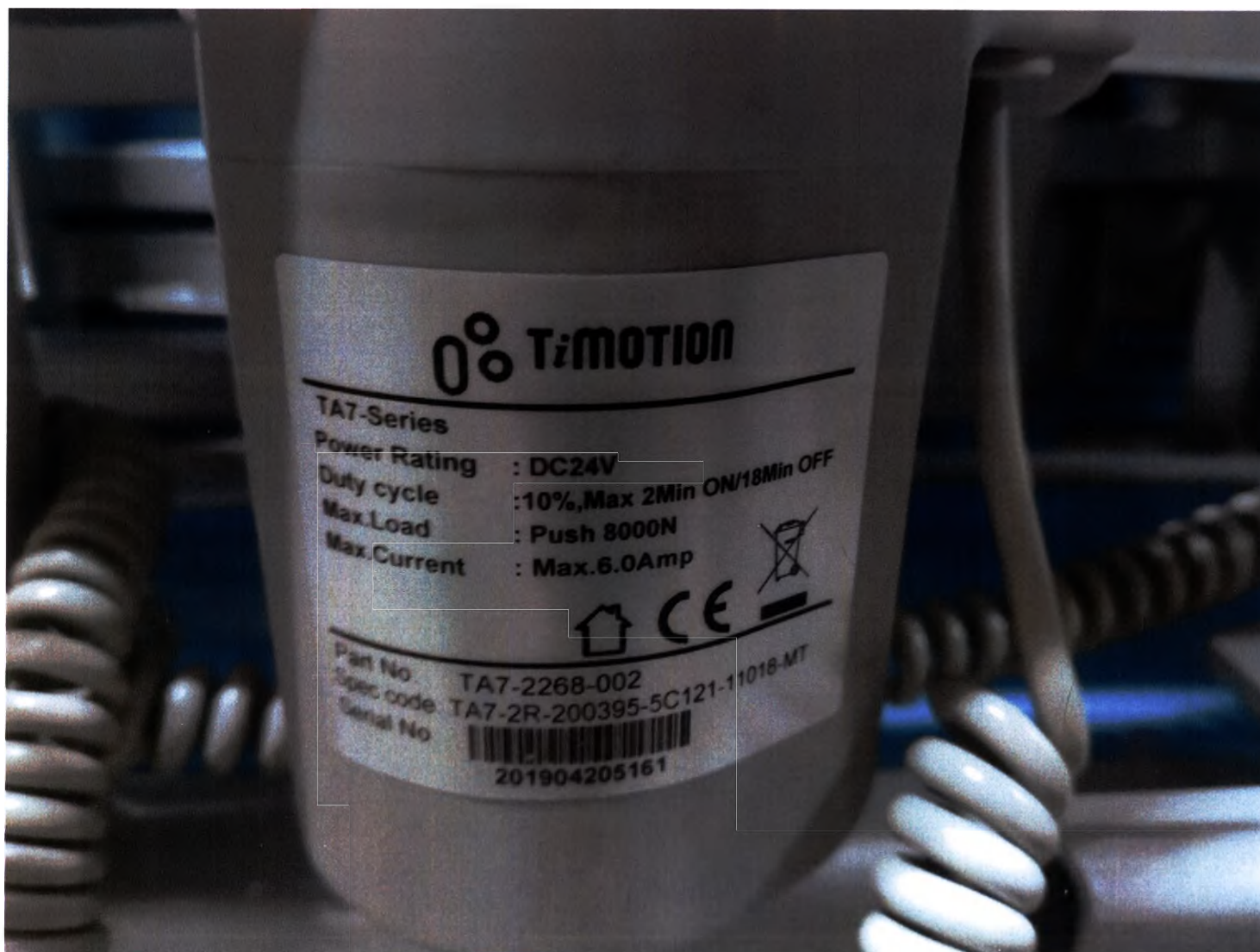
Маркировка электродвигателя
