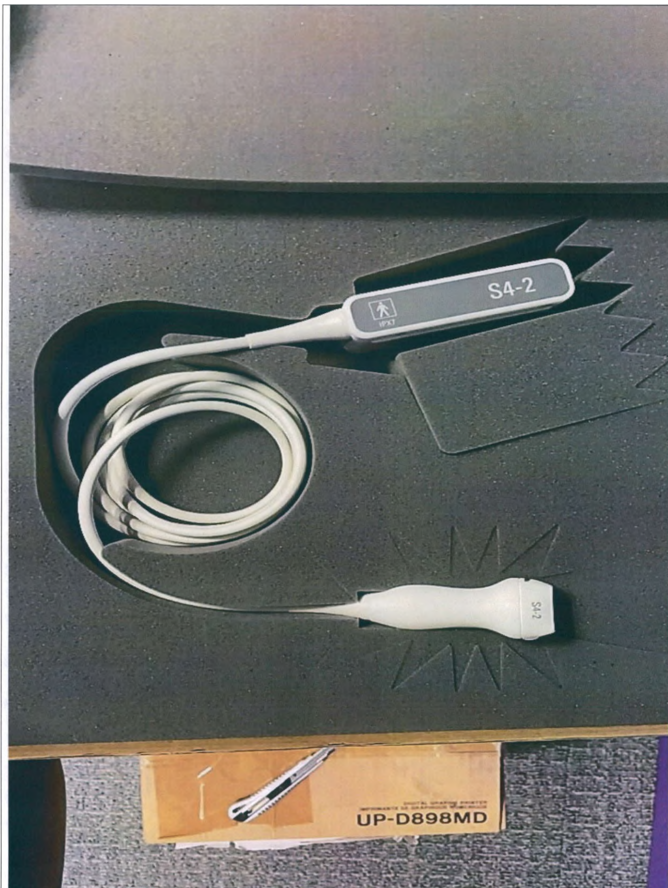
6. Датчик с фазированной (секторной) матрицей S4-2.
