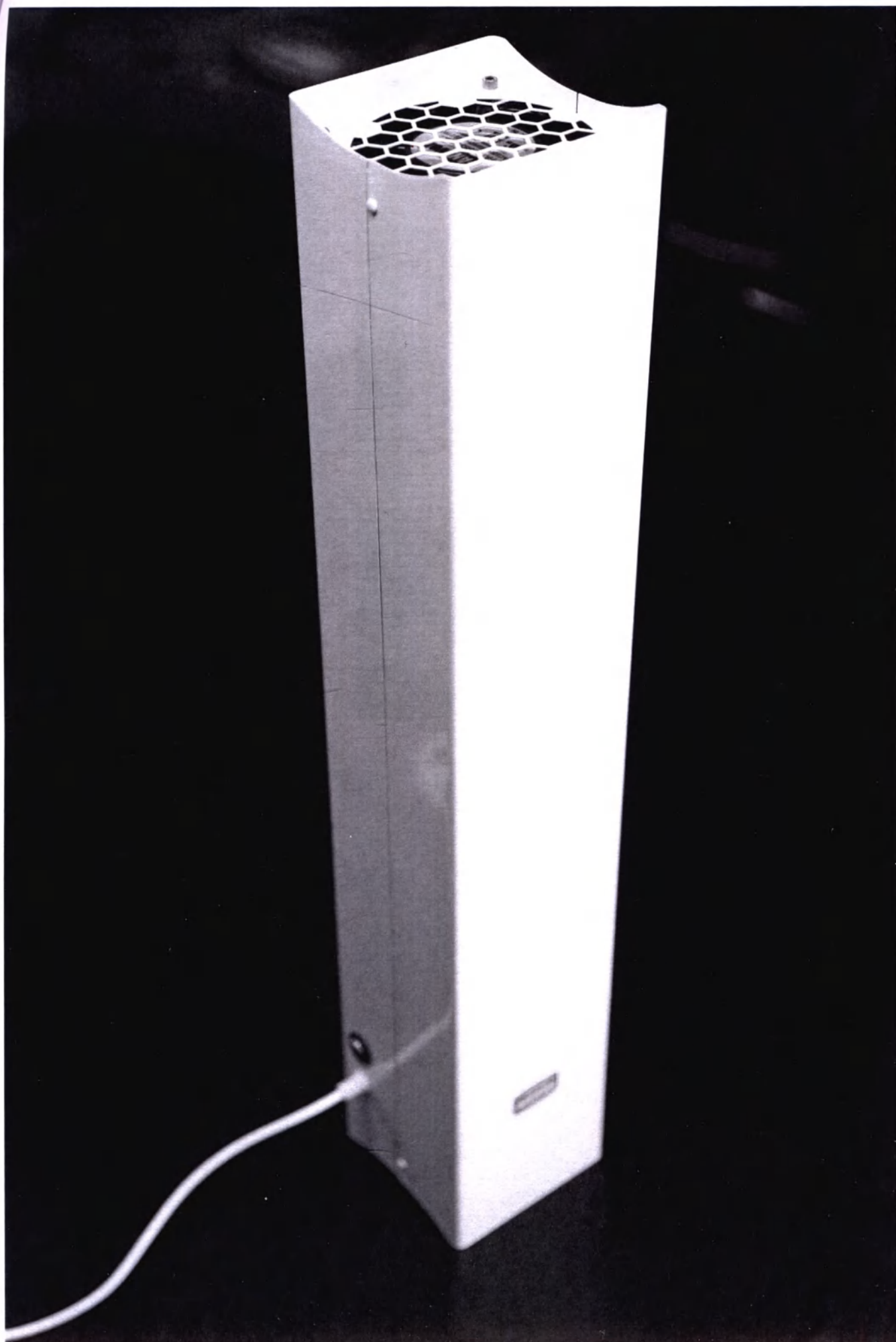
Облучатель бактерицидный ультрафиолетовый ФОТОН ОБ-06 (закрытого типа) по ТУ 32.50.50-001-76410031-2020
