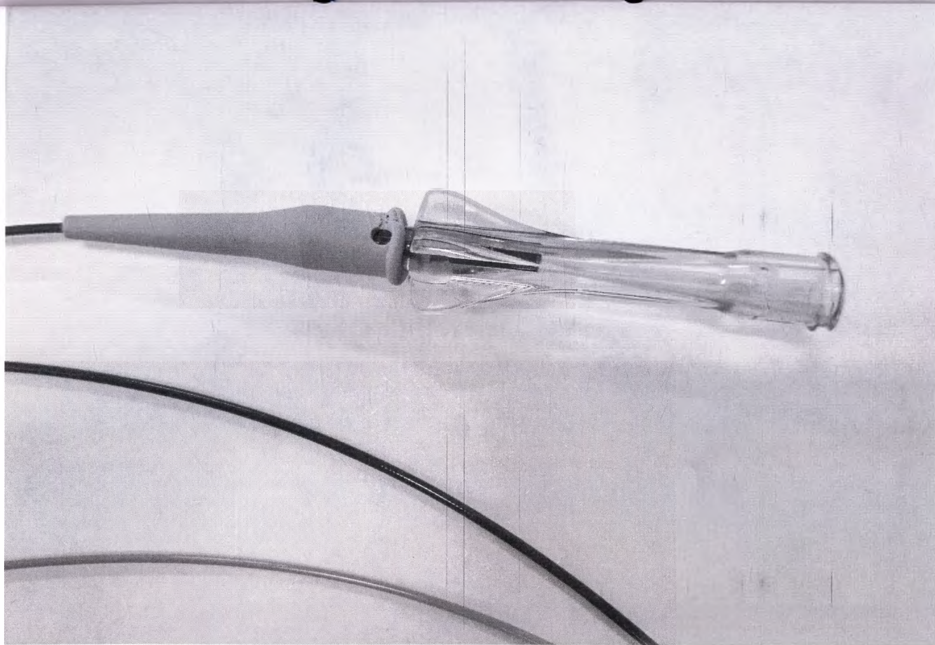
Втулка катетера Marksman
