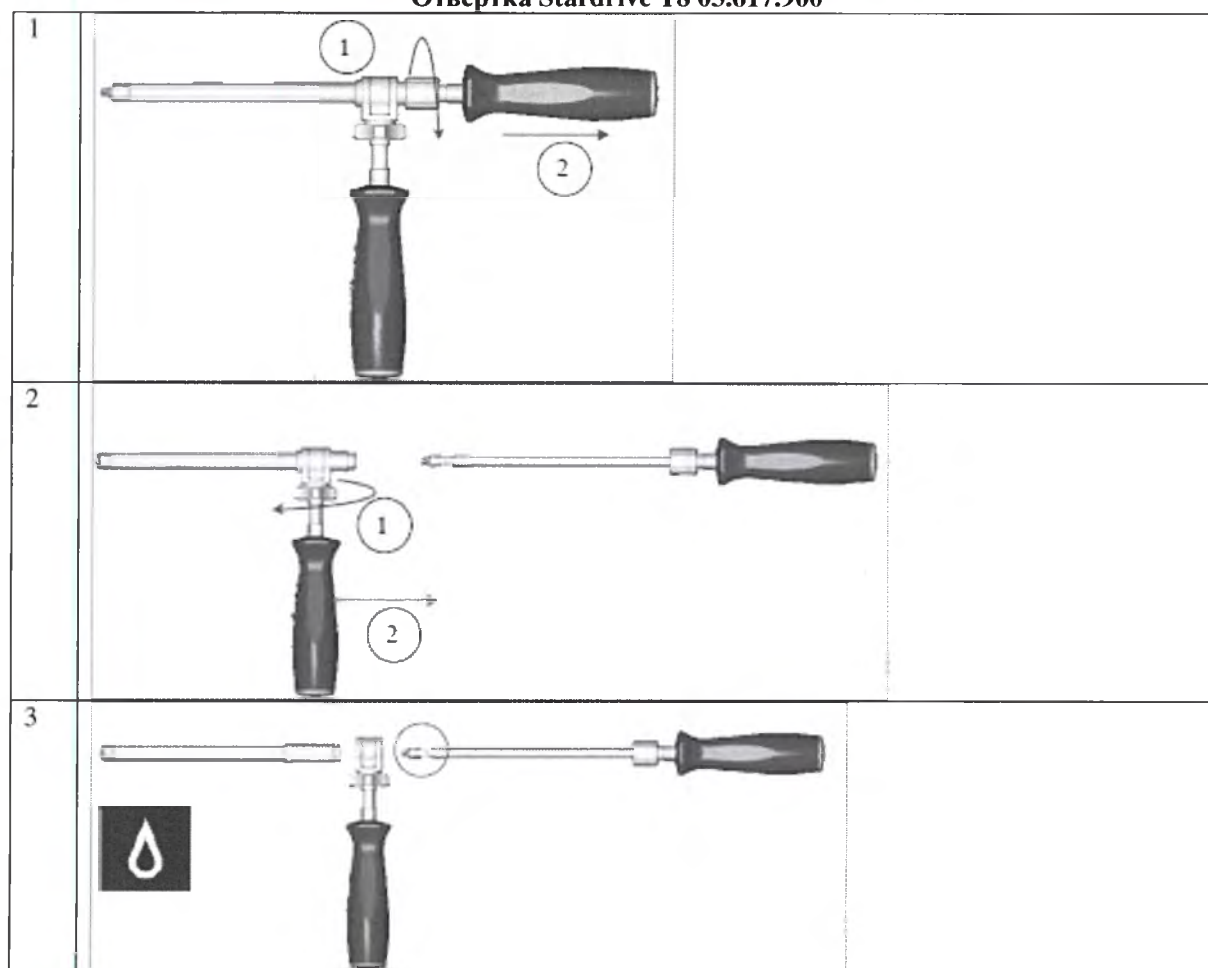
Отвертка Stardrive T8 03.617.900
