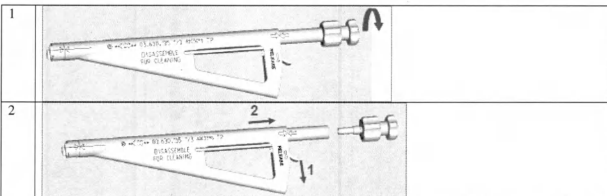
Держатель имплантата для системы FACET WEDGE 03.630.135
