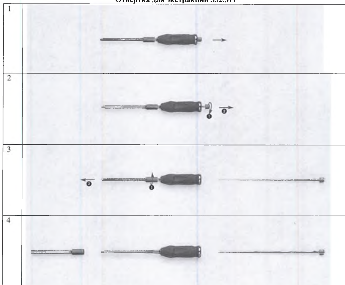
Отвертка для экстракции 352.311
