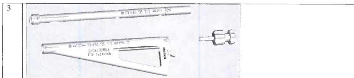
Ретрактор продольный 03.615.100, Ретрактор поперечный 03.615.002
