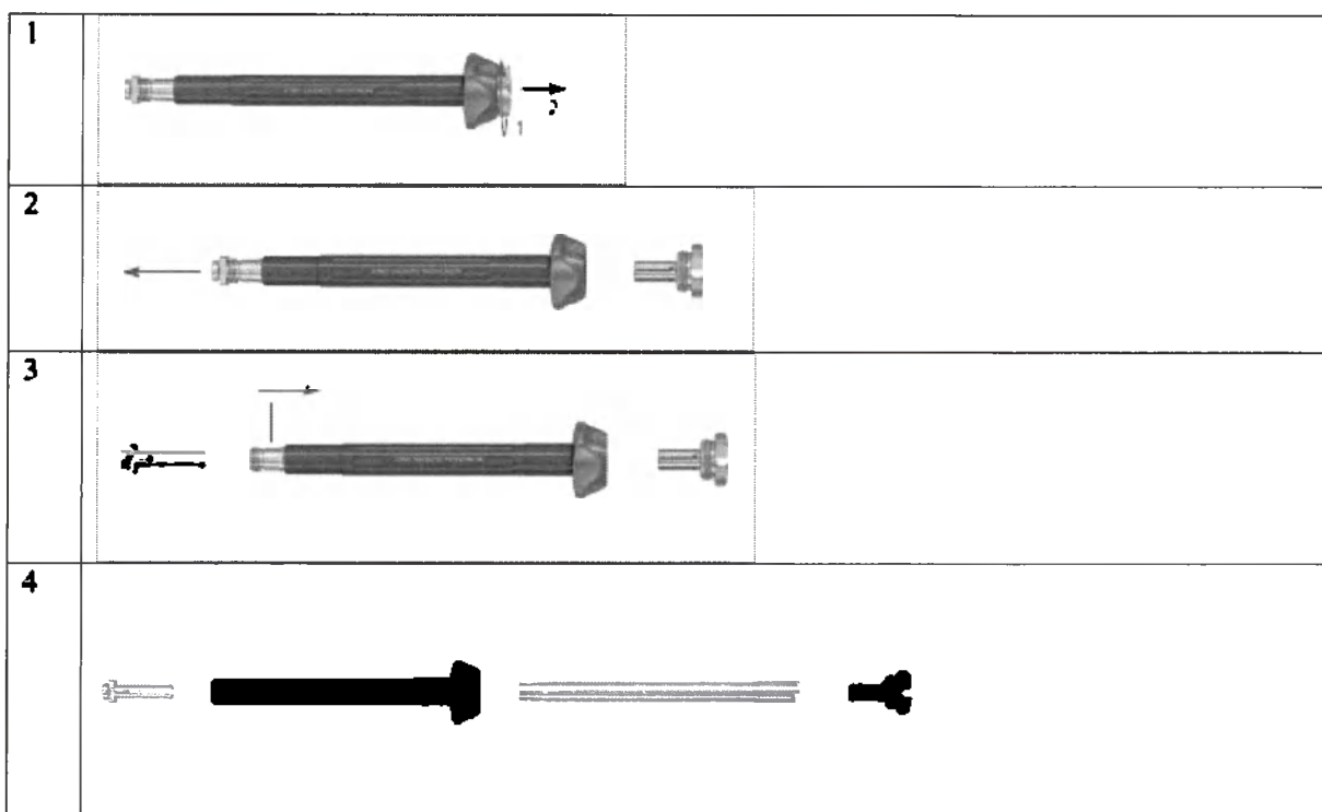
Втулка удерживающая для моноаксиальных винтов, стандартная Matrix 5,5 03.632.024
