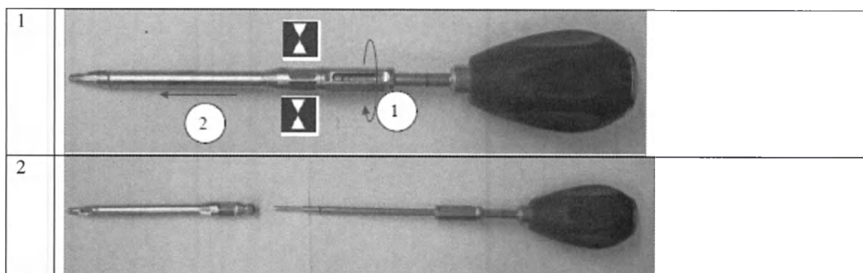
Модуль для заполнения Zero-P 03.617.984/-US, подкладка для системы Zero-P VA 03.647.984
