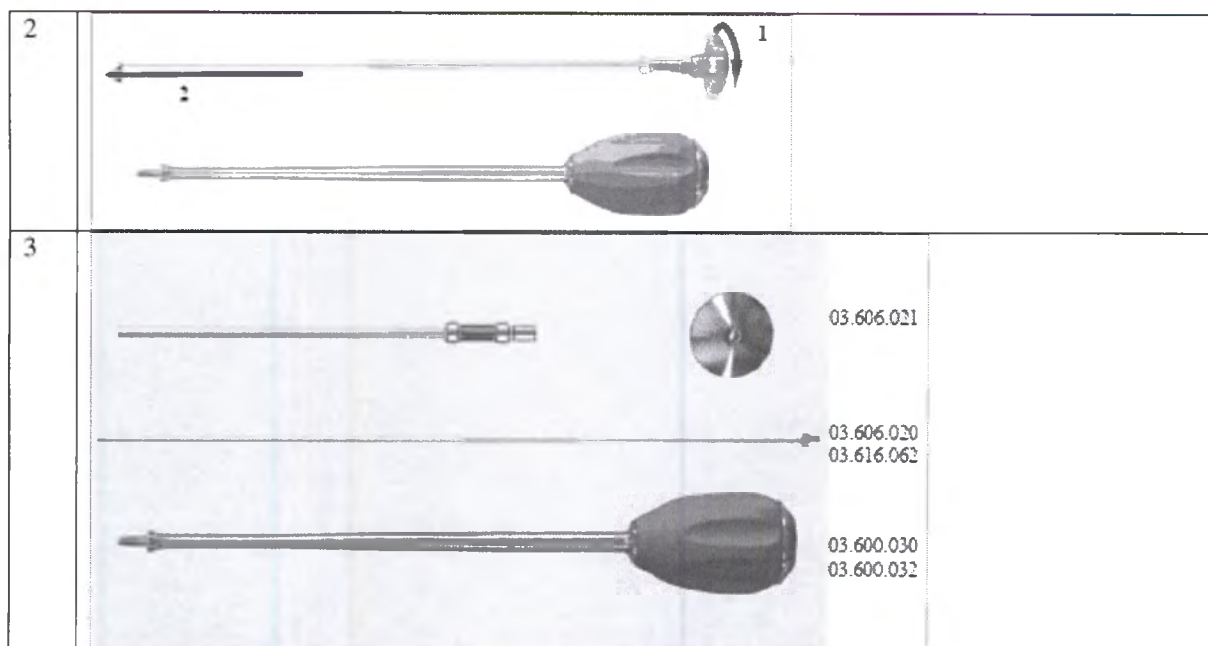
Наконечник дистрактора для головок винтов для системы Matrix 5 03.632.084
