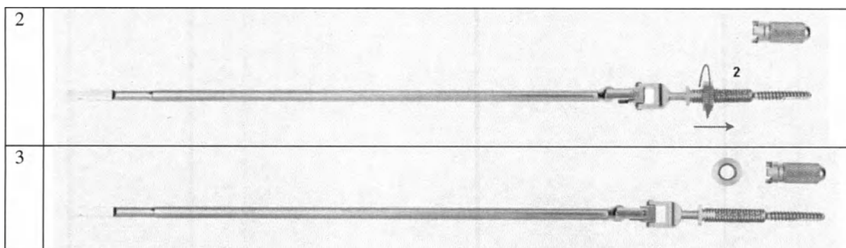
Измеритель глубины для винтов диаметром 3,5 до 4,0 мм 319.009, измеритель длины для бикортикальных винтов 387.292, измеритель для винтов, диапазон измерения диаметром 3,5–5 03.161.028
