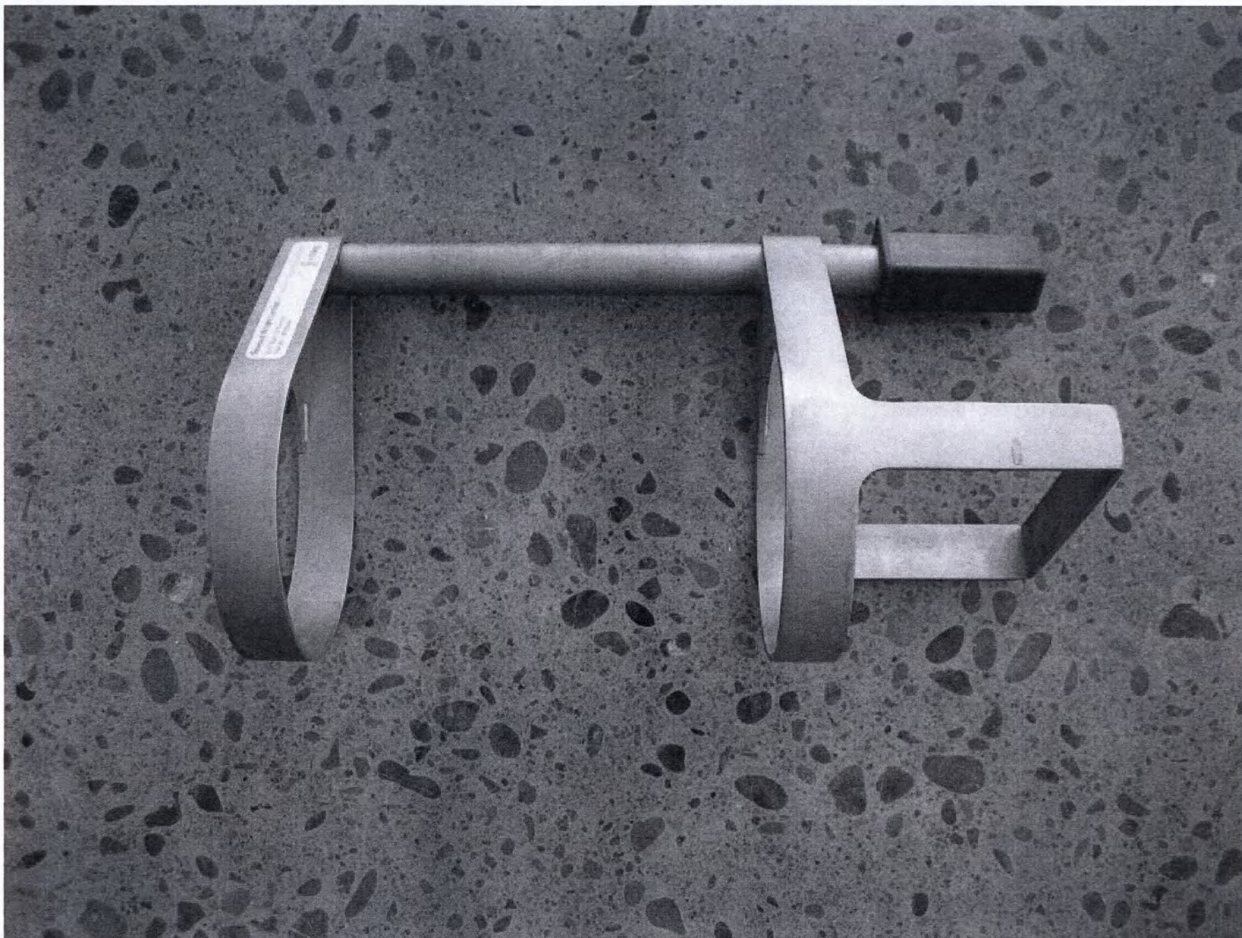
Рис. 13 Держатель для кислородного баллона размер A/C
