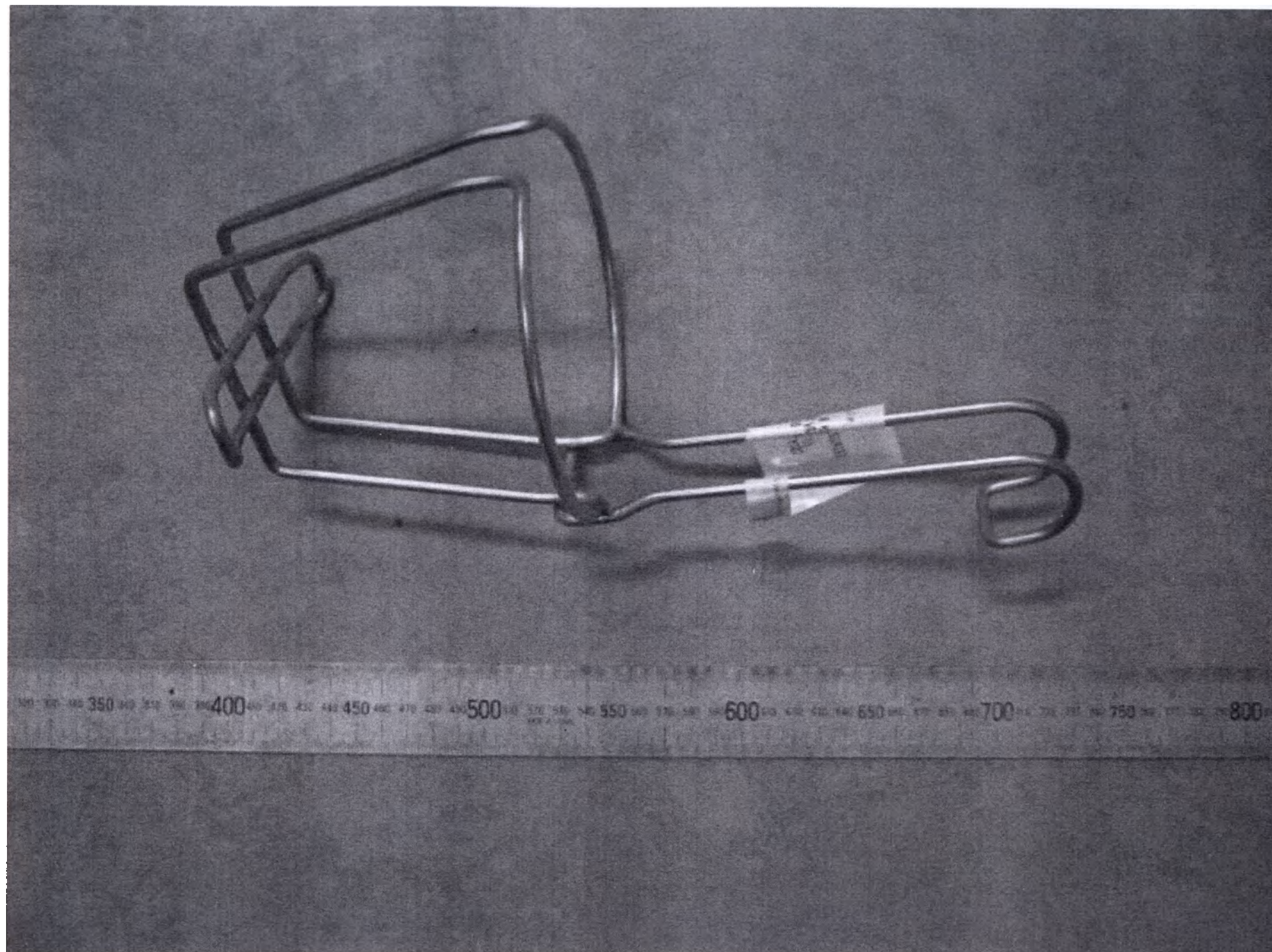
Рис. 18 Держатель мочевого катетера
