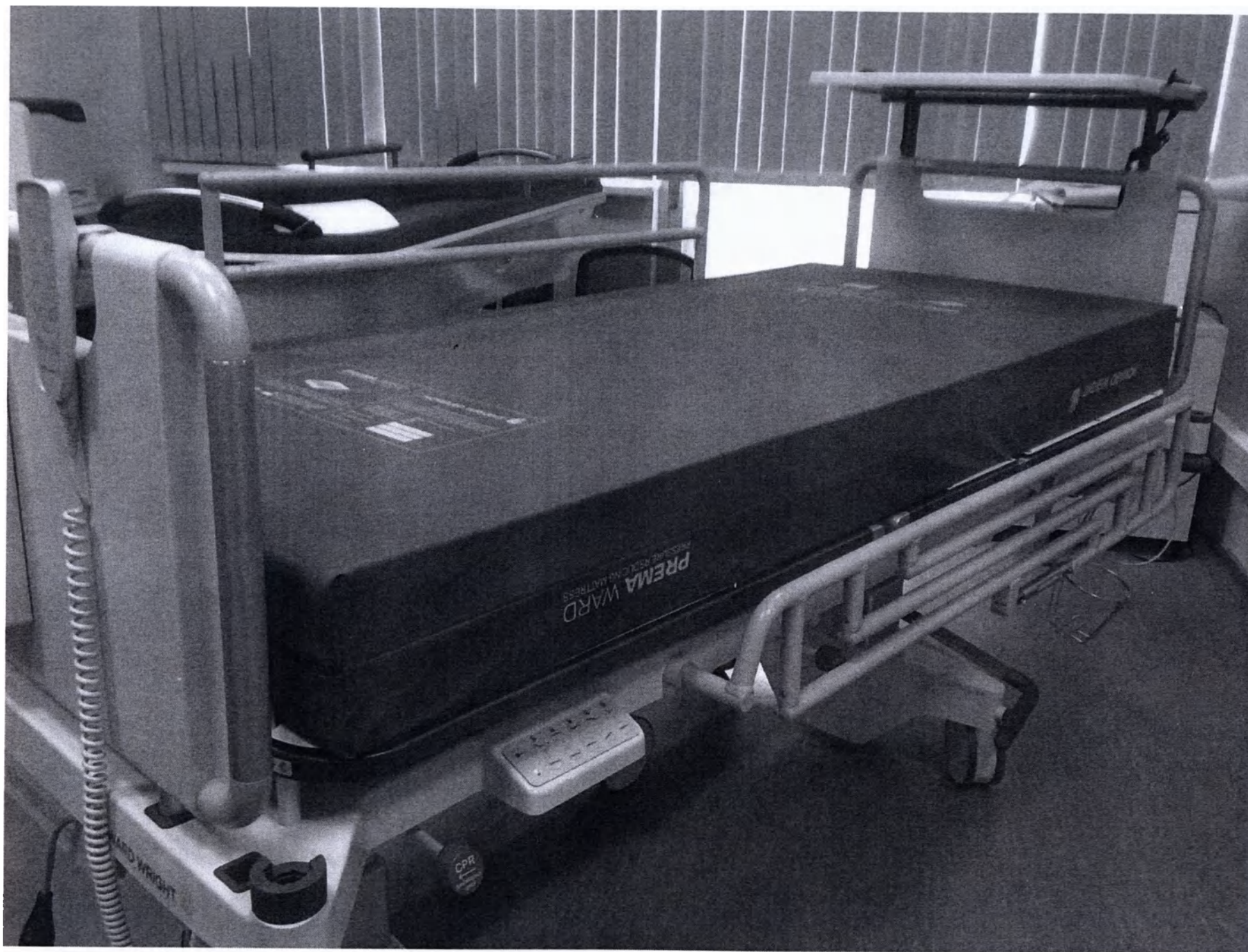
Рис. 1 Кровать медицинская функциональная для интенсивной терапии М8 в вариантах исполнения с принадлежностями, вариант исполнения: Кровать для интенсивной терапии М8 с горизонтальными боковыми ограждениями.
