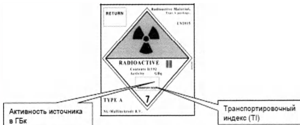
Рис. 5: этикетка категории «II-желтая» для возврата отработанного источника
