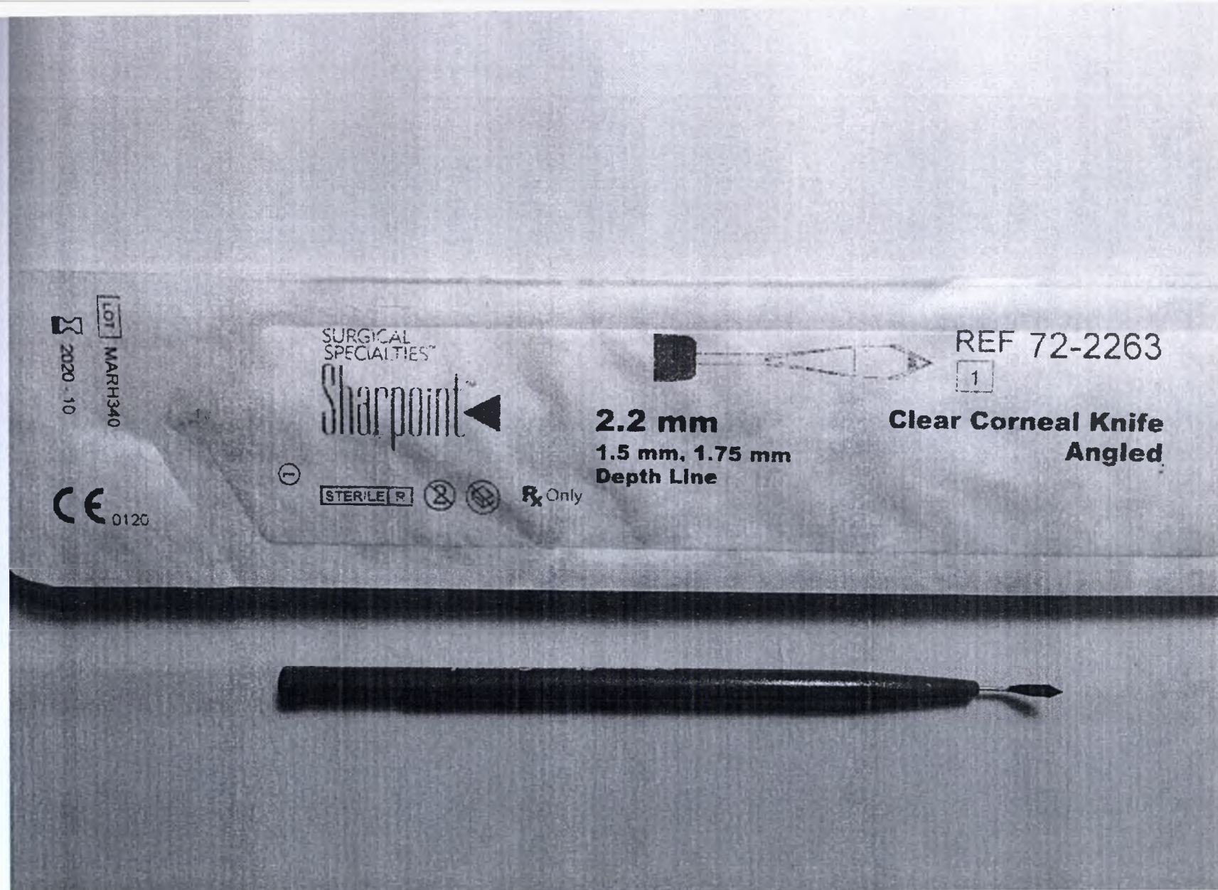
Нож офтальмологический для роговичного разреза, двойная заточка: 72-2263, под углом 40°, ширина лезвия 2,2 мм, 1,5мм и 1,75мм индикаторы глубины разреза
