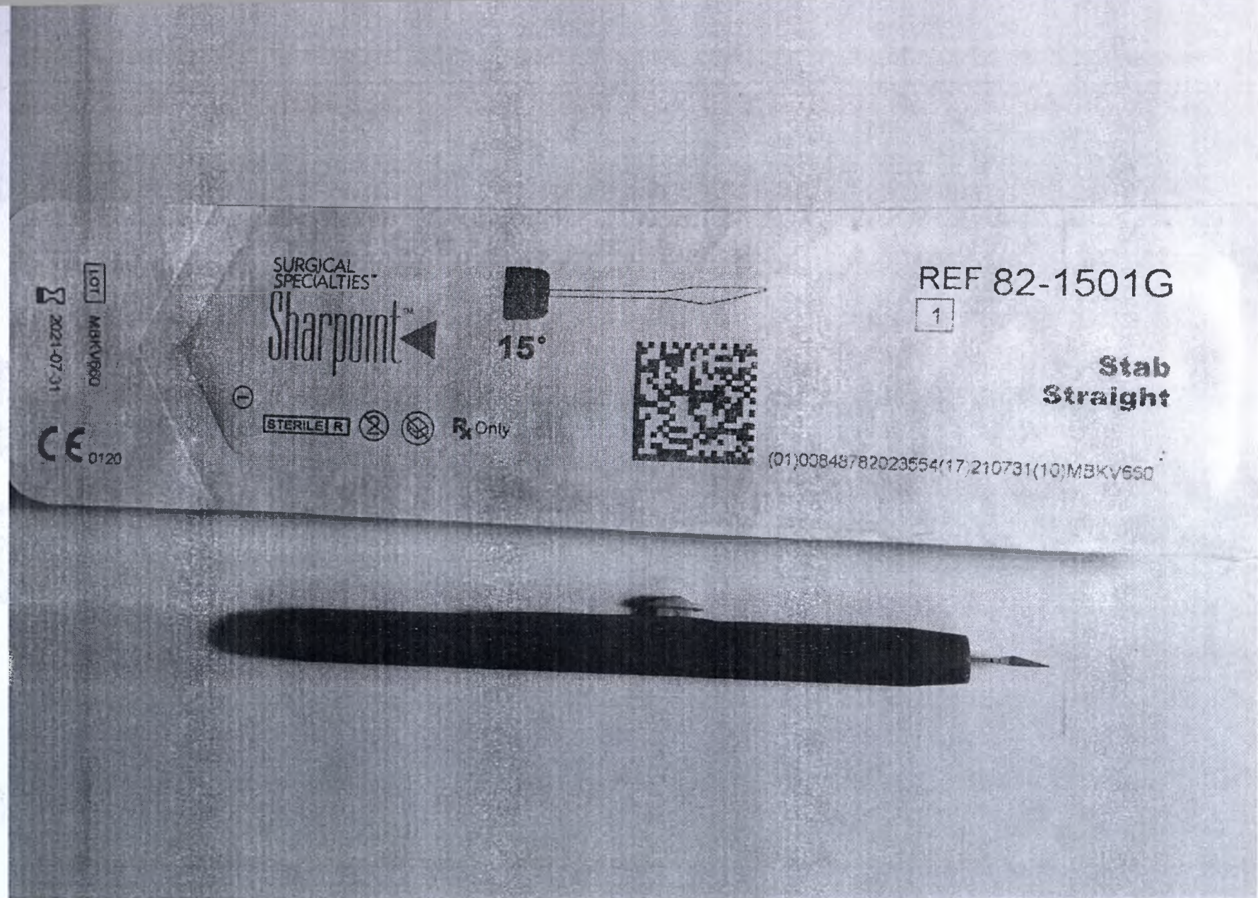
Нож офтальмологический ударный (копьевидный): 82-1501G, прямой, угол заточки 15°, ширина лезвия 1,5 мм, с защитой лезвия
