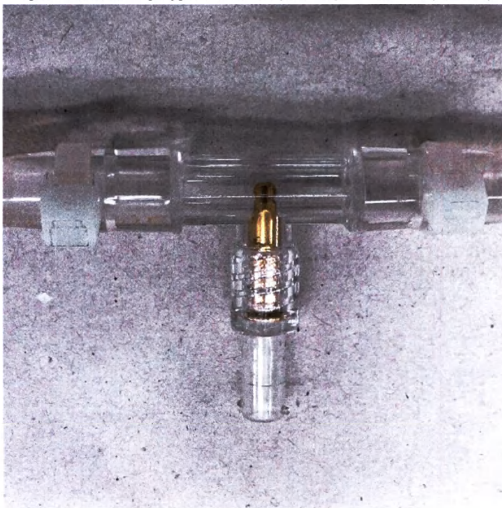
Коннектор датчиков температуры 1/4 дюйма (6,35 мм) - 1/4 дюйма (6,35 мм) - 2 шт.
