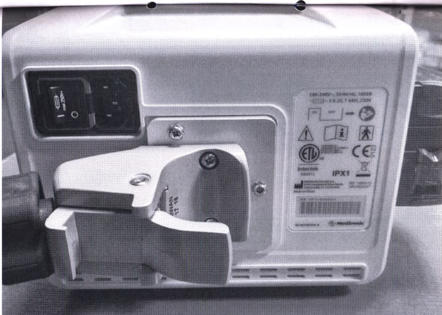
Задняя панель Консоли XPS Nexus
