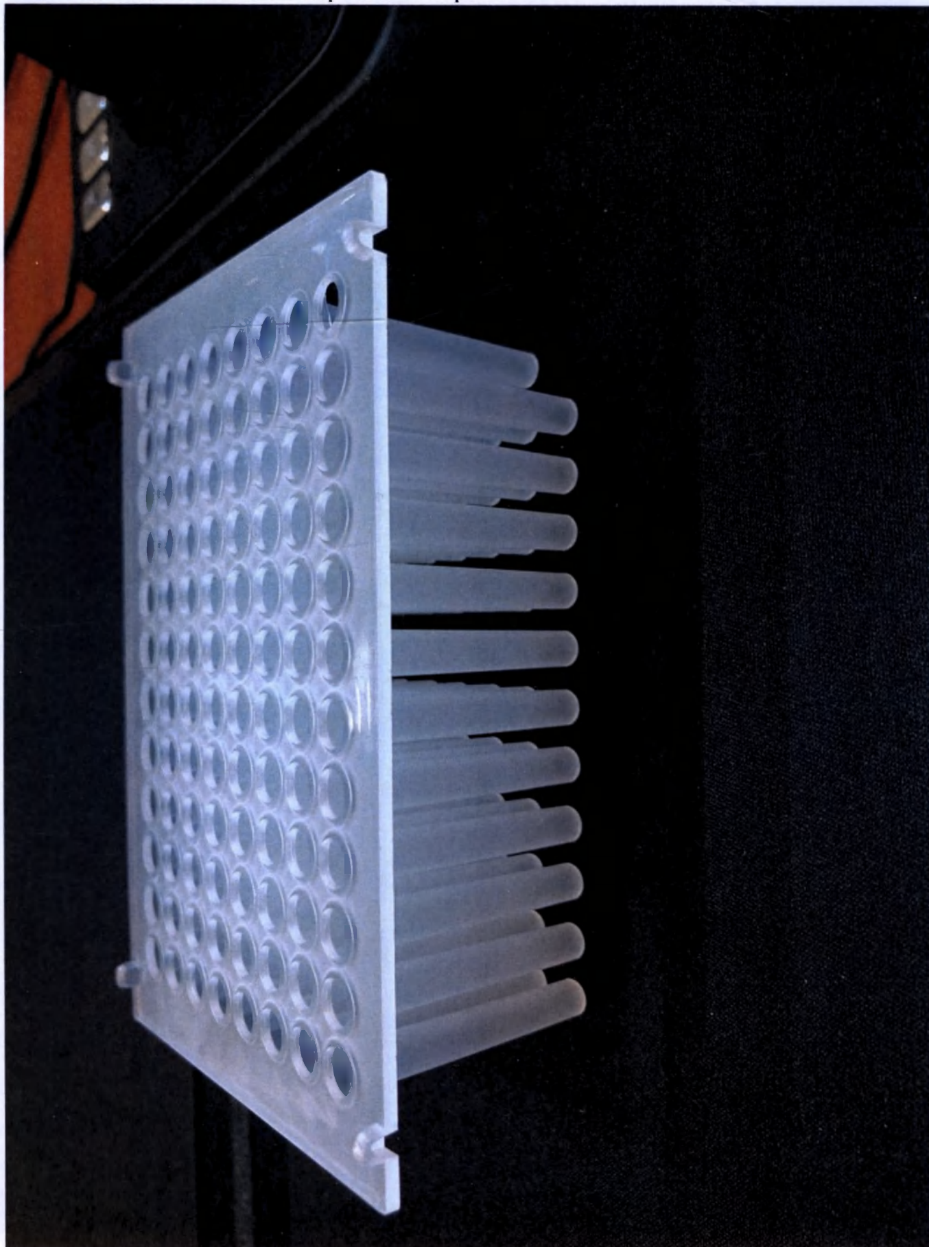
Общий вид насадки на магнитные стержни на 96 стержней
