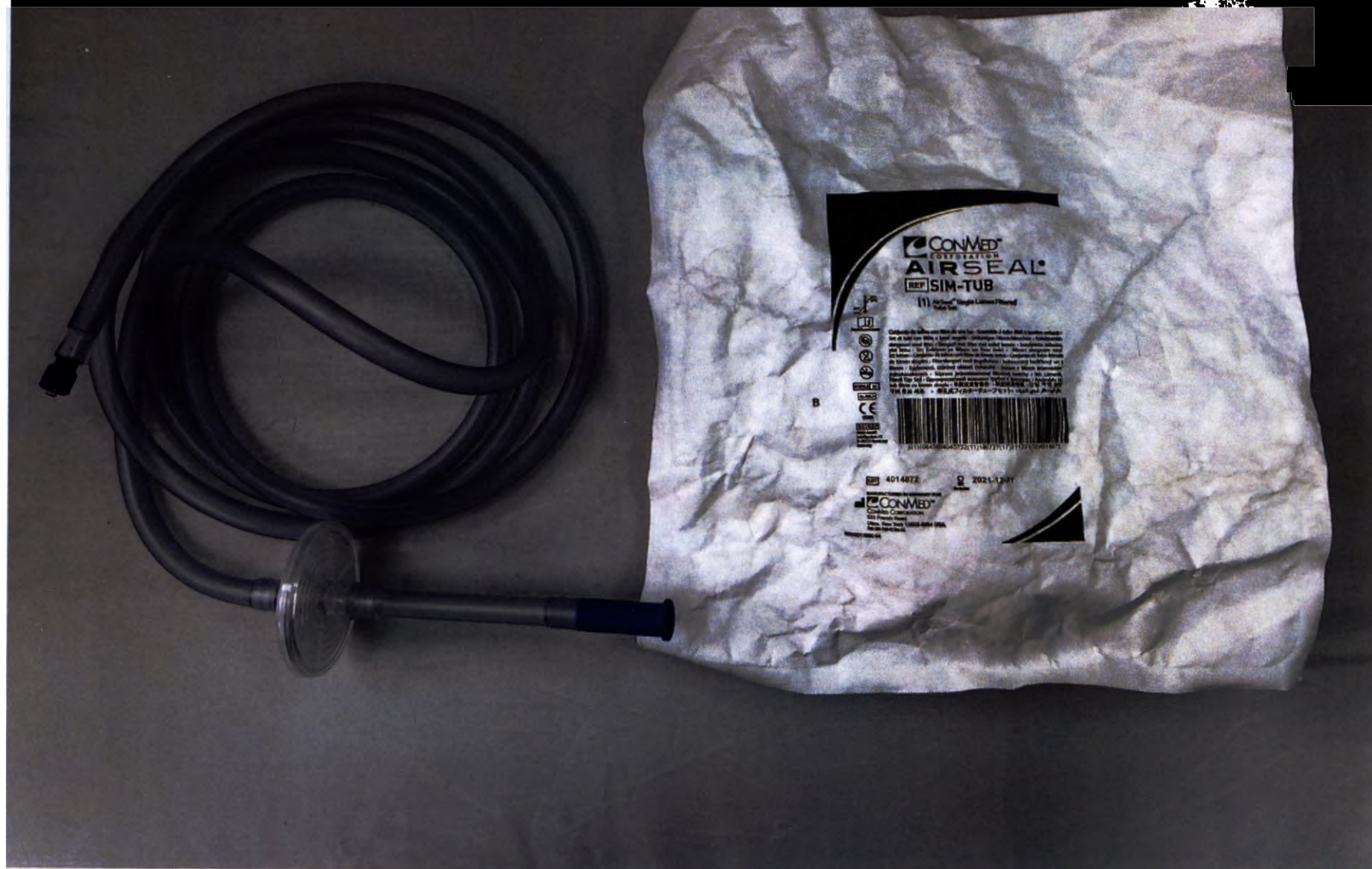
Трубка однопросветная с фильтром для режима стандартной инсuffляции.
