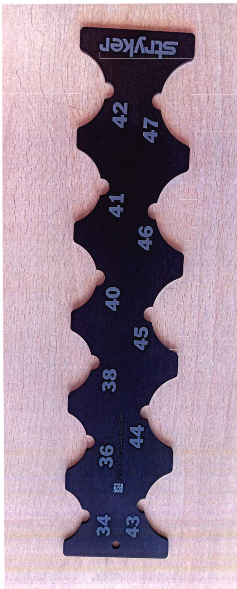
Шаблон для подбора размера централизатора, 34-47 мм
