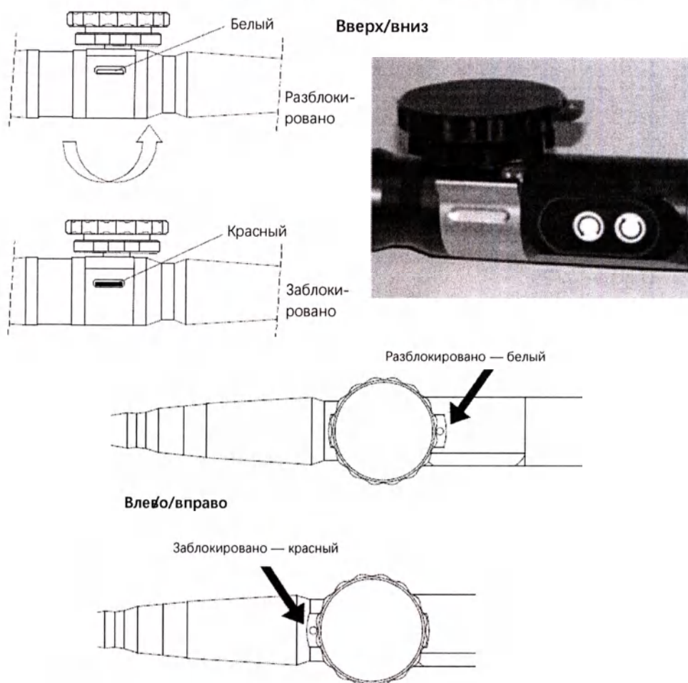
Рис. Н-2. Кнопки для фиксации, датчики Р7-3Тs
