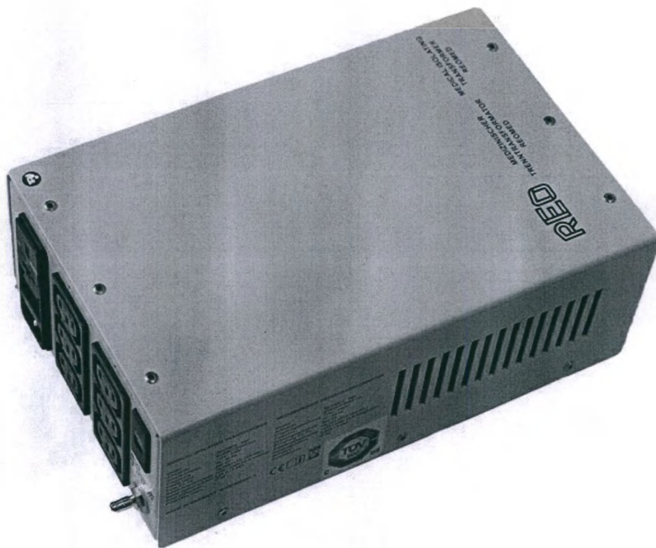
Трансформатор изолирующий медицинского назначения
