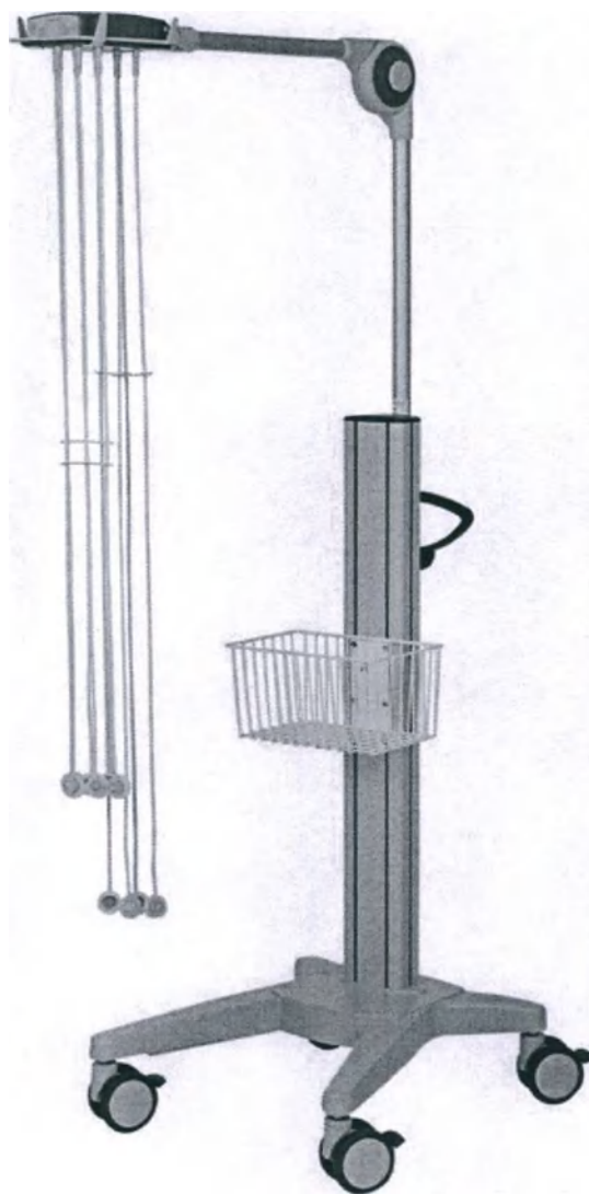
Устройство вакуумной аппликации электродов ЭКГ ergo vac со сменными отведениями, вариант исполнения: ergo vac compact
