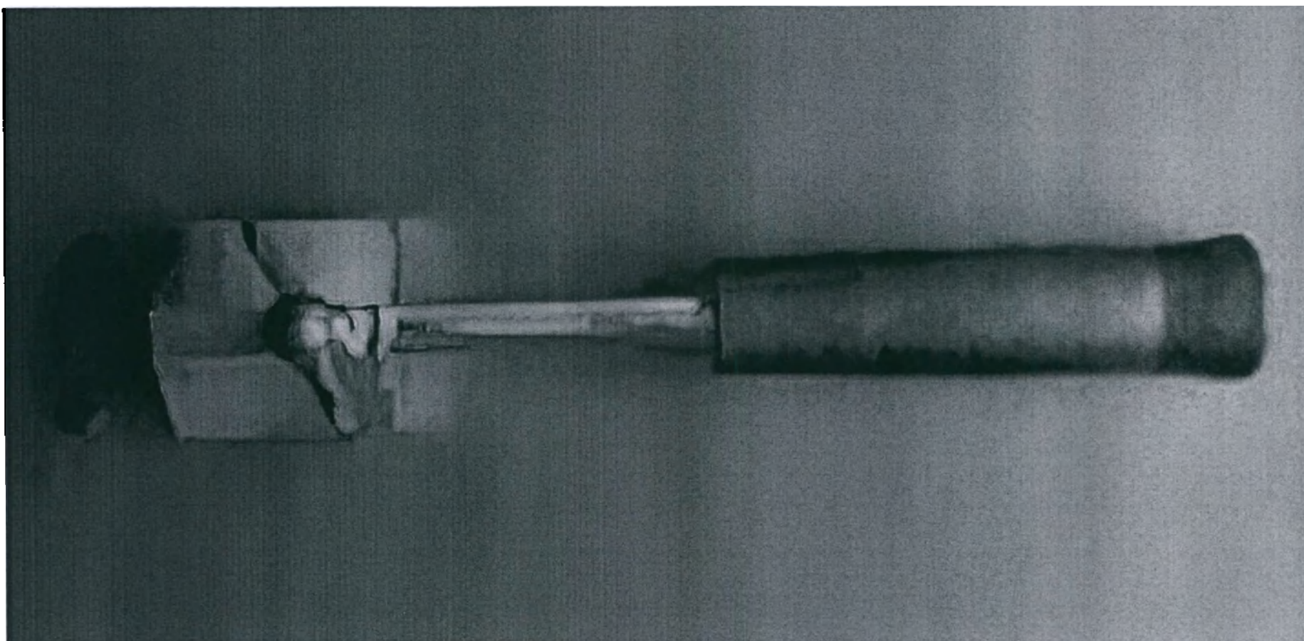
Рукоятка для лежащего велоэргометра, РУ №ФСЗ 2010/06043
