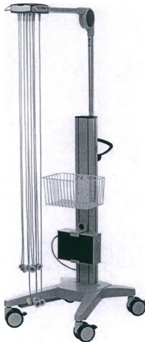
Устройство вакуумной аппликации электродов ЭКГ ergo vac со сменными отведениями, вариант исполнения: ergo vac
