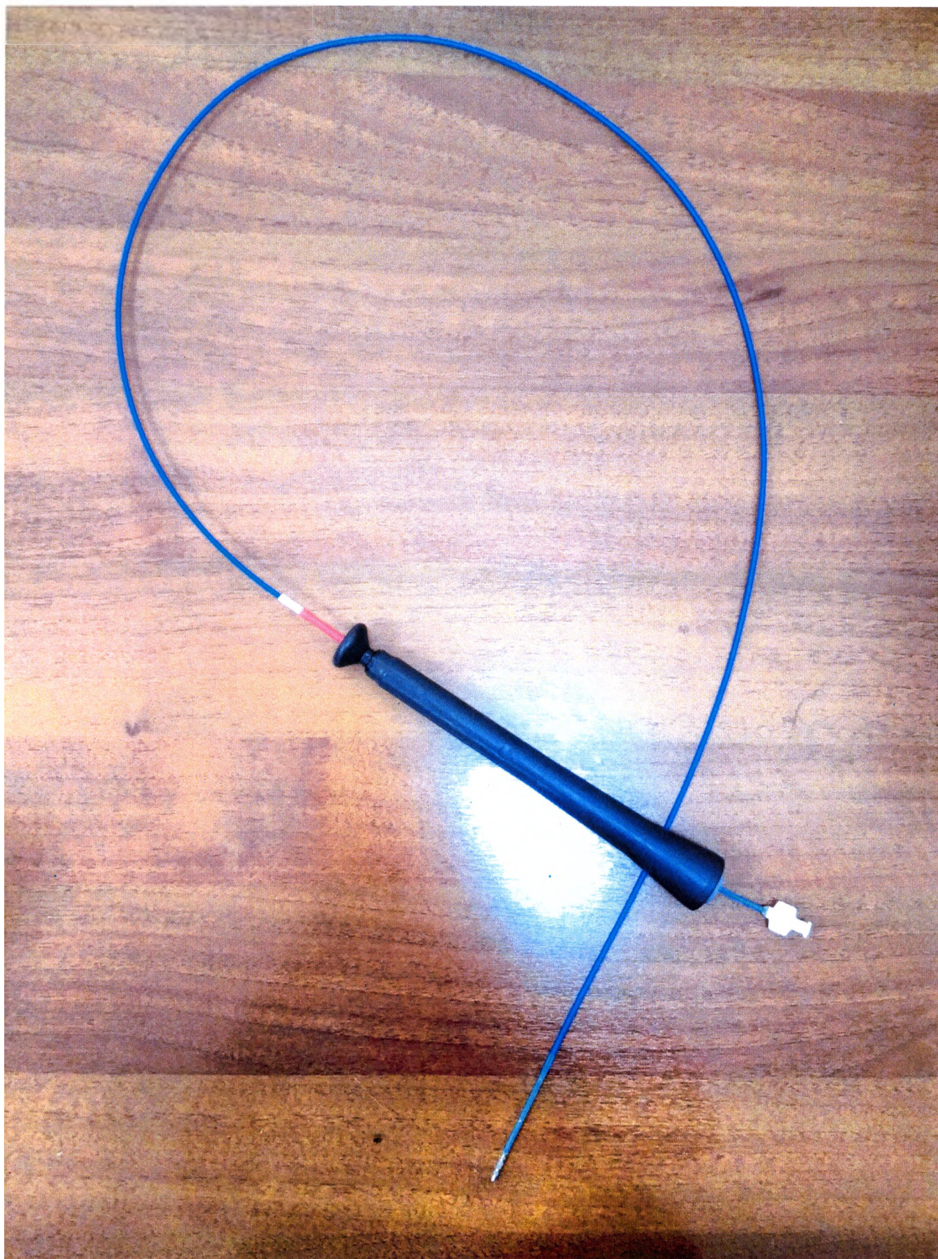
Рисунок 6. Катетер навигационный ThermoCool для радиочастотной абляции сердца (вариант исполнения Катетер однонаправленный ThermoCool SMARTTOUCH SF )
