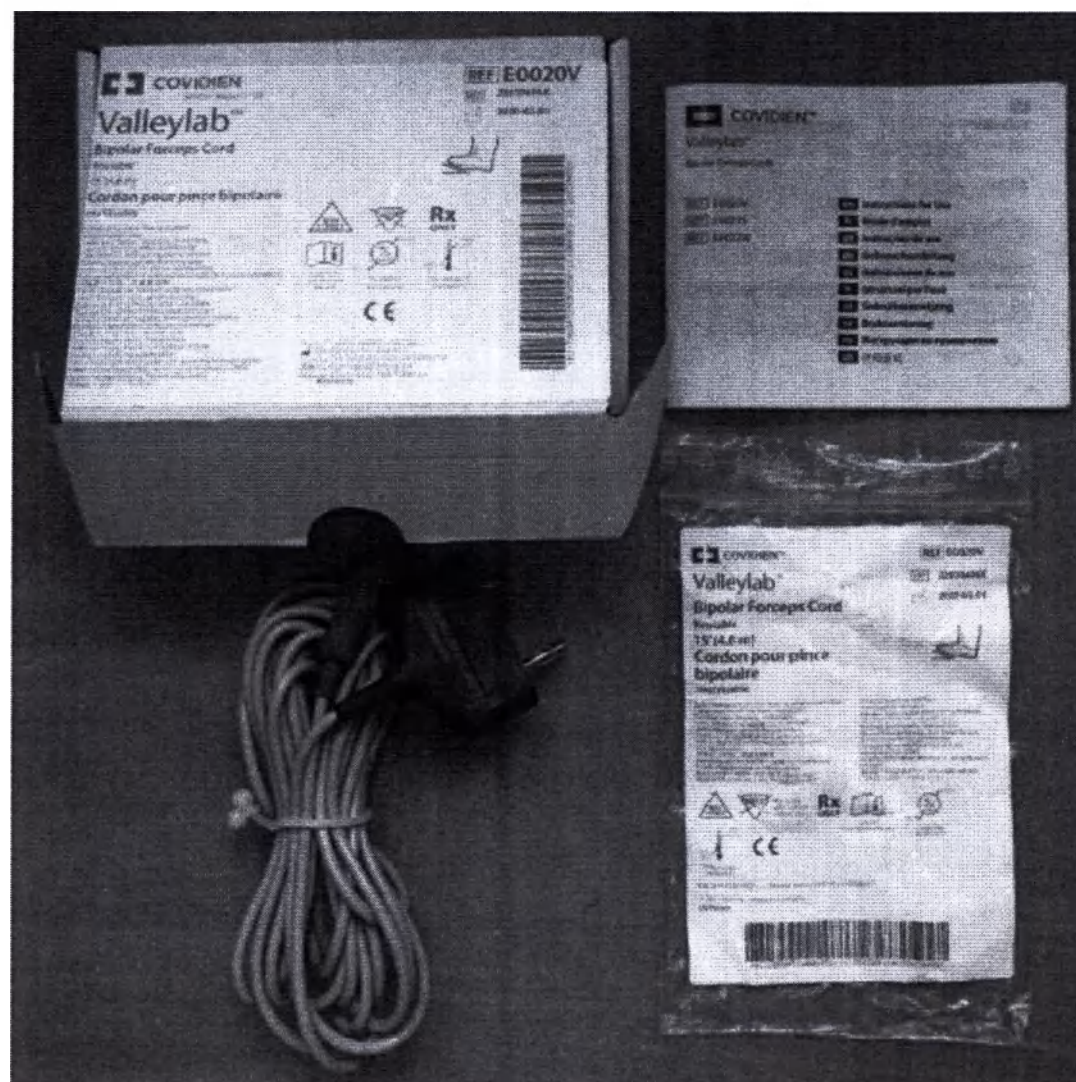
Рис. 14 Упаковка Кабеля биполярного пинцета Valleylab, многоразового использования, представлена на примере Кабеля биполярного пинцета Valleylab 15' (4,6 м), многоразового использования
